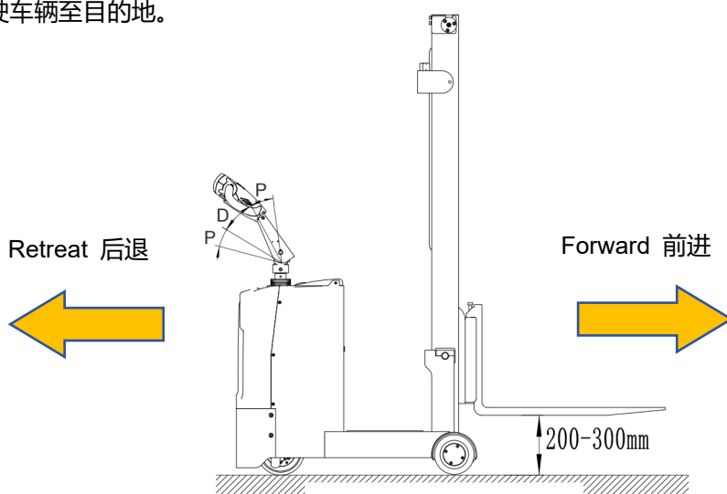
图 8-1 行驶示意图
