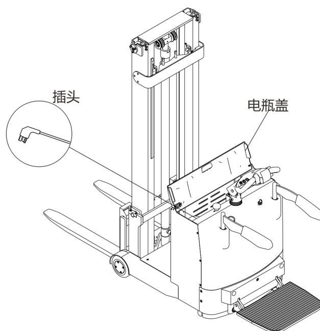
图 10-2 充电示意图
