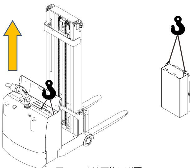
图 10-1 电池更换示意图
