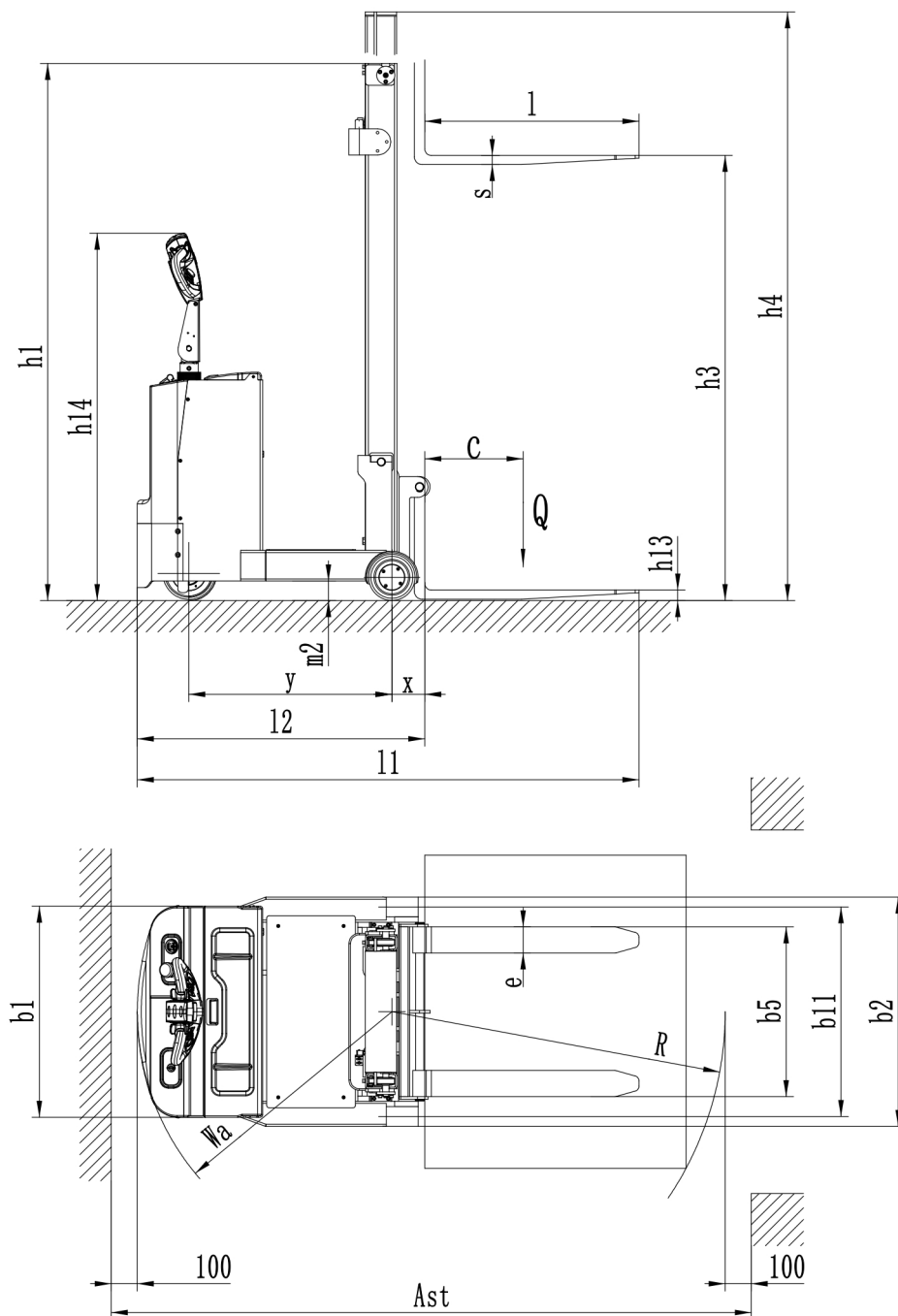
图 3-2 技术参数图
