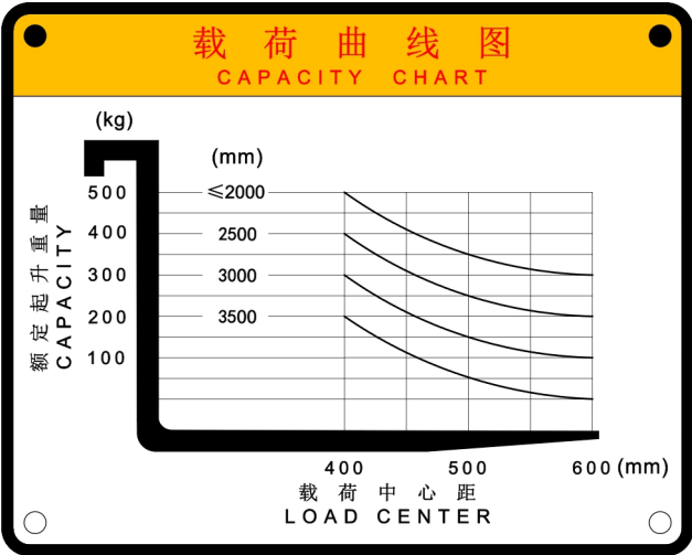
图 3-5 载荷曲线示意图 0.5t
