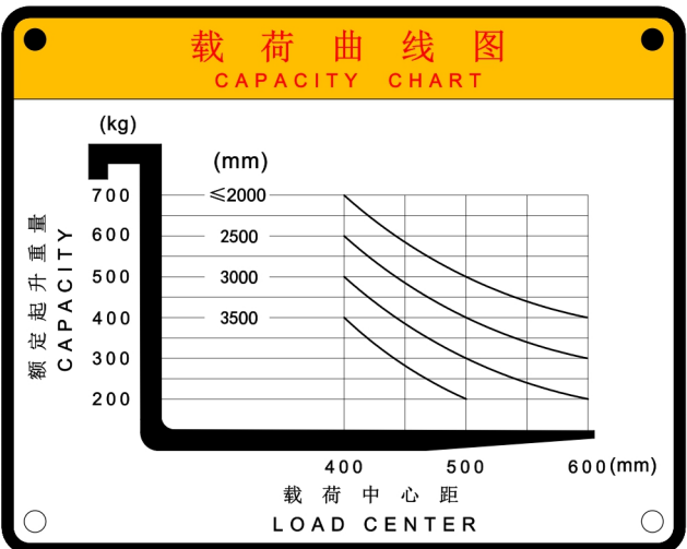
图 3-6 载荷曲线示意图 0.7t
