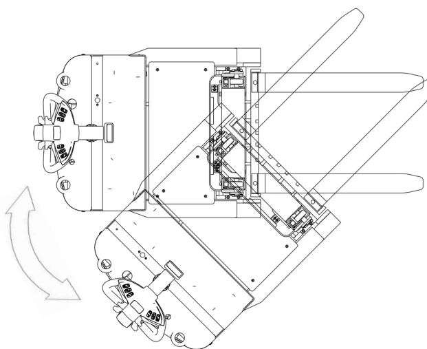
图 8-2 转弯轨迹示意图
