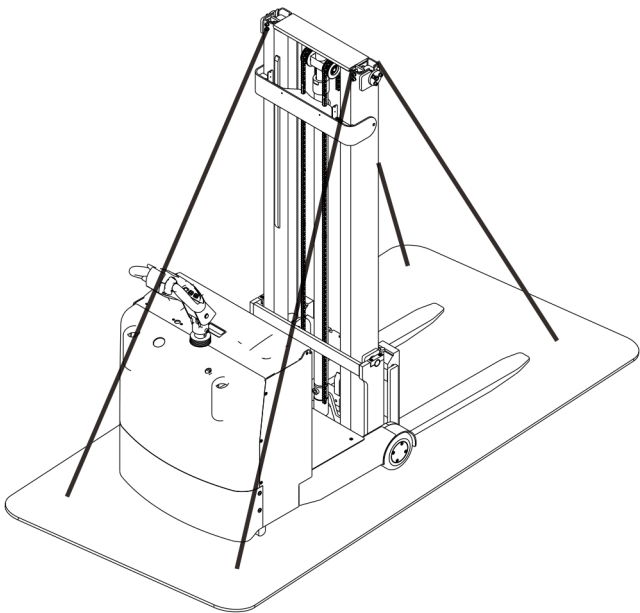
图 5-3 固定点
