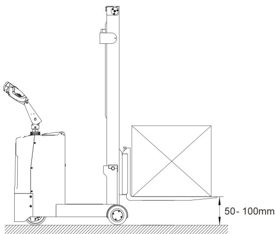
图 9-2 货物提升 50mm—100mm
