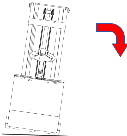
图 8-5 车辆倾覆
