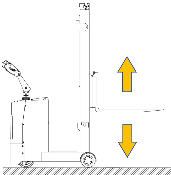
图 8-4 门架主起升
