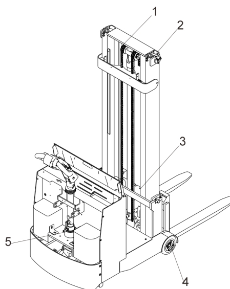
图 13-1 润滑点
