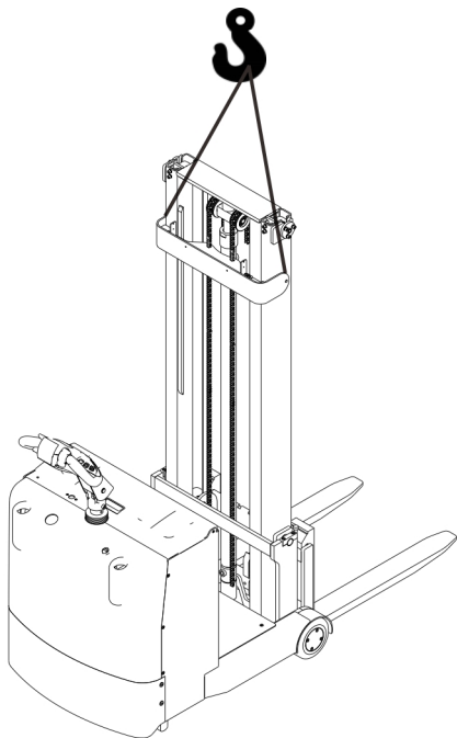
图 5-2 起吊
