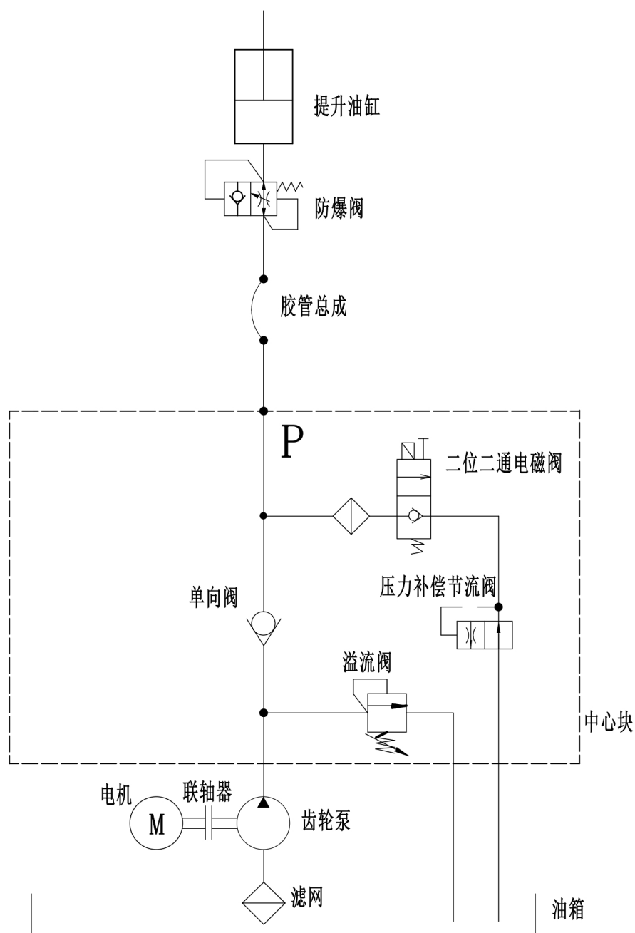
图 16-1 液压原理图
