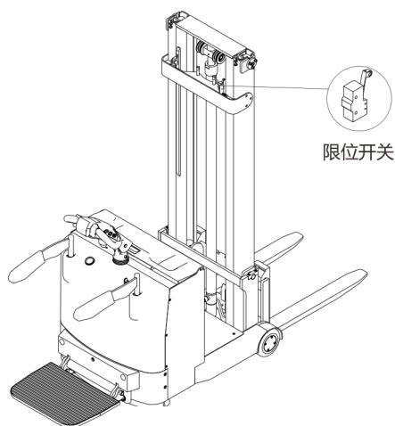
图 8-7 限位开关
