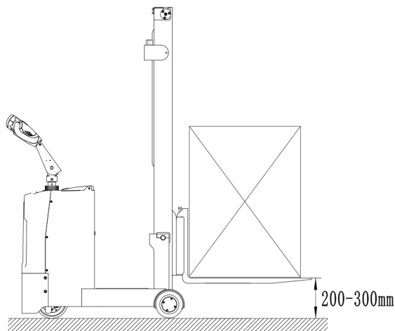
图 9-3 大体积物料
