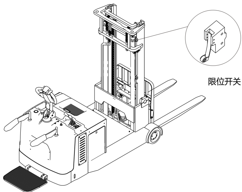
图 8-8 限高示意图
