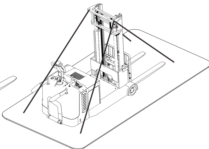
图 5-2 固定点
