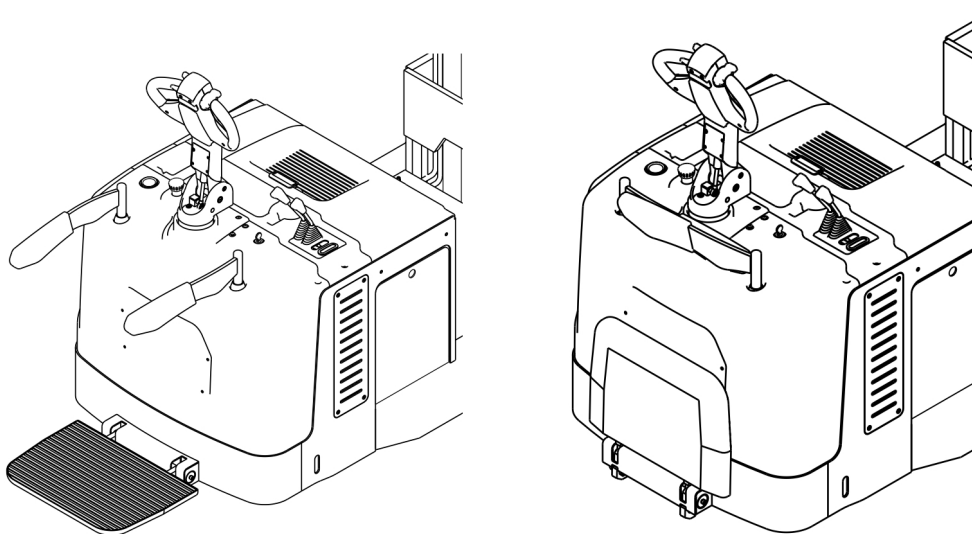
图 8-7 踏板和护臂的两种状态
