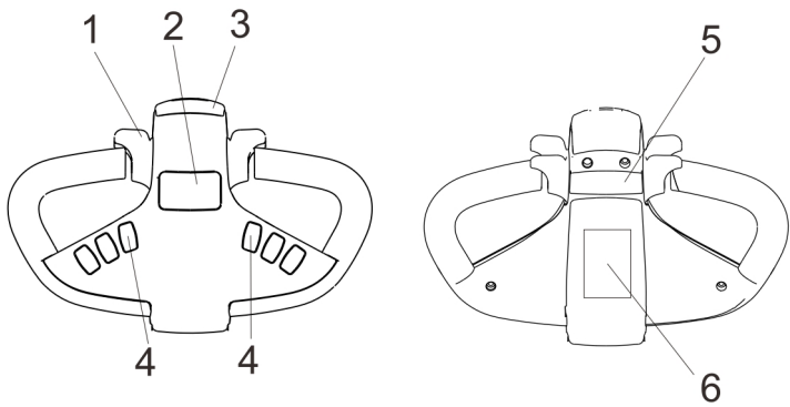
图 7-2 操作手柄
