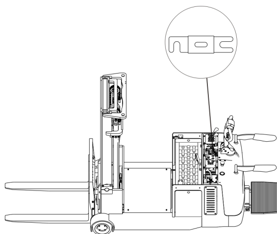
图 13-3 保险丝位置
