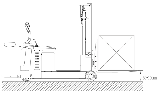
图 9-2 货物提升 50mm—100mm
