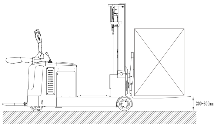
图 9-3 大体积物料 200mm-300mm
