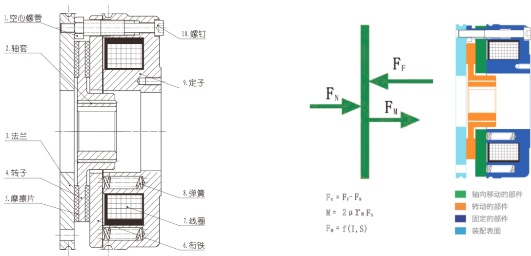
图 8-4 制动原理图
