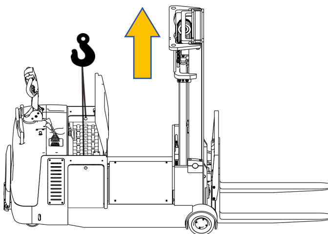
图 10-1 电池更换示意图
