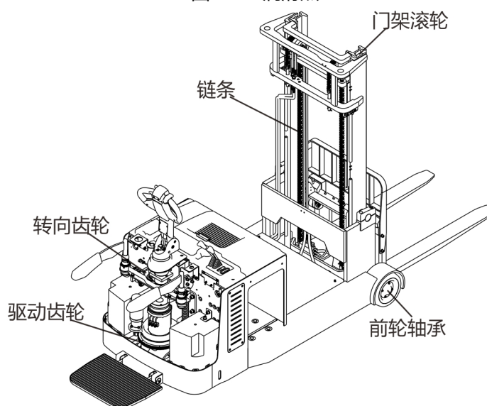
图 13-1 润滑点
