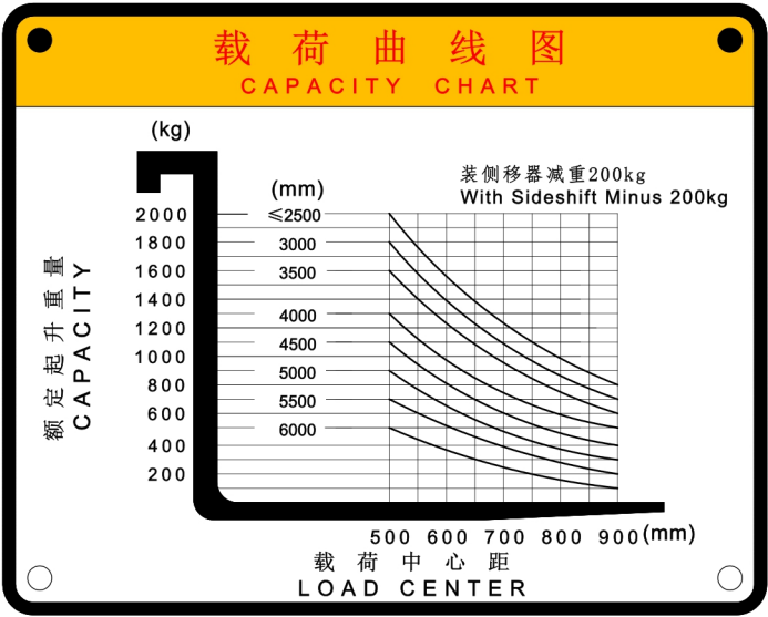
图 3-5 载荷曲线示意图
