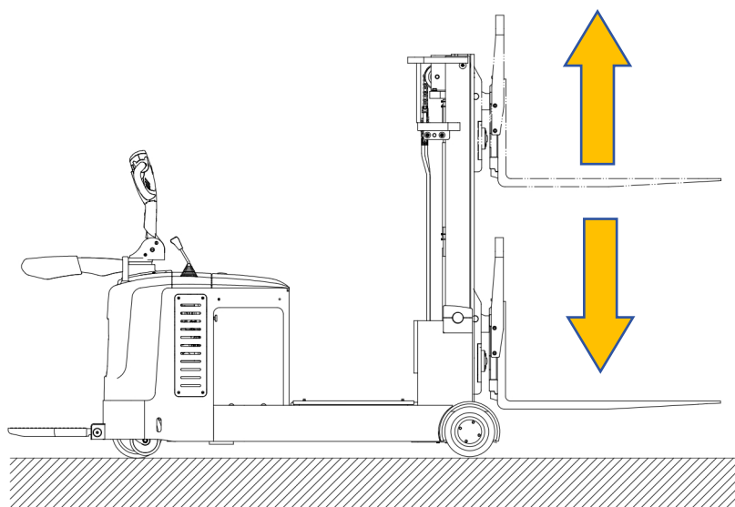
图 8-5 门架主起升
