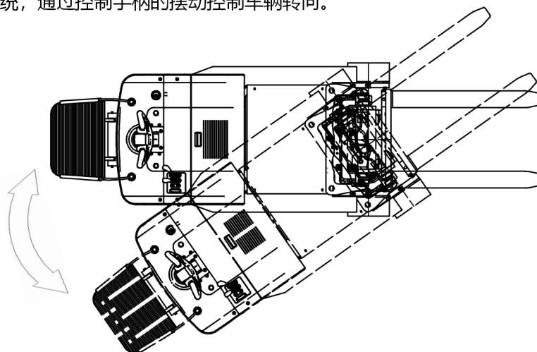
图 8-2 转弯轨迹示意图
