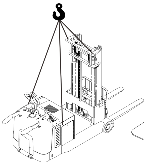
图 5-1 起吊
