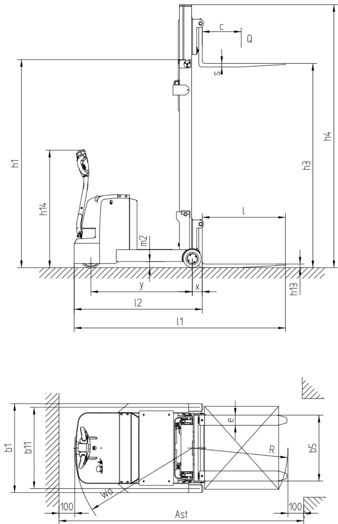
图 3-2 技术参数图
