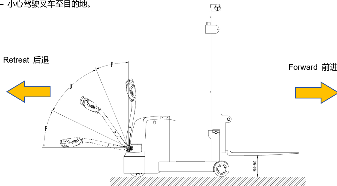
图 8-1 空载行驶示意图
