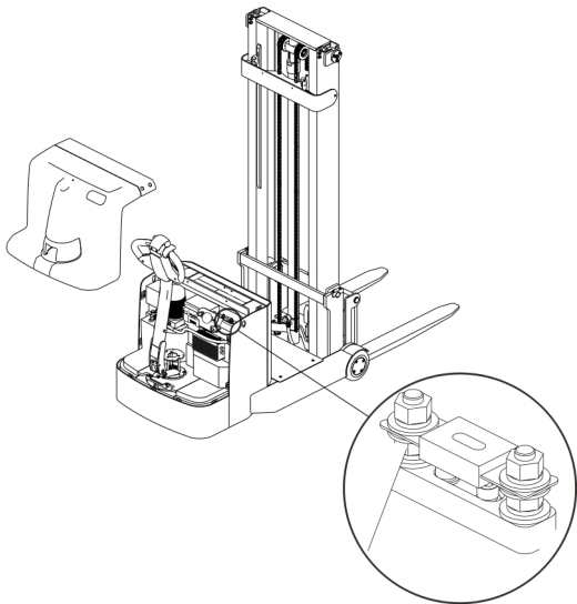
图 12-2 保险丝位
