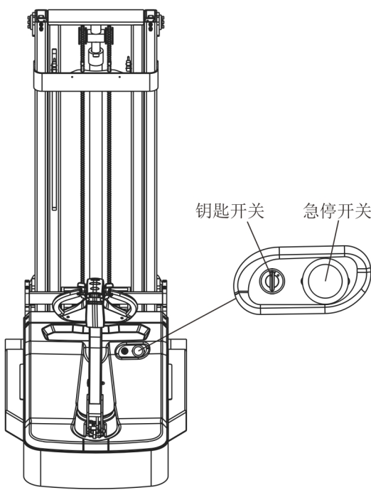
图 7-1 操作控制台
