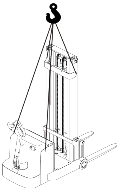
图 5-1 起吊
