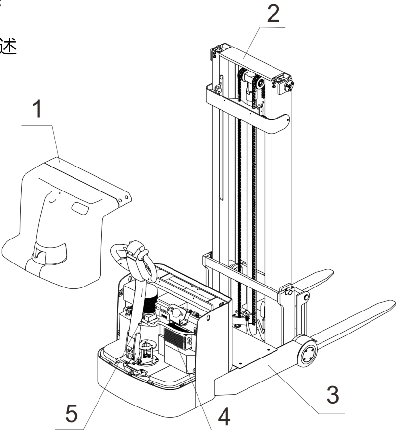
图 3-1 主体分类
