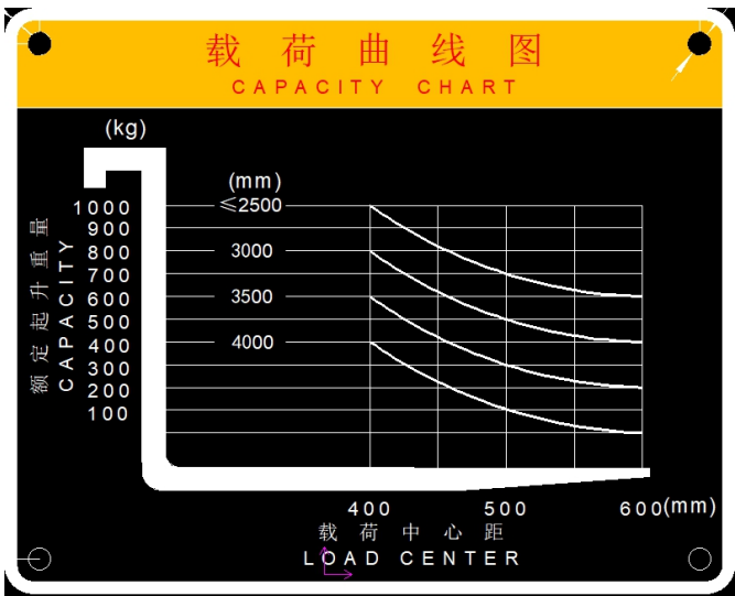
图 3-5 载荷曲线示意图
