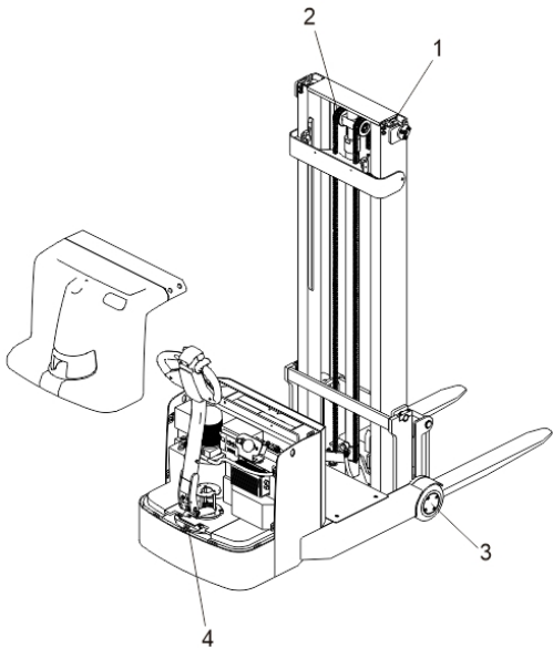
图 12-1 润滑点
