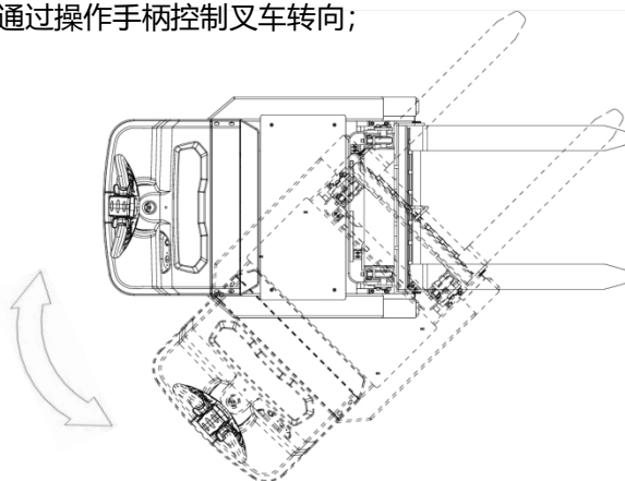
图 8-2 转弯轨迹示意图
