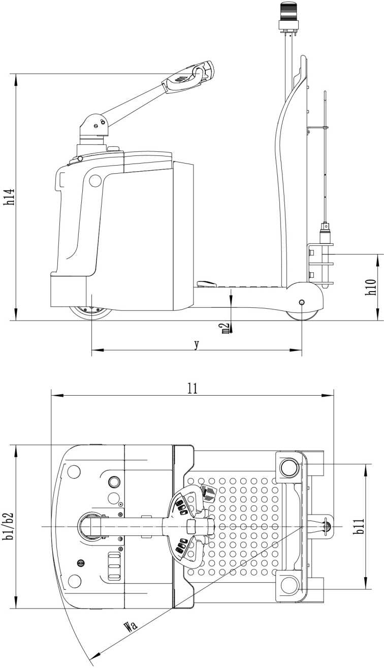
图 3 技术参数图
