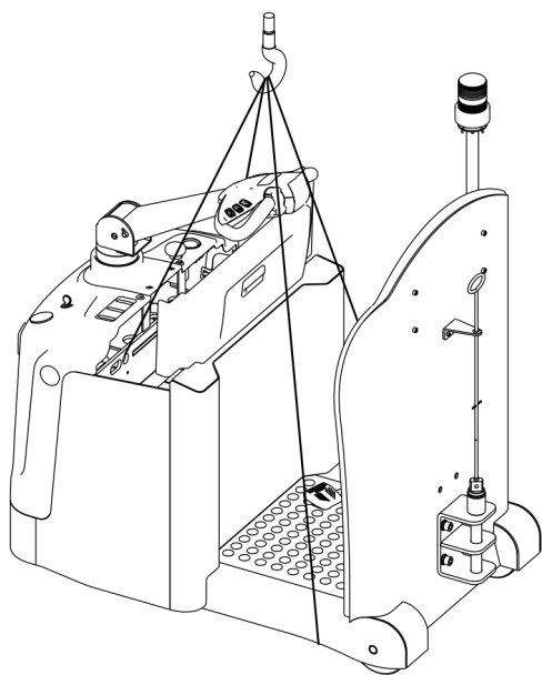
图 6 起吊
