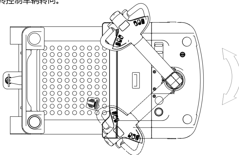
图 12 转向示意图
