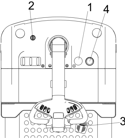
图 8 操作控制台
