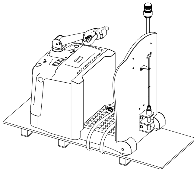
图 7 固定点
