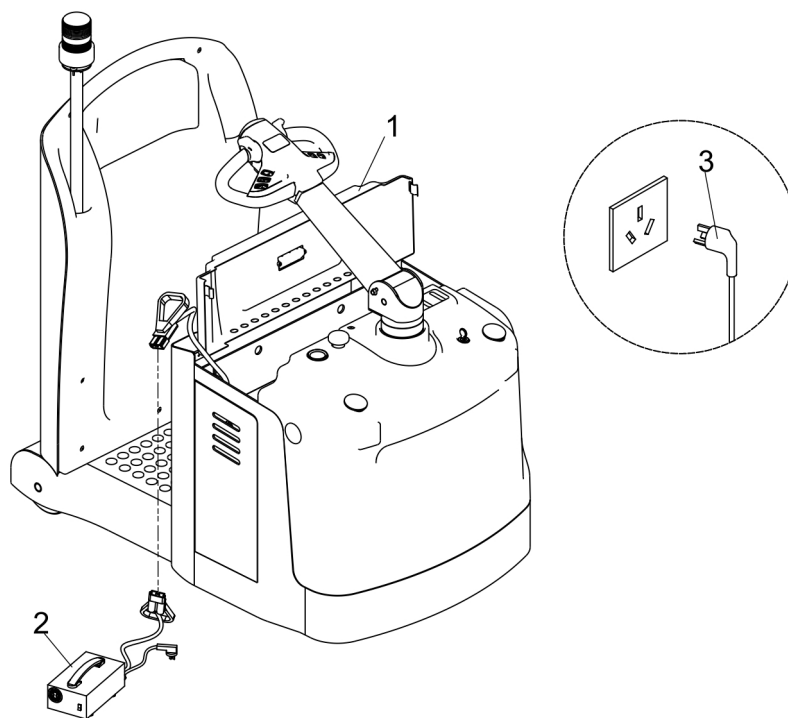
图 22 充电口位置示意图
