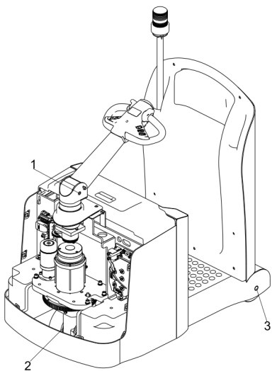
图 24 润滑点
