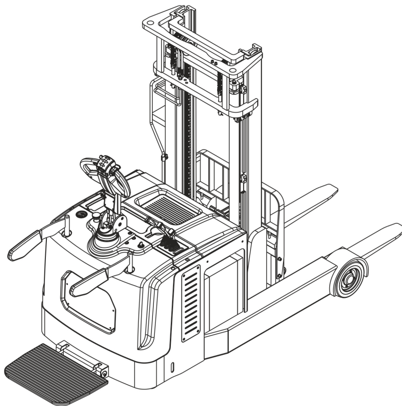
图 1 Q20GA 电动前移式叉车
