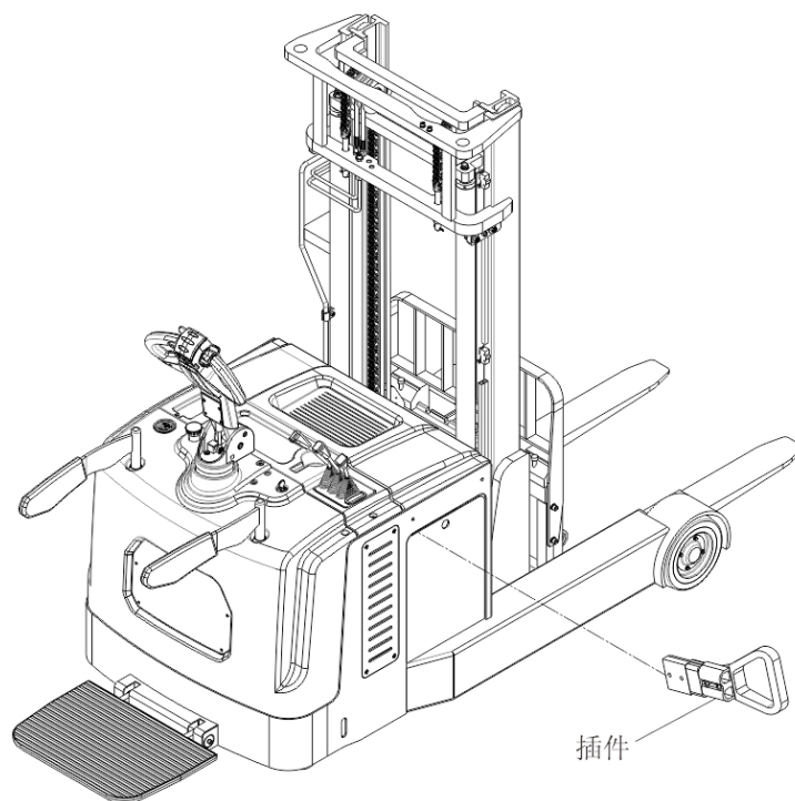
图 26 充电口位置示意图
