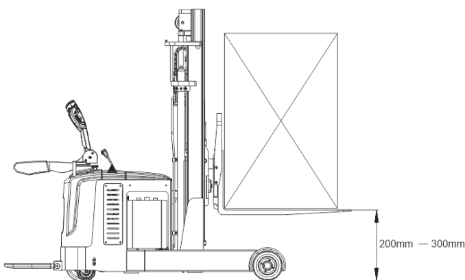
图 25 大体积物料
