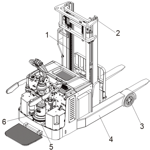
图 29 润滑点
