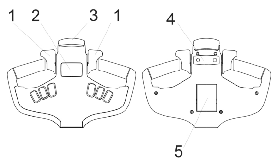
图 11 操作手柄——刷卡器
