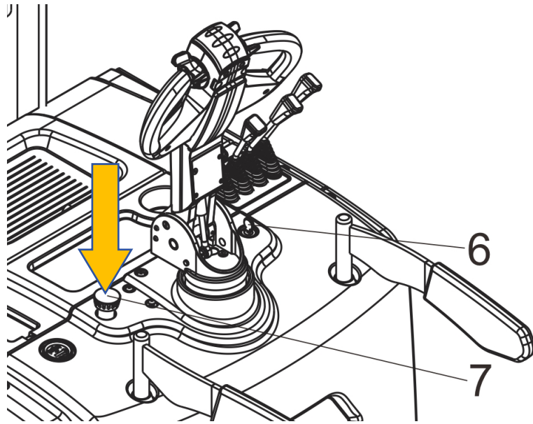
图 17 停车
