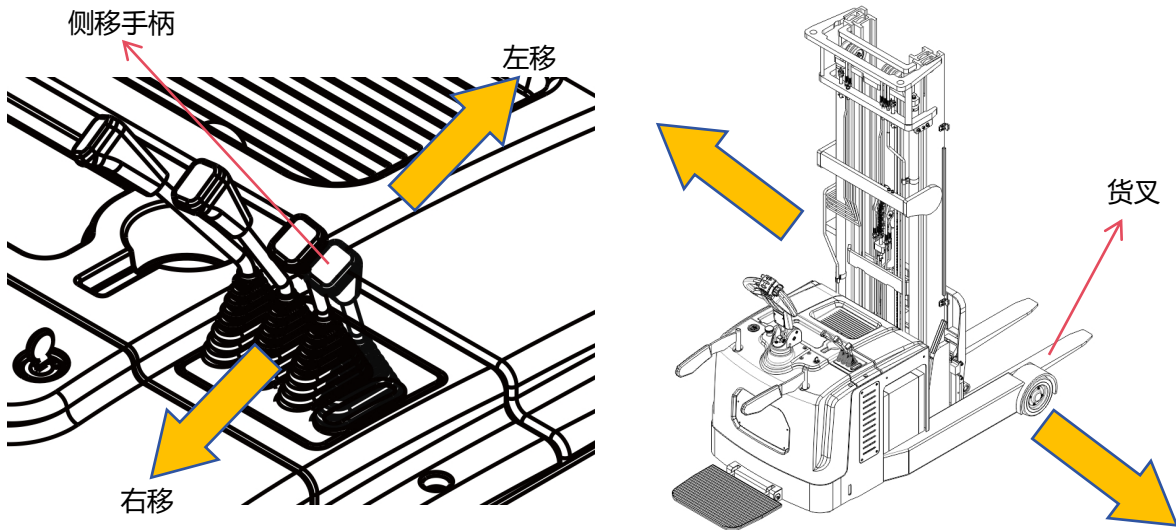
图 21 货叉侧移示意图
