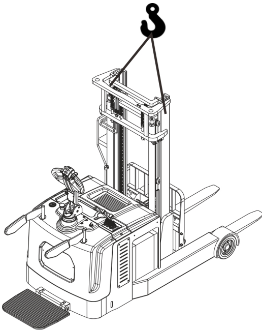
图 7 起吊
