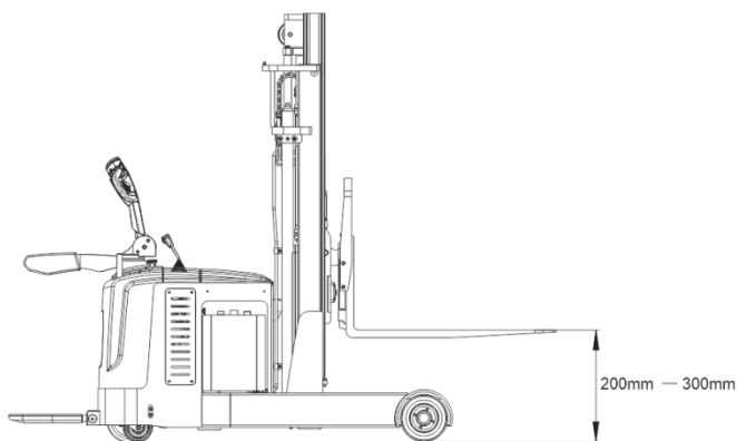
图 23 货叉离地 200mm-300mm
