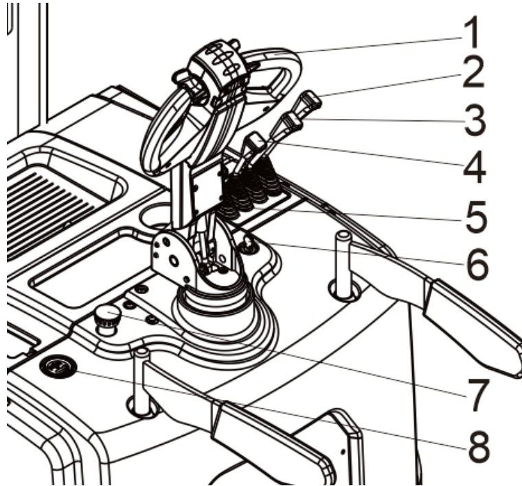
图 9 操作控制台
