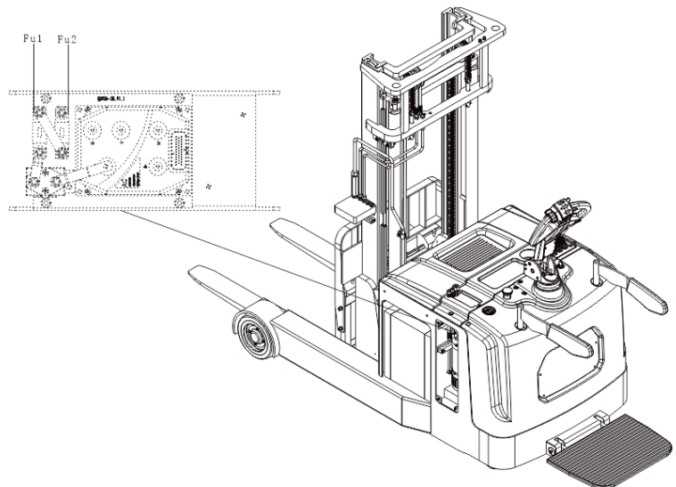
图 30 保险丝位置
