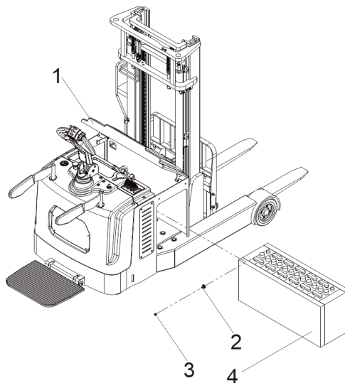
图 26 电池更换示意图
