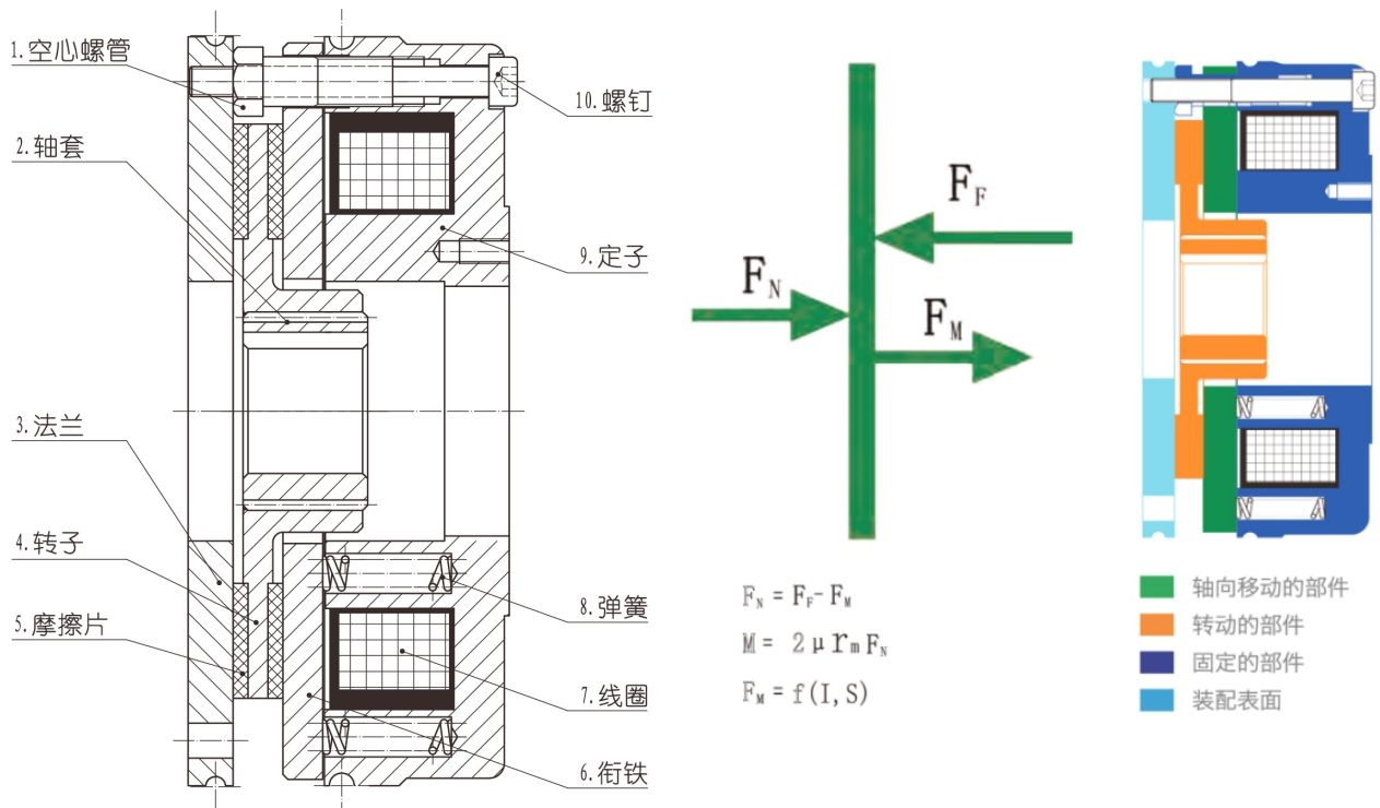
图 16 制动原理图
