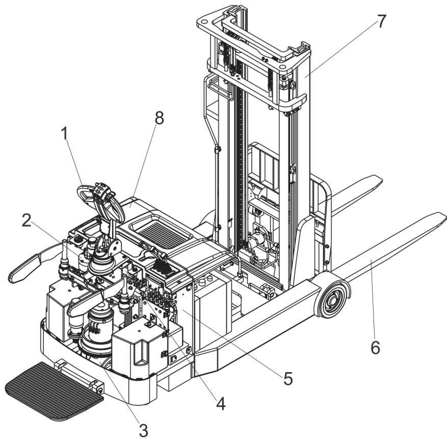
图 2 主体分类
