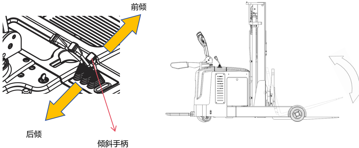
图 20 货叉前后倾斜示意图
