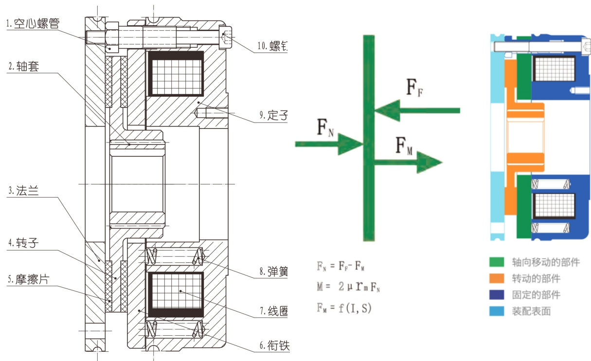
图 20 制动原理图
