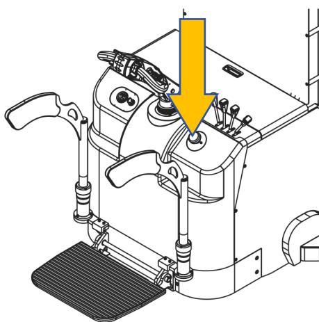
图 21 按下急停开关
