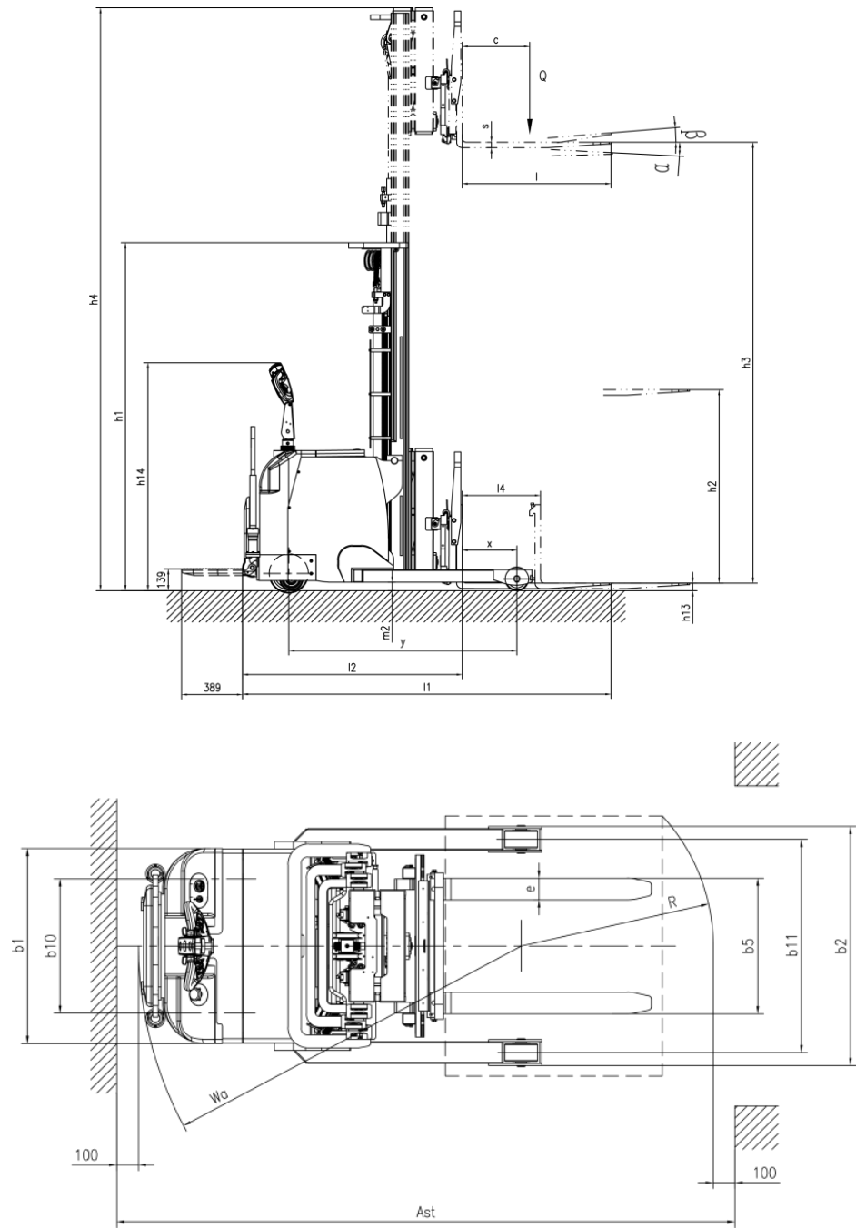
图 3 技术参数图
