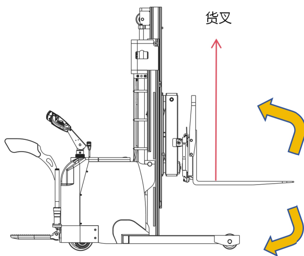
图 24 货叉前后倾斜示意图
