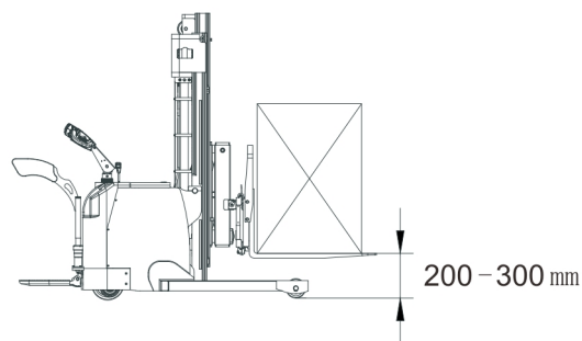
图 28 大体积物料 200-300mm
