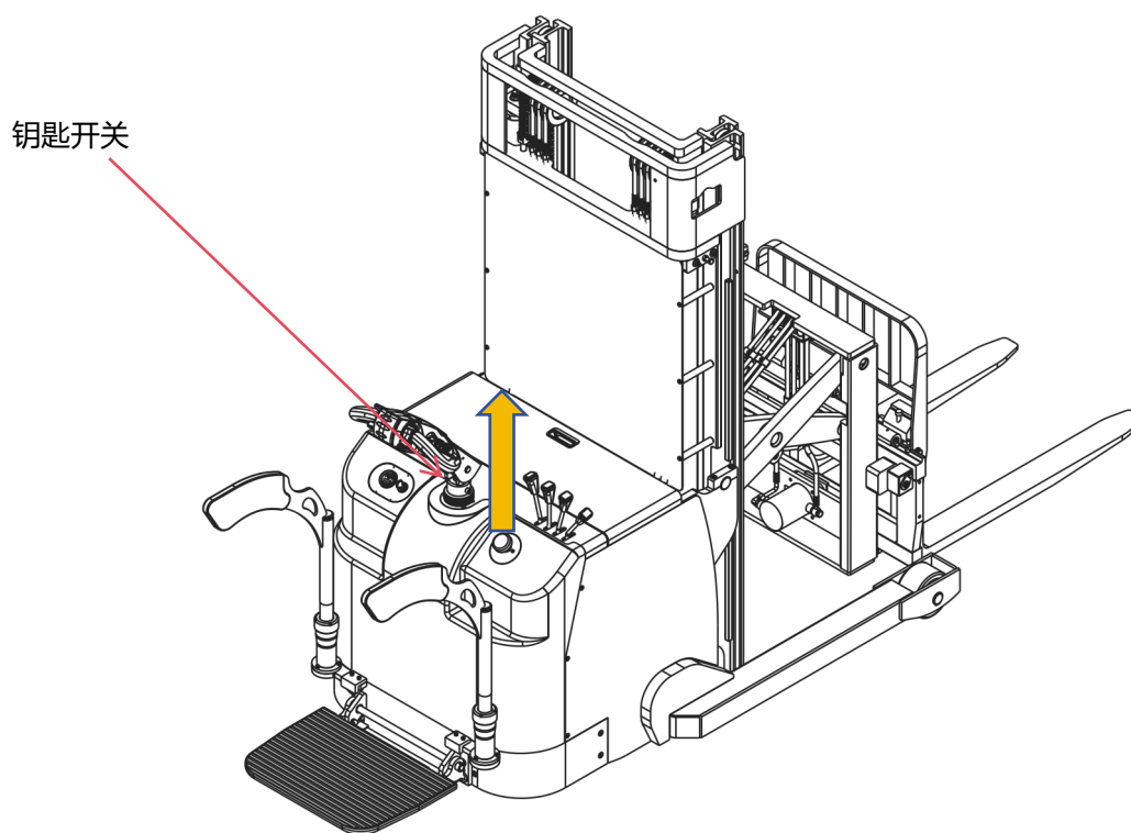
图 15 钥匙开关启动
