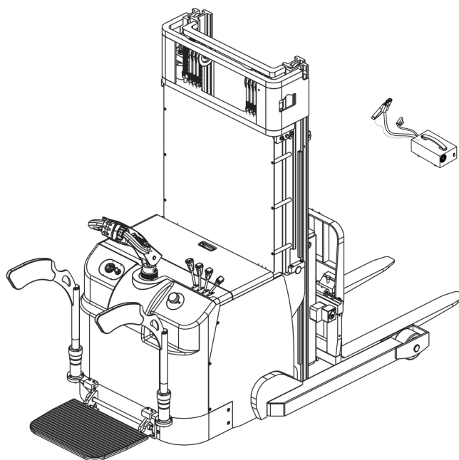
图 30 充电口位置示意图
