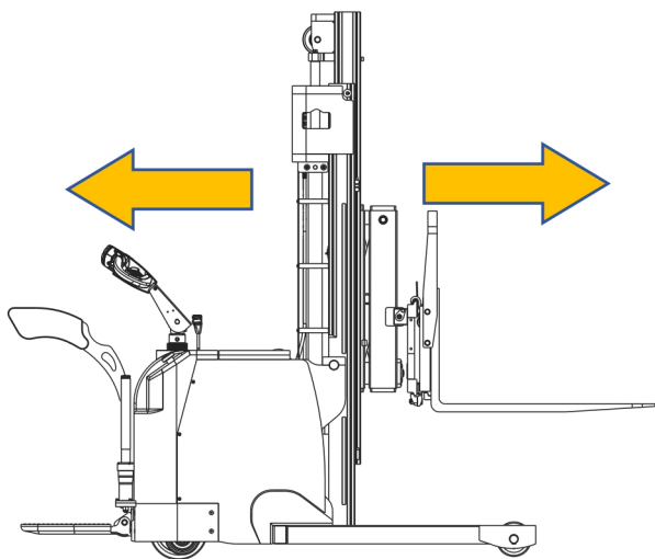
图 23 门架前移后移示意图
