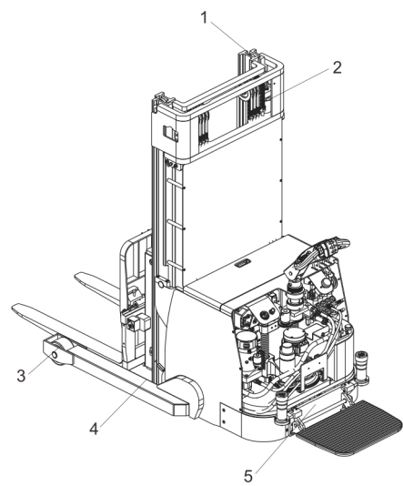
图 33 润滑点
