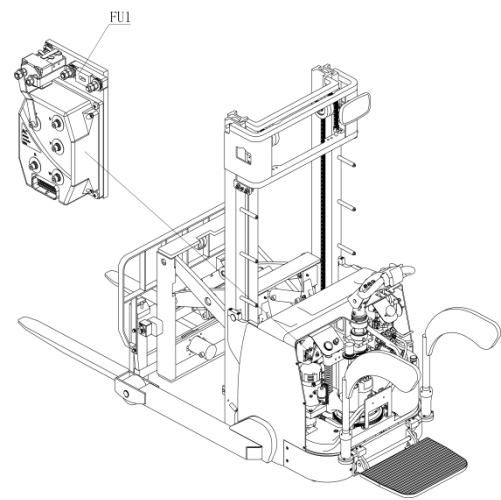
图 34 保险丝位置
