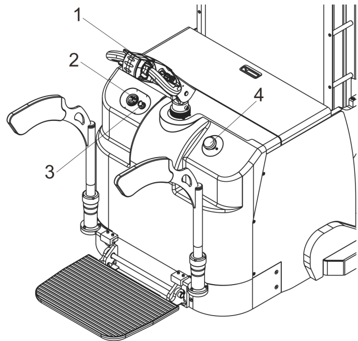
图 12 操作控制台
