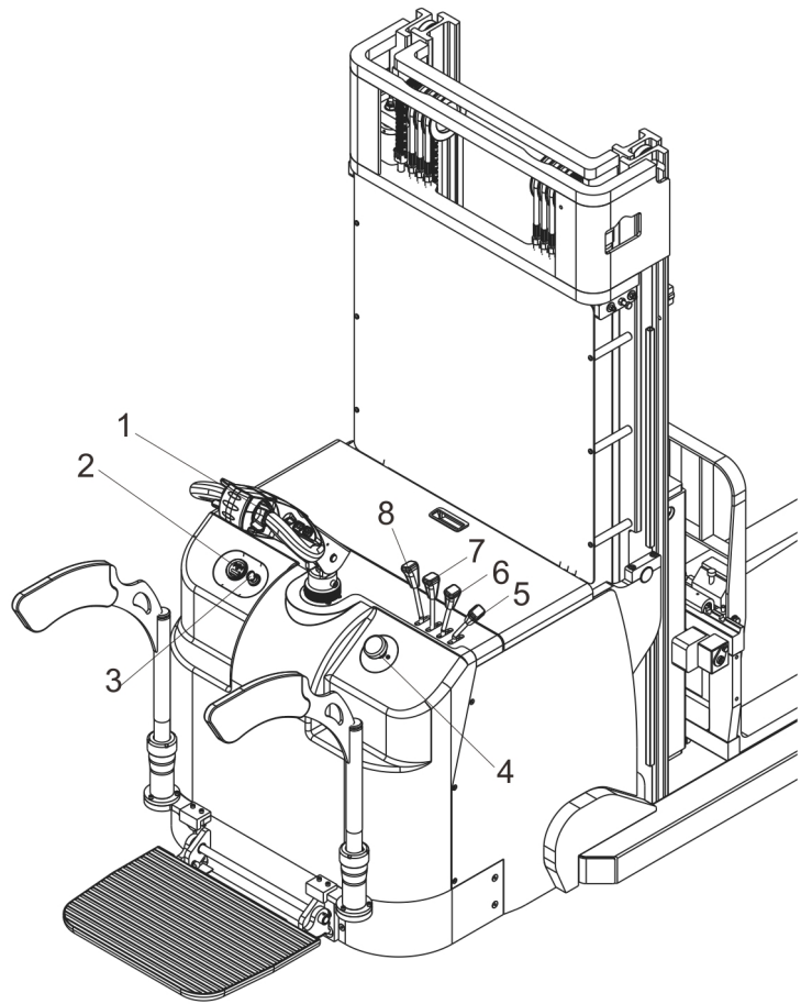
图 9 操作控制台
