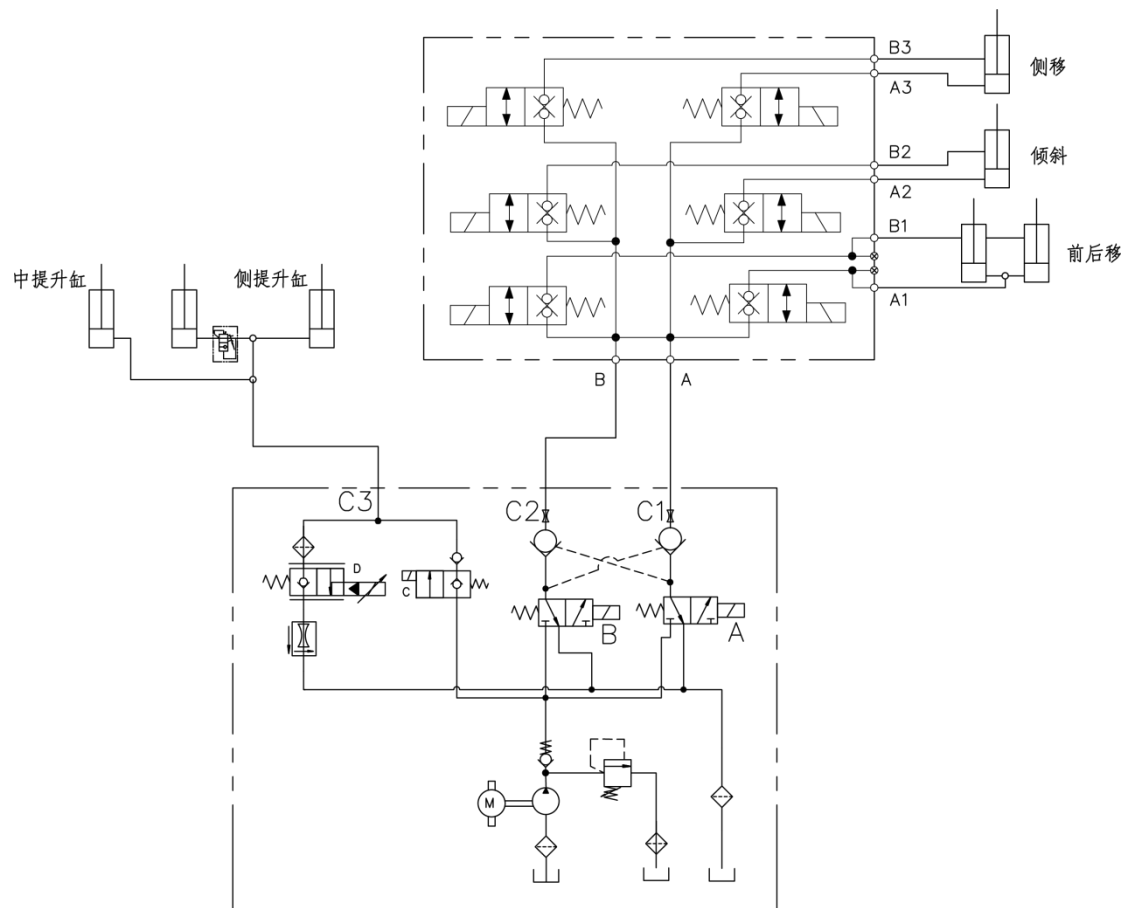
图 38 液压原理图(电磁阀、带侧移)
