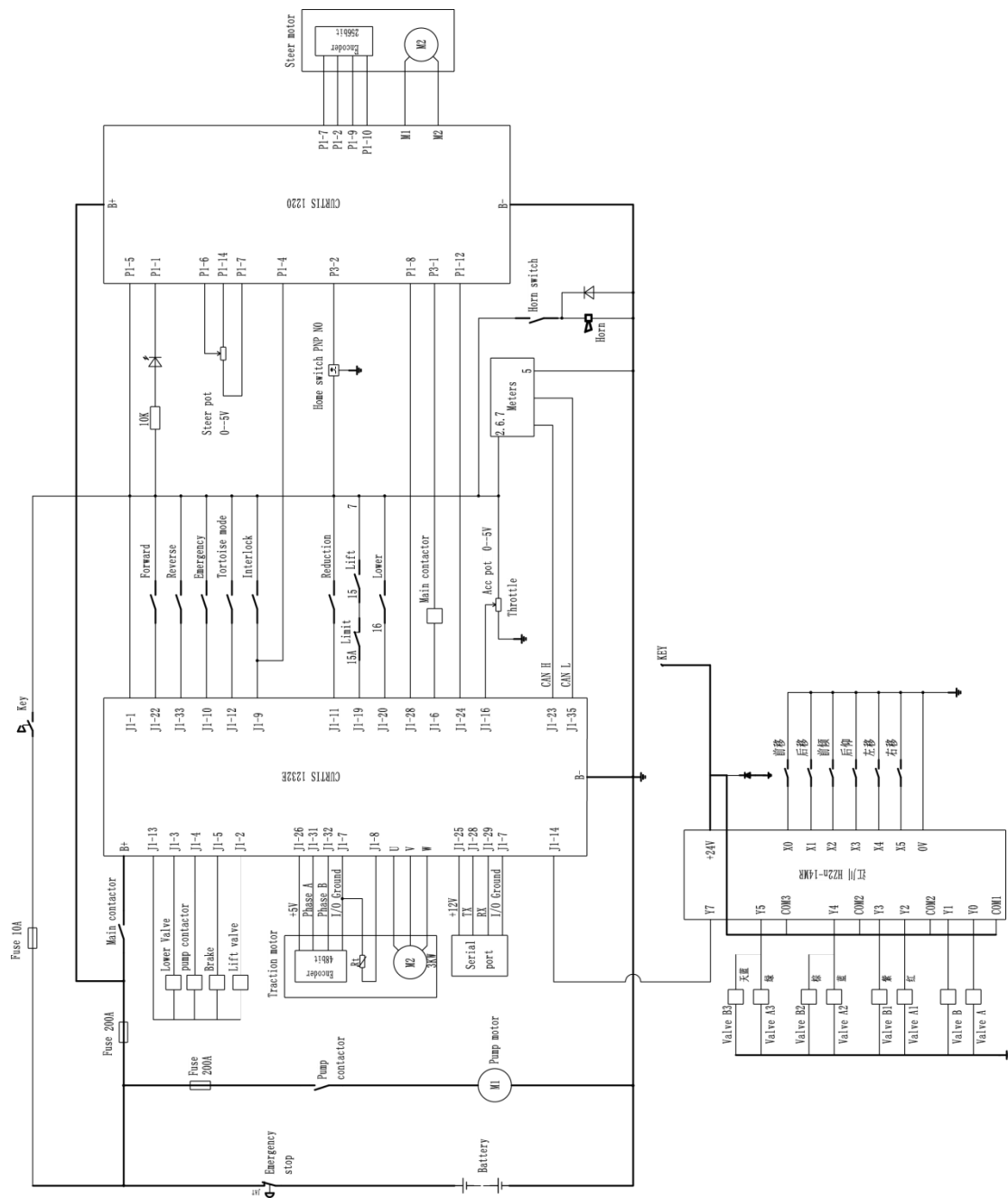
图 36 三级电磁阀式电气原理图
