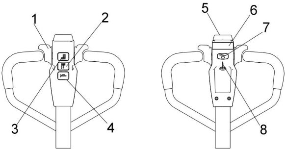
图 9 操作手柄
