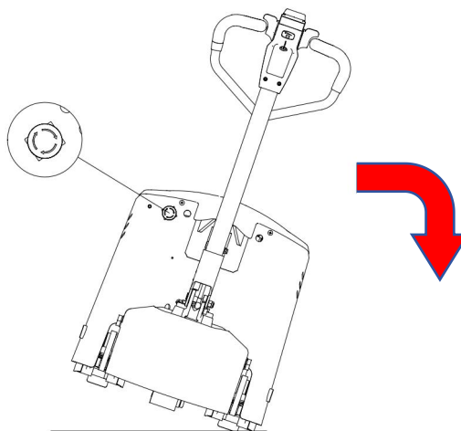
图 20 车辆倾覆
