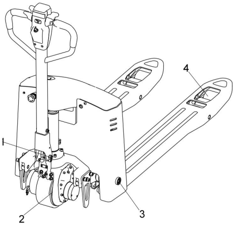
图 26 润滑点
