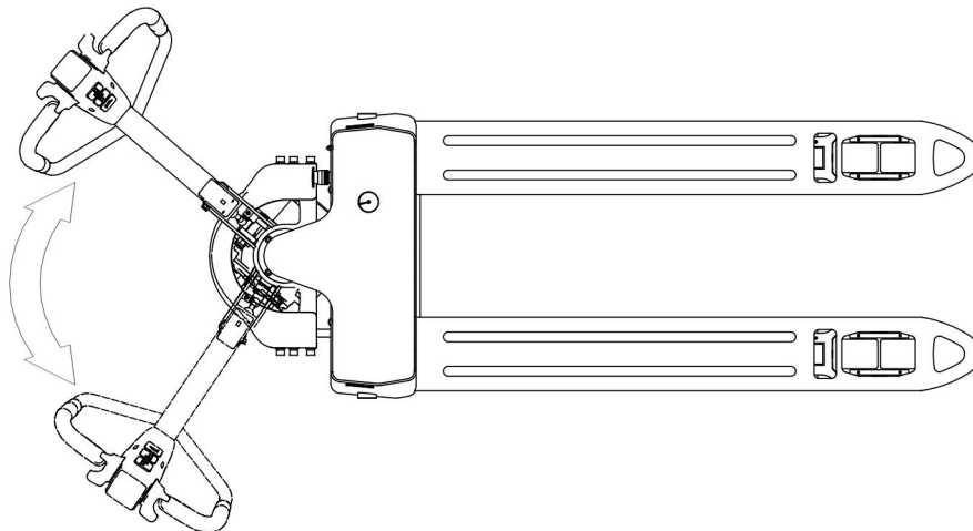
图 14 转向示意图
