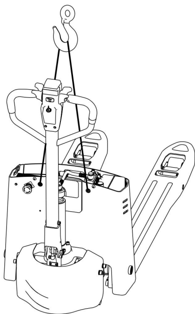
图 6 起吊
