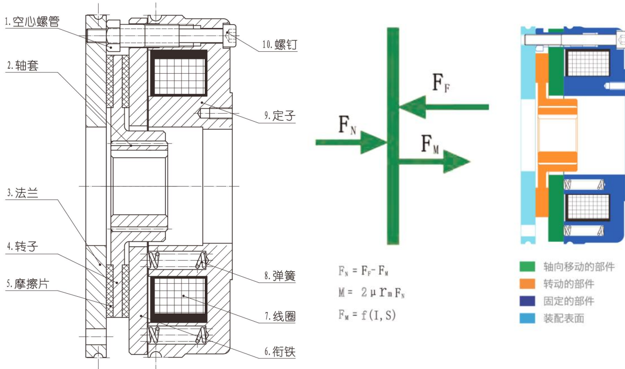
图 17 制动原理图
