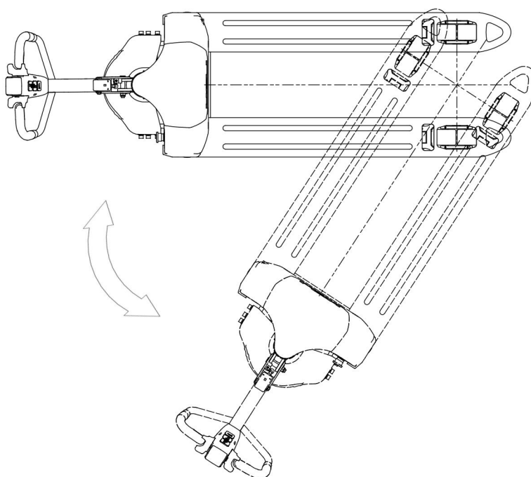
图 15 转弯轨迹示意图
