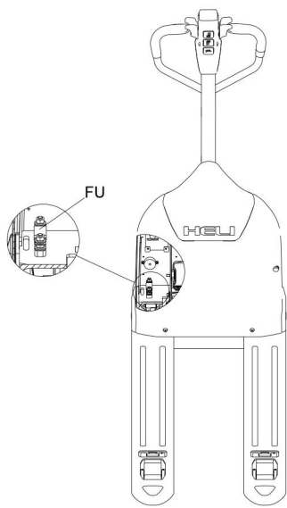
图 28 保险丝位置
