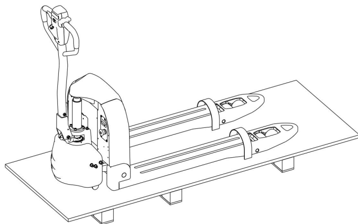
图 7 固定点
