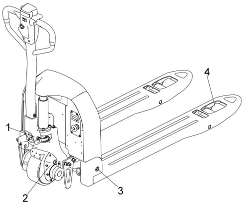
图 27 润滑点
