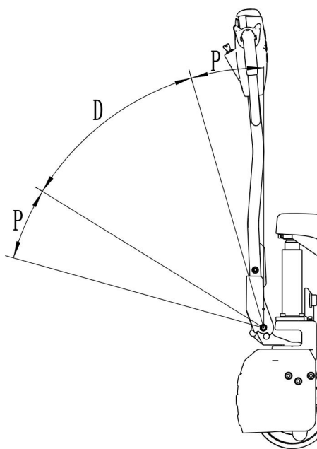
图 16 操纵杆角度
