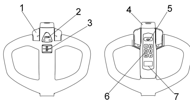
图 10 智能手柄
