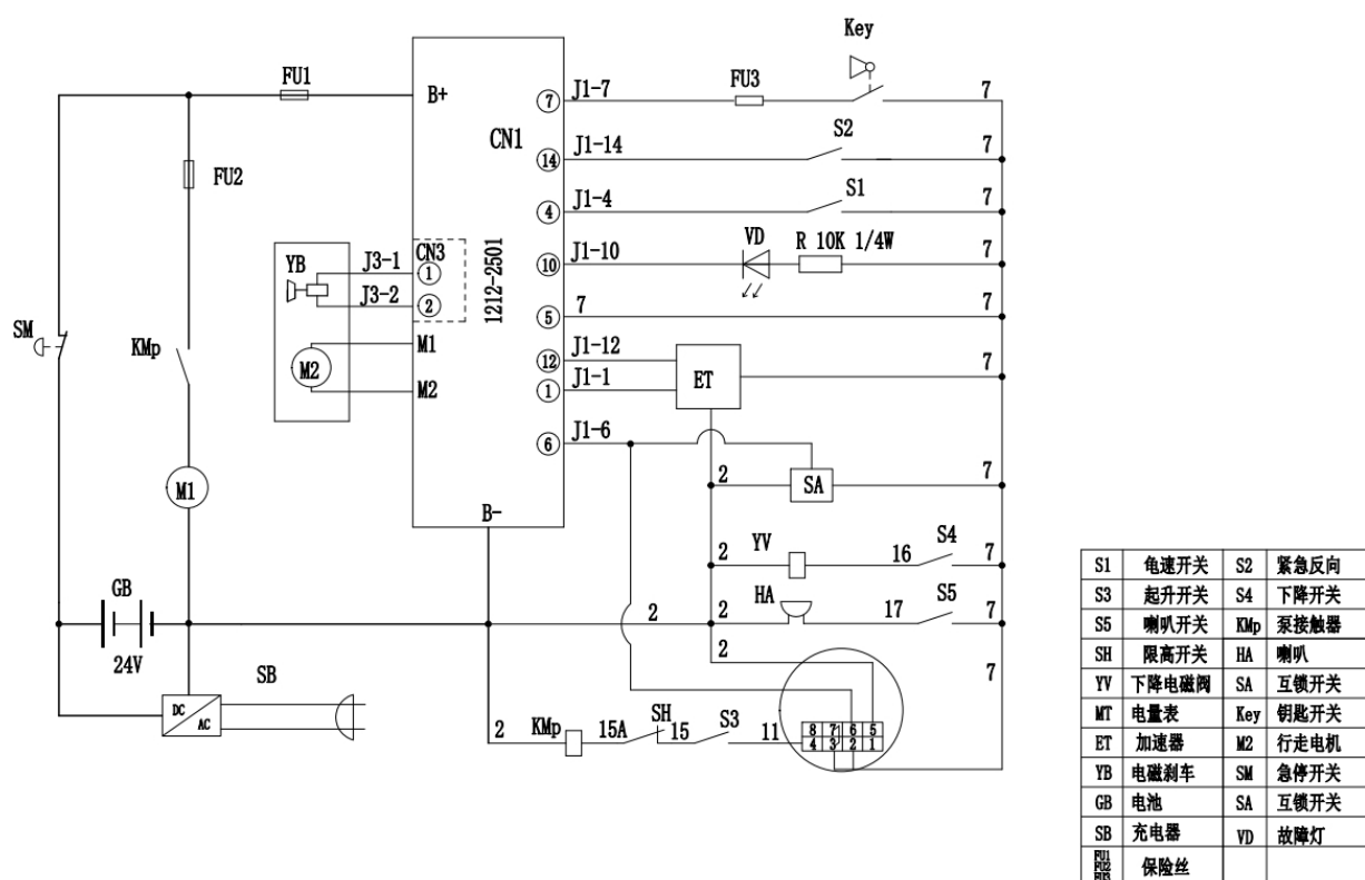
图 15-1 电气原理图 (车体带电量表)
