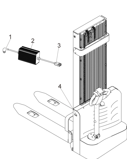
图 10-2-1 外置充电器位置示意图
