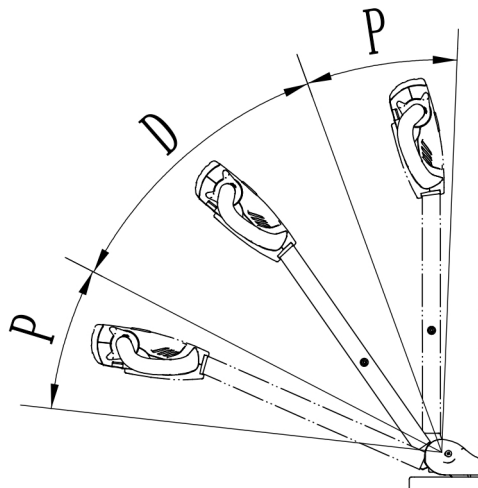
图 8-3 操纵杆角度
