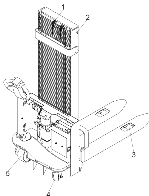
图 13-1 润滑点
