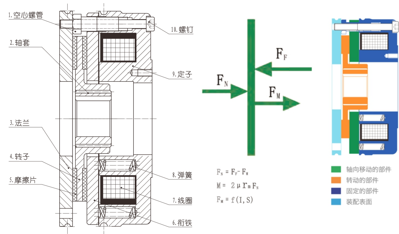
图 8-4 制动原理图
