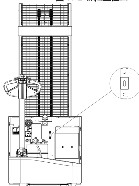
图 13-2 保险丝位置
