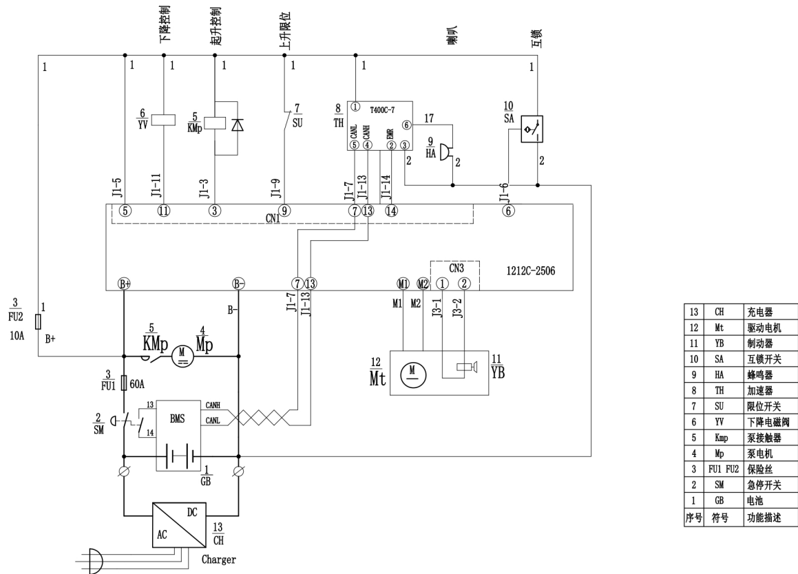
图 15-3 电气原理图(智能手柄)
