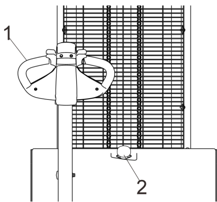
图 7-1 操作控制台
