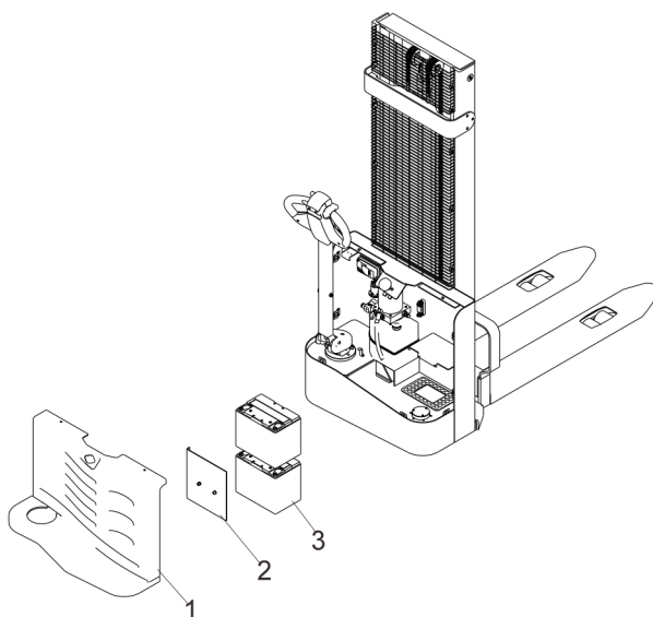
图 10-1 电池更换示意图
