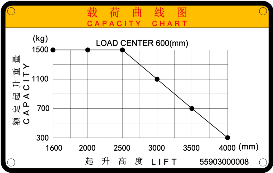
图 3-5 载荷曲线示意图
