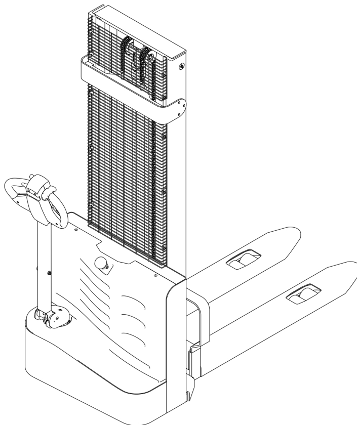
图 1-1 CL15GB-CH 电动托盘堆垛车
