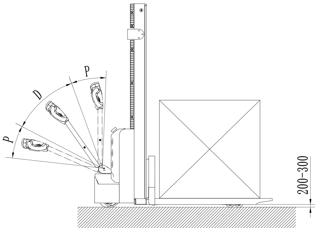
图 9-1 载荷行驶示意图
