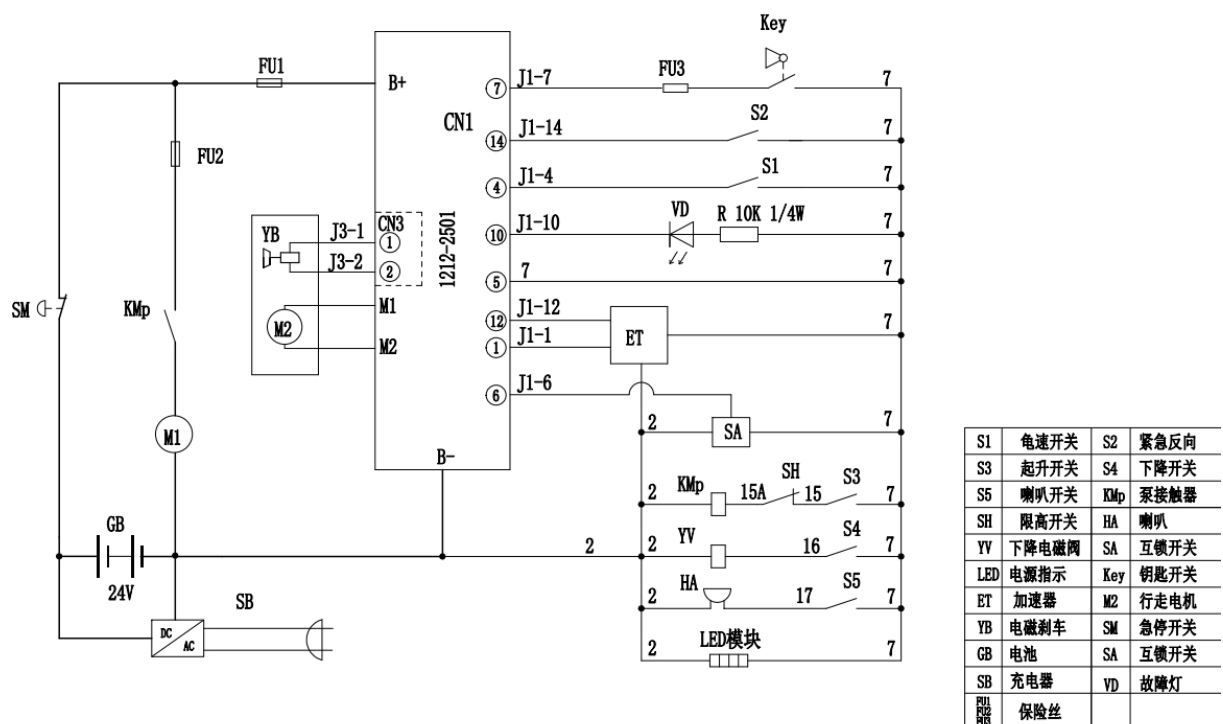
图 15-1 电气原理图 (车体带电量表)
