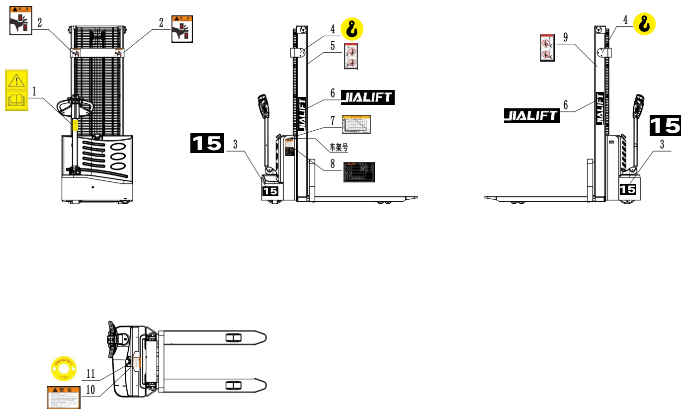
图 3-3 标贴描述
