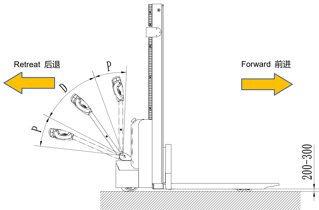
图 8-1 行驶示意图
