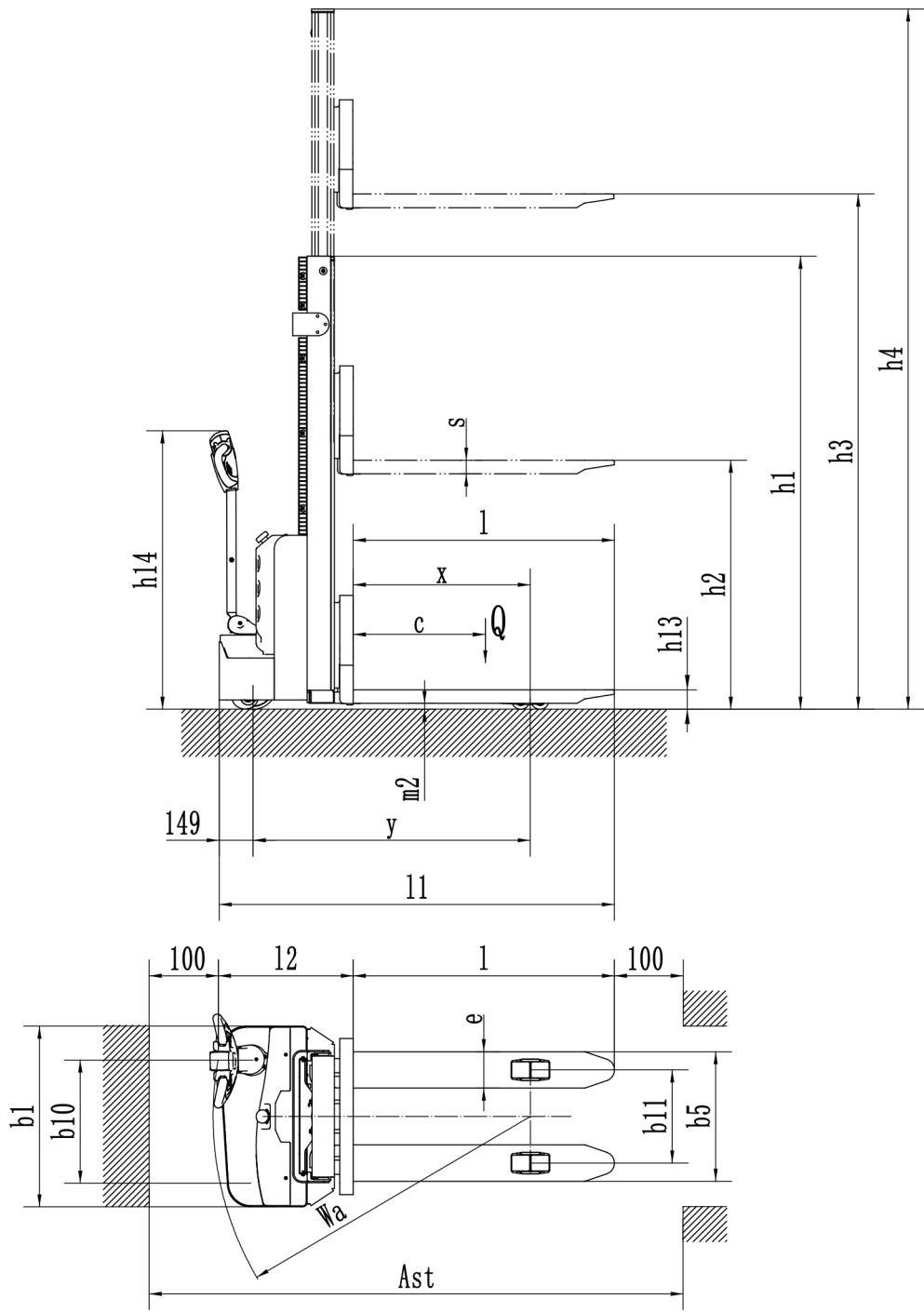
图 3-2 技术参数图
