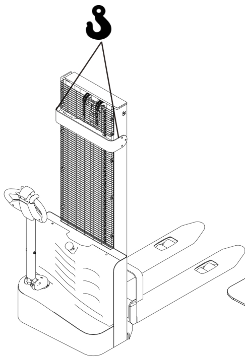
图 5-1 起吊
