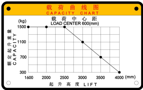
图 3-6-1 载荷曲线图 1.5t
