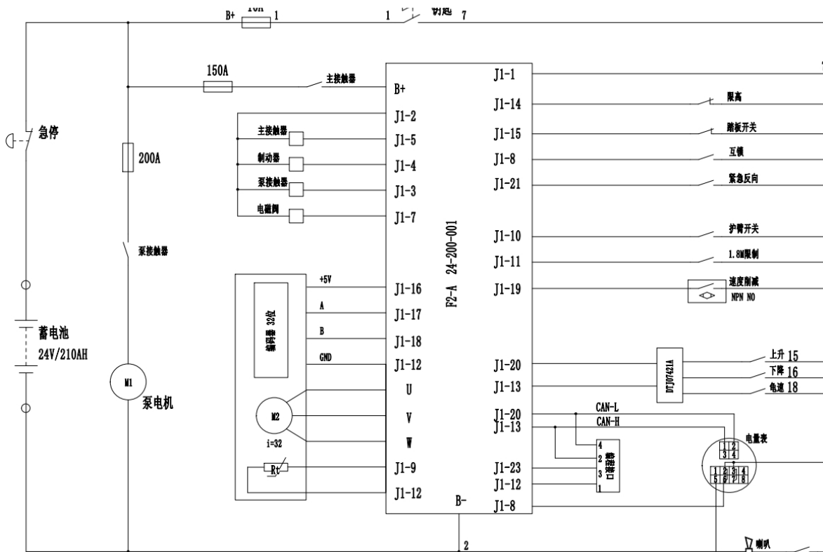
图 15-2 电气原理图 (柯蒂斯控制器)
