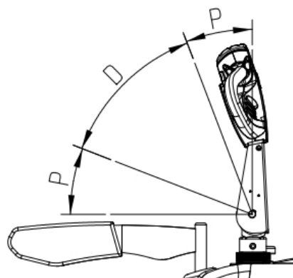
图 8-4 操纵杆角度
