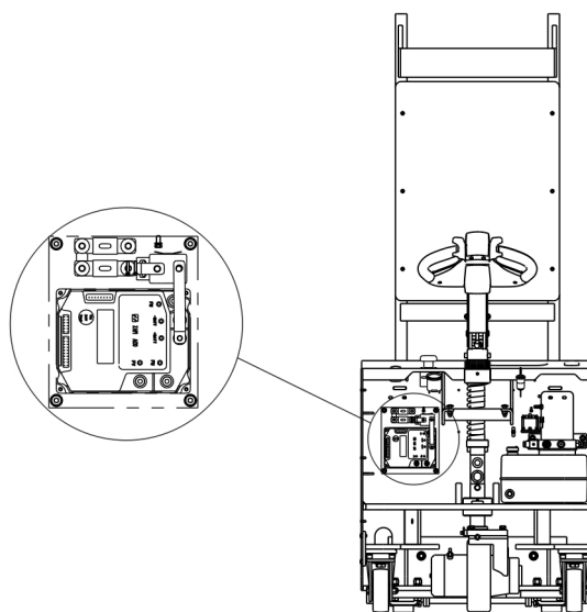
图 13-3 保险丝位置
