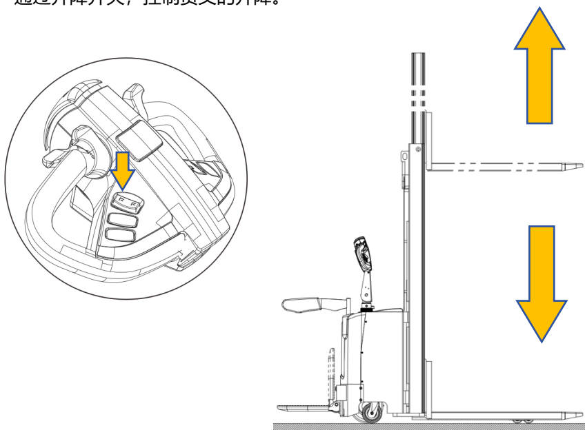
图 8-7 起升示意图
