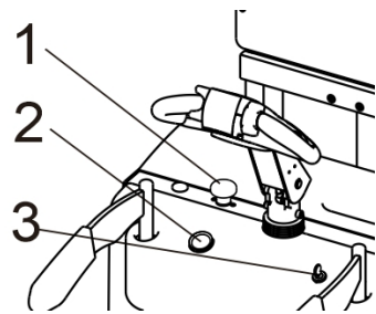
图 7-1-1 操作控制台
