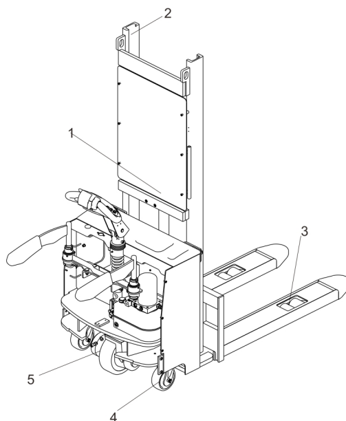
图 13-2 润滑点
