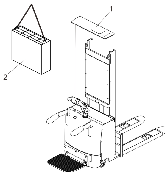
图 10-1 电池更换示意图
