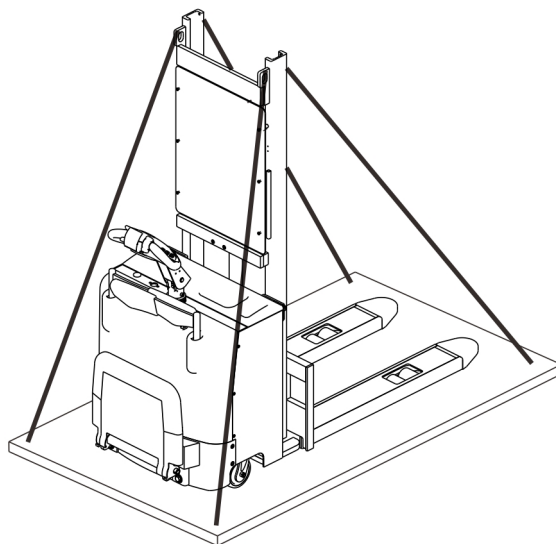
图 5-2-2 固定点
