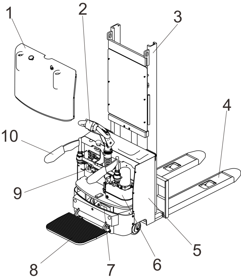
图 3-1 主体分类
