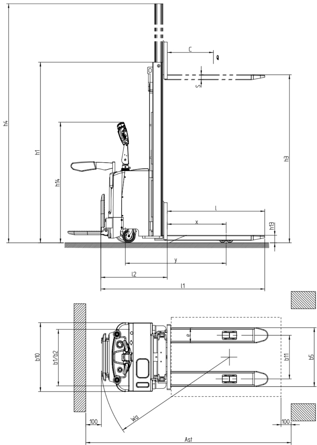
图 3-2 技术参数图
