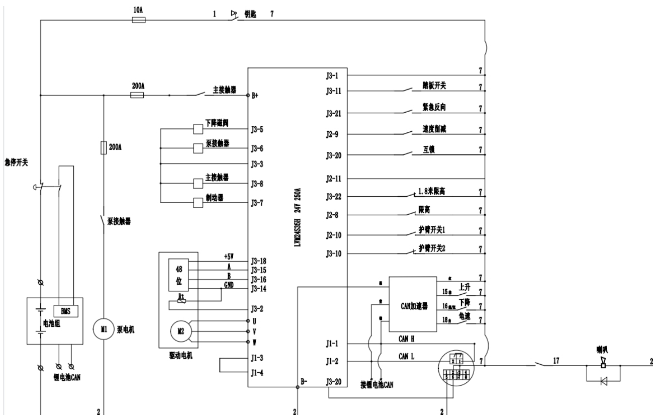
图 15-3 电气原理图 (国产控制器)
