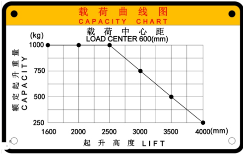
图 3-6-1 载荷曲线图 1.0t
