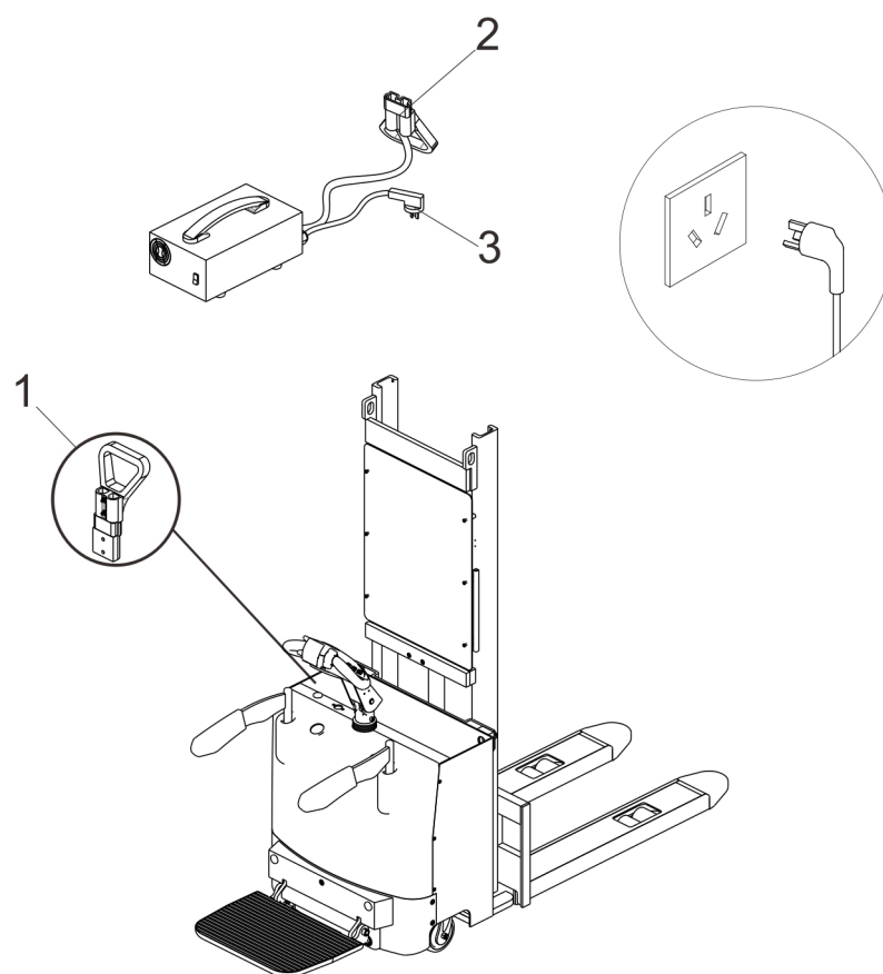
图 10-2-1 充电示意图
