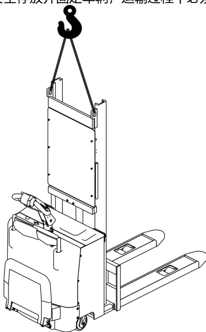
图 5-2-1 起吊
