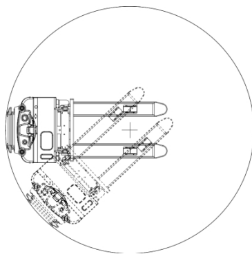
图 8-3 转弯轨迹示意图
