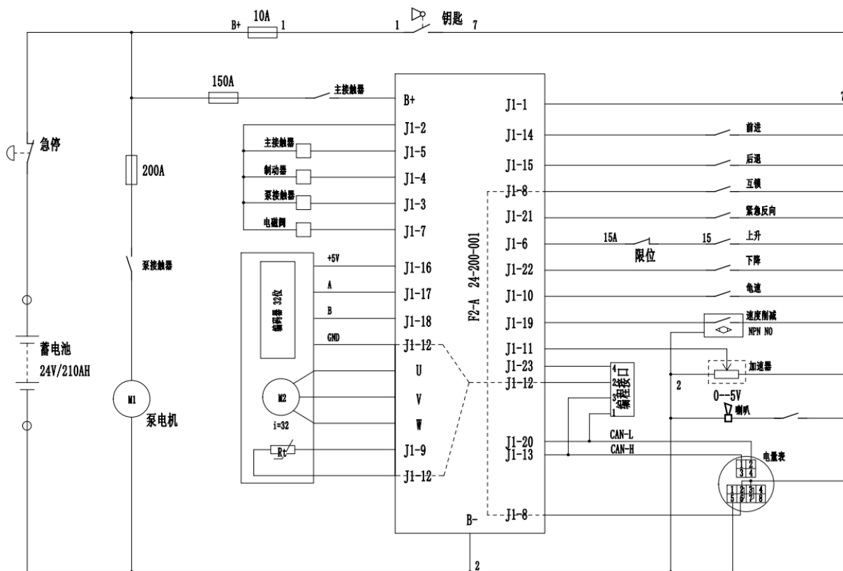
图 15-1 电气原理图 (柯蒂斯控制器, 老款机械转向)
