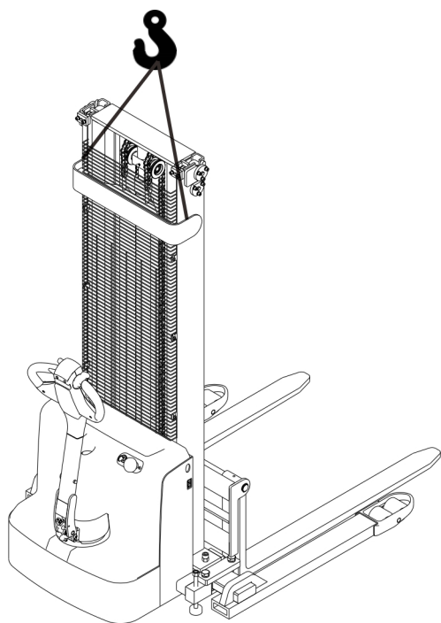
图 5-1 起吊
