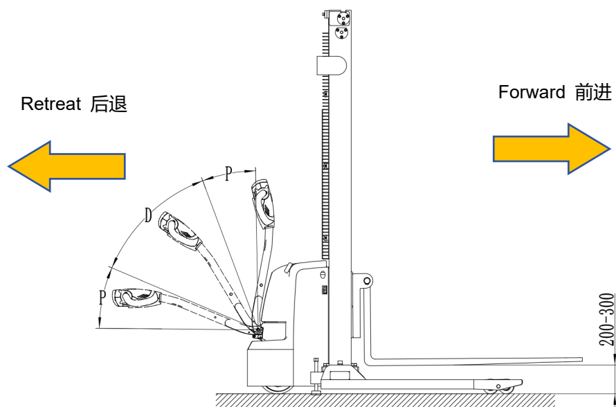
图 8-1 行驶示意图
