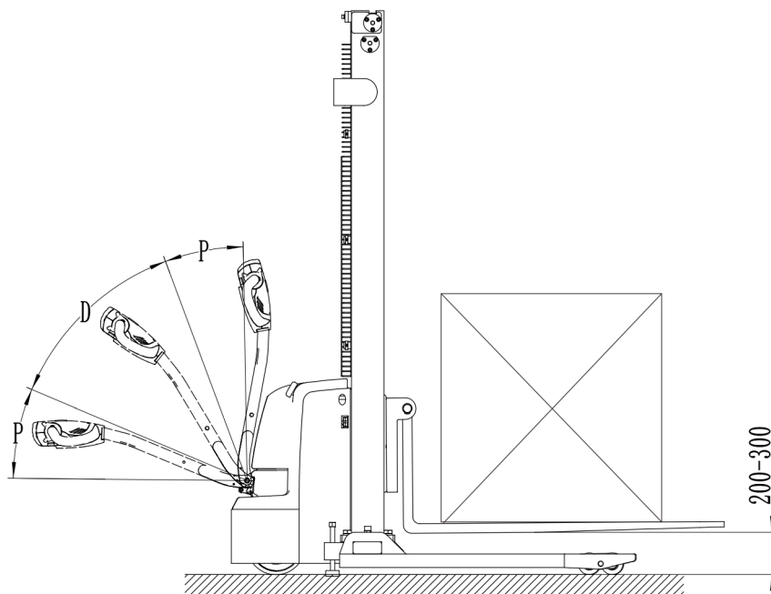
图 9-1 载荷行驶示意图
