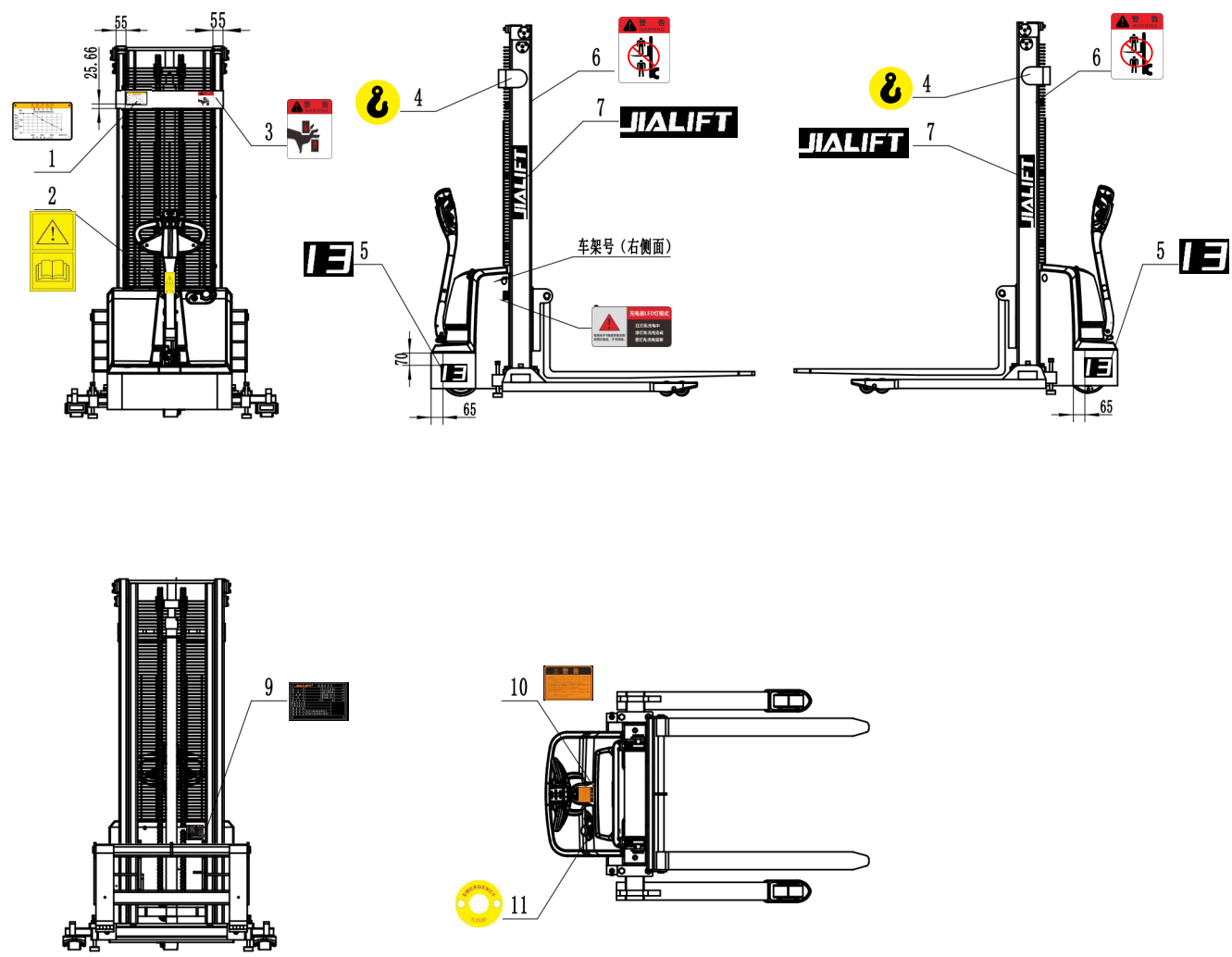
图 3-3 标贴描述
