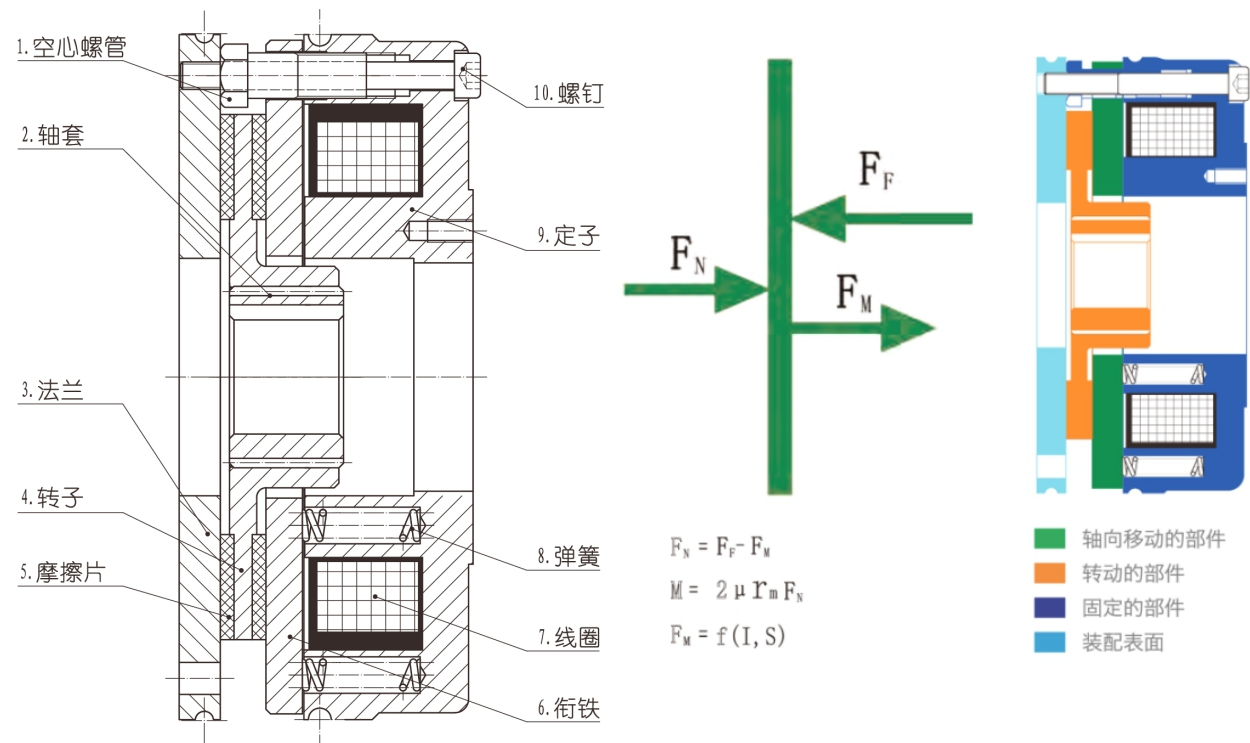
图 8-4 制动原理图
