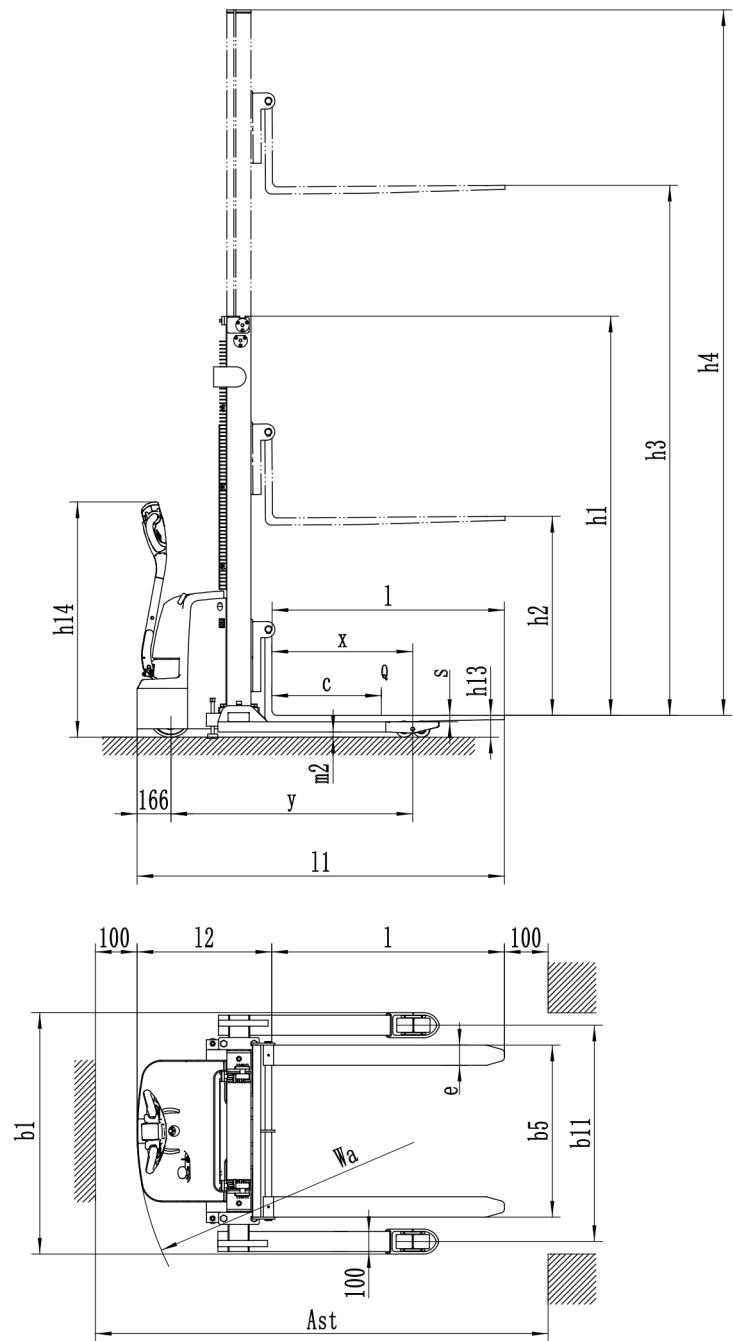
图 3-2 技术参数图
