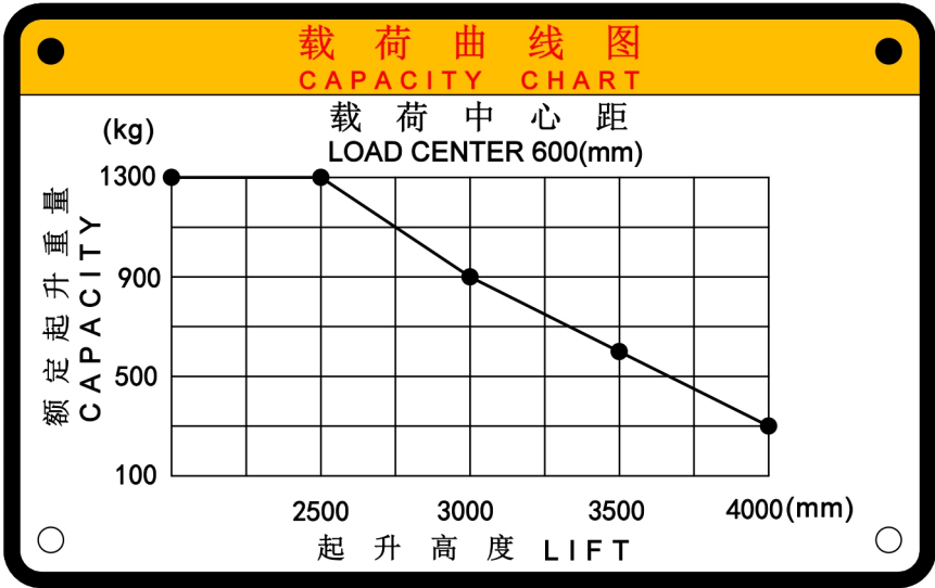
图 3-5 载荷曲线示意图
