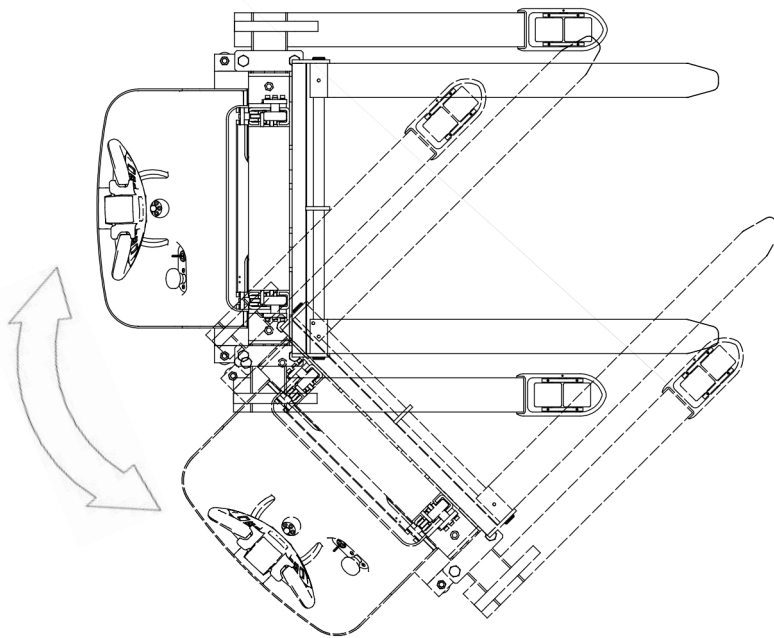
图 8-2 转向示意图
