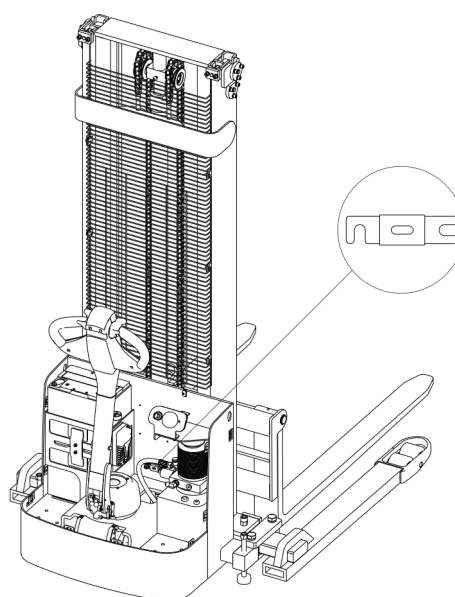
图 13-2 保险丝位置
