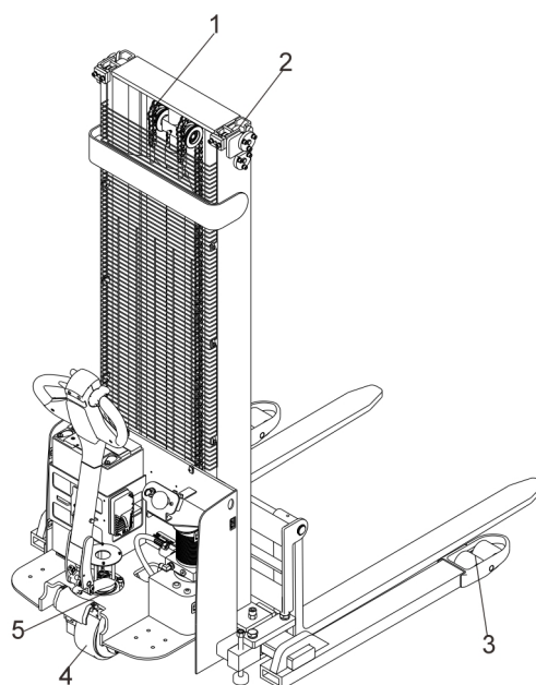
图 13-1 润滑点
