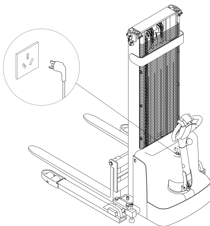
图 10-2 充电口位置示意图
