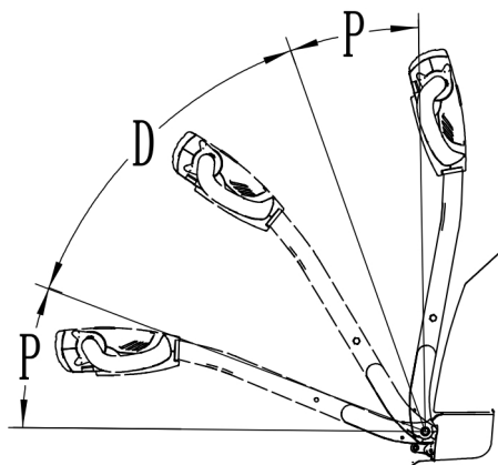
图 8-3 操纵杆角度
