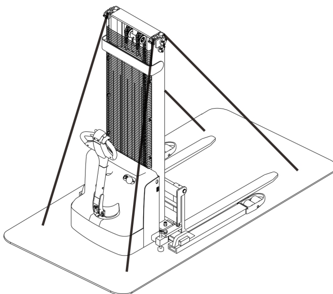
图 5-2 固定点
