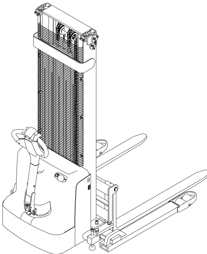
图 1-1 CL13GHY 电动托盘堆垛车（插腿式）
