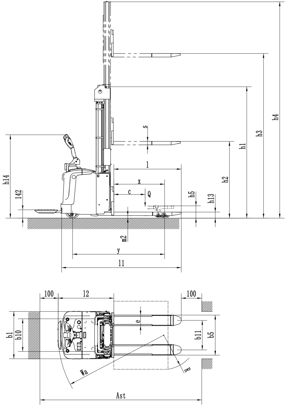
图 3-2 技术参数图
