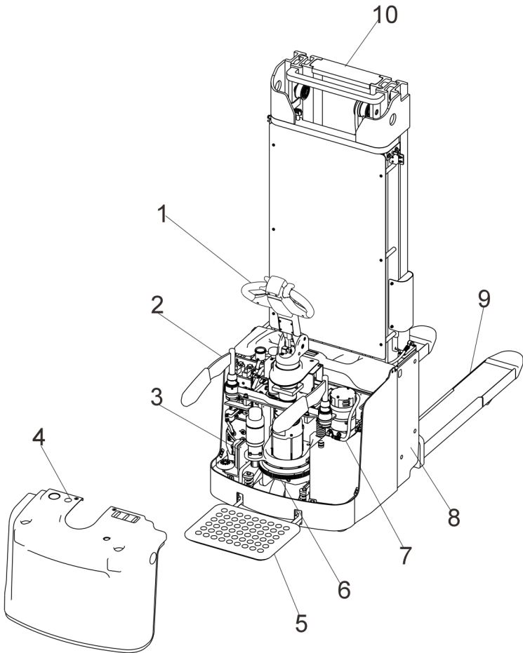
图 3-1 主体分类
