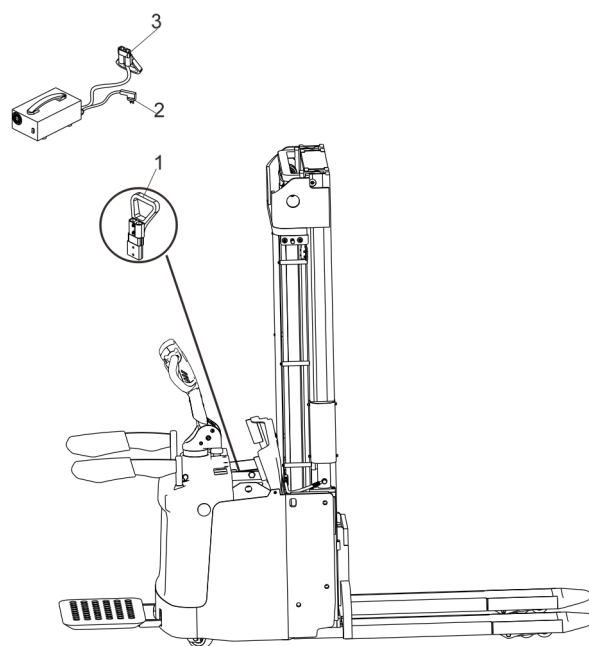
图 10-2 充电器充电示意图
