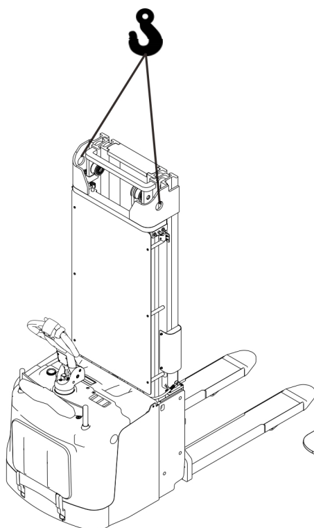
图 5-1 起吊
