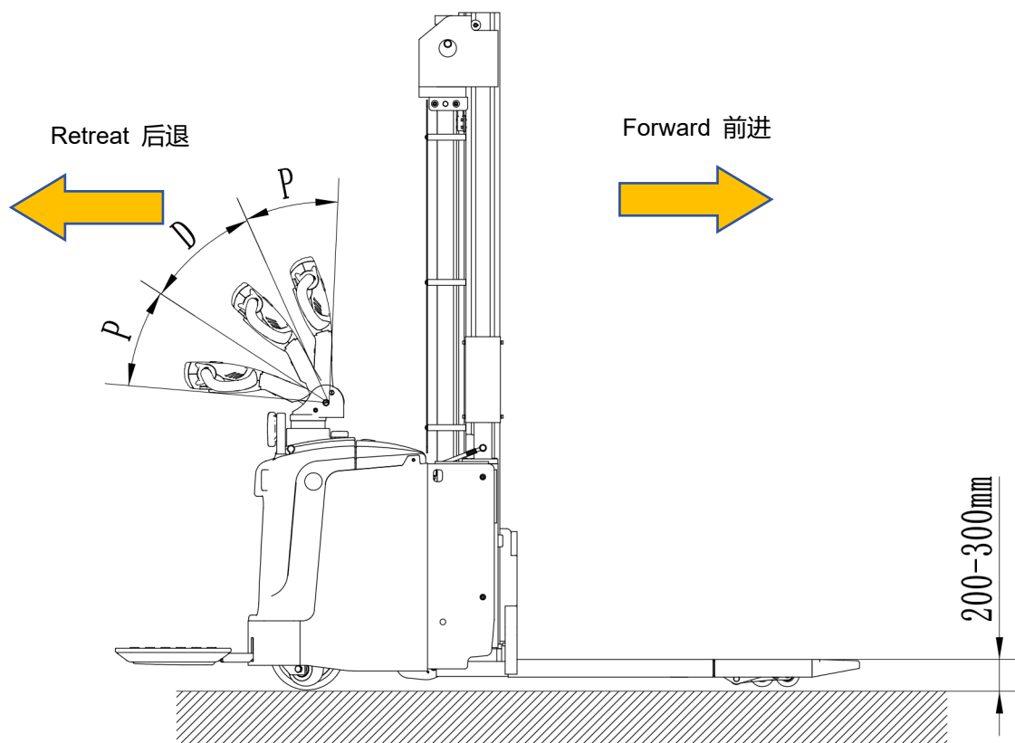
图 8-1 行驶示意图
