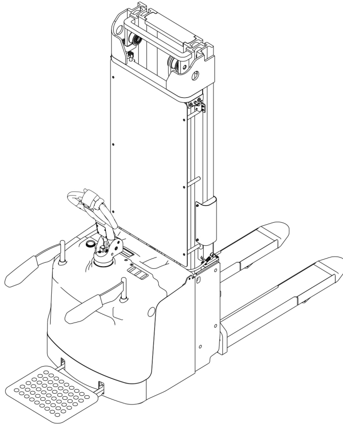
图 1-1 CL15-20GC 电动托盘堆垛车(双提升)
