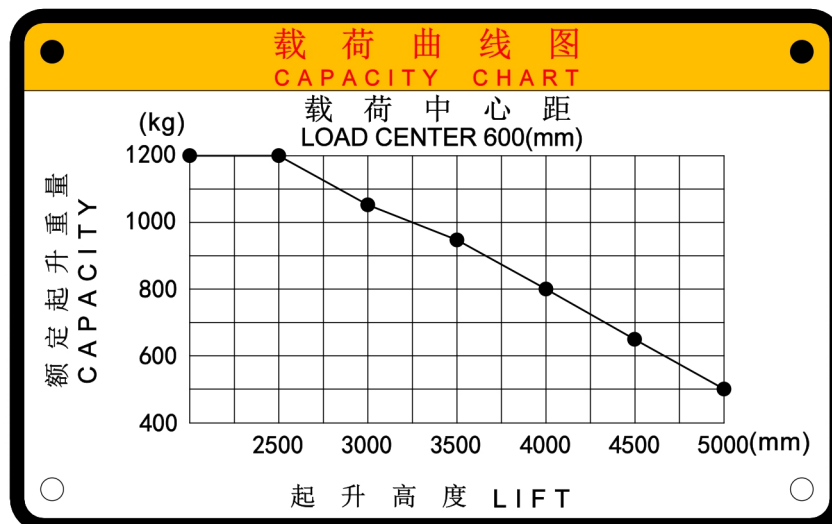
图 3-5-2 2t 载荷曲线示意图
