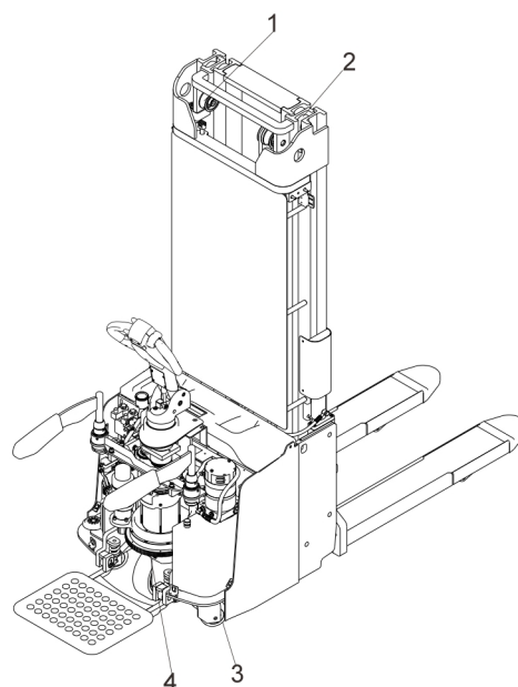
图 13-1 润滑点
