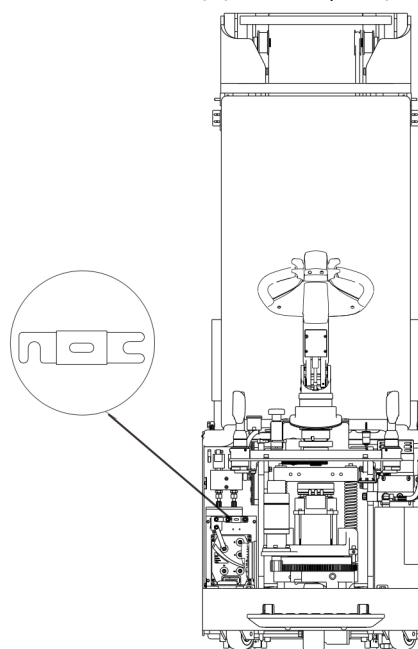
图 13-2 保险丝位置
