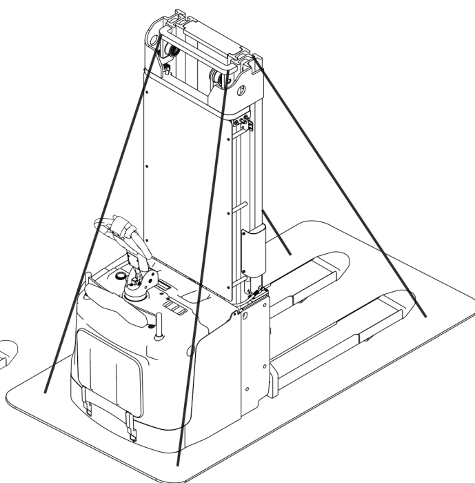
图 5-2 固定点
