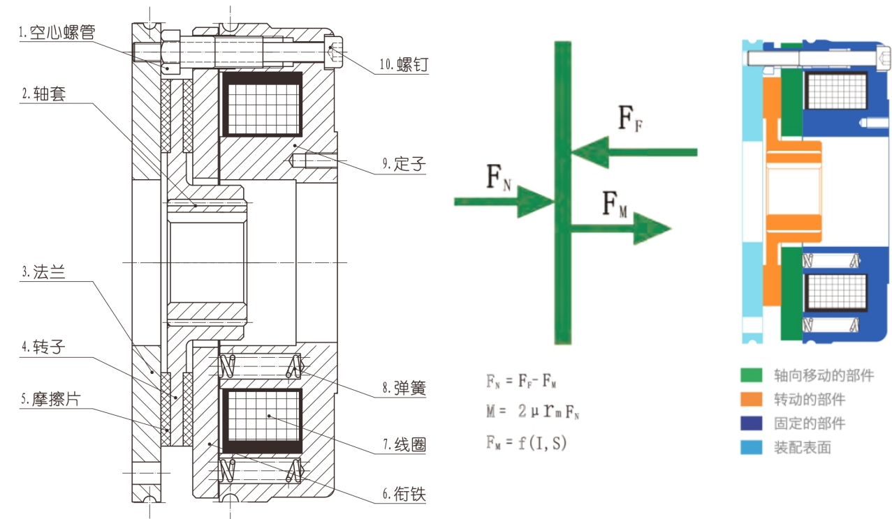
图 8-4 制动原理图
