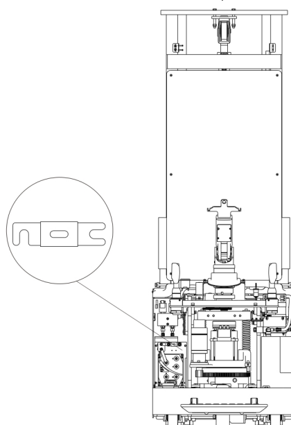
图 13-2 保险丝位置
