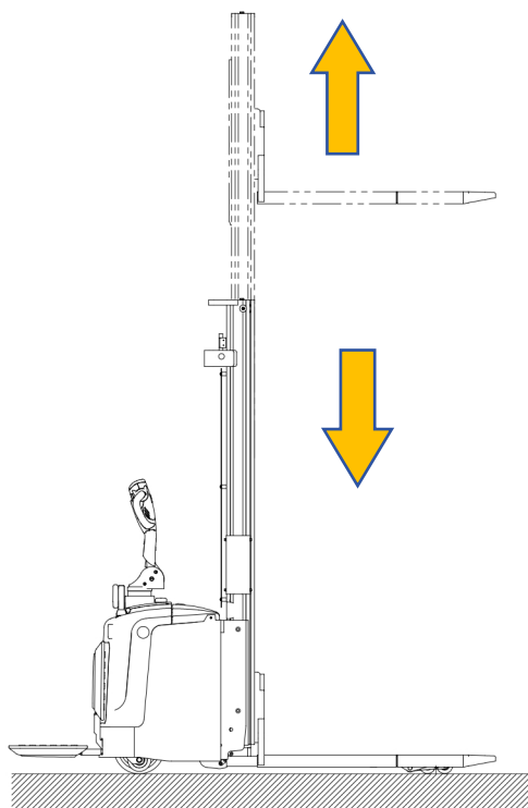
图 8-5 起升示意图
