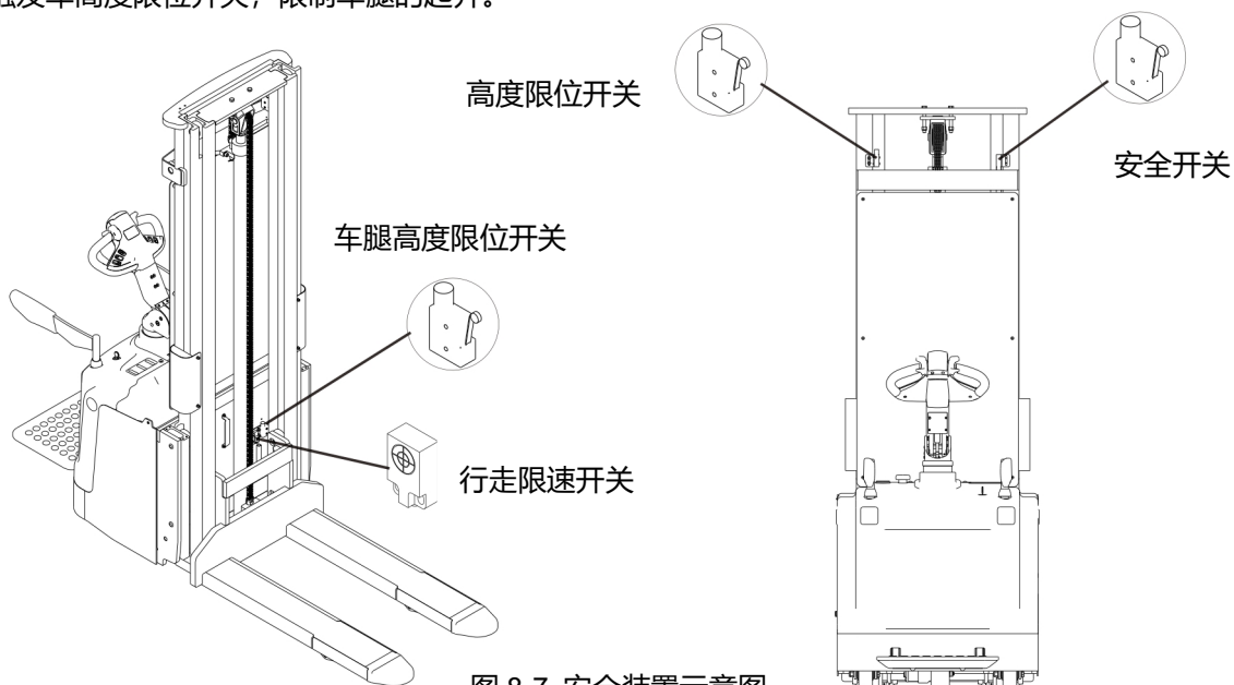
图 8-7 安全装置示意图
