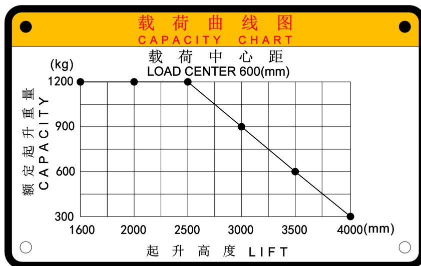
图 3-5-2 2t 载荷曲线示意图
