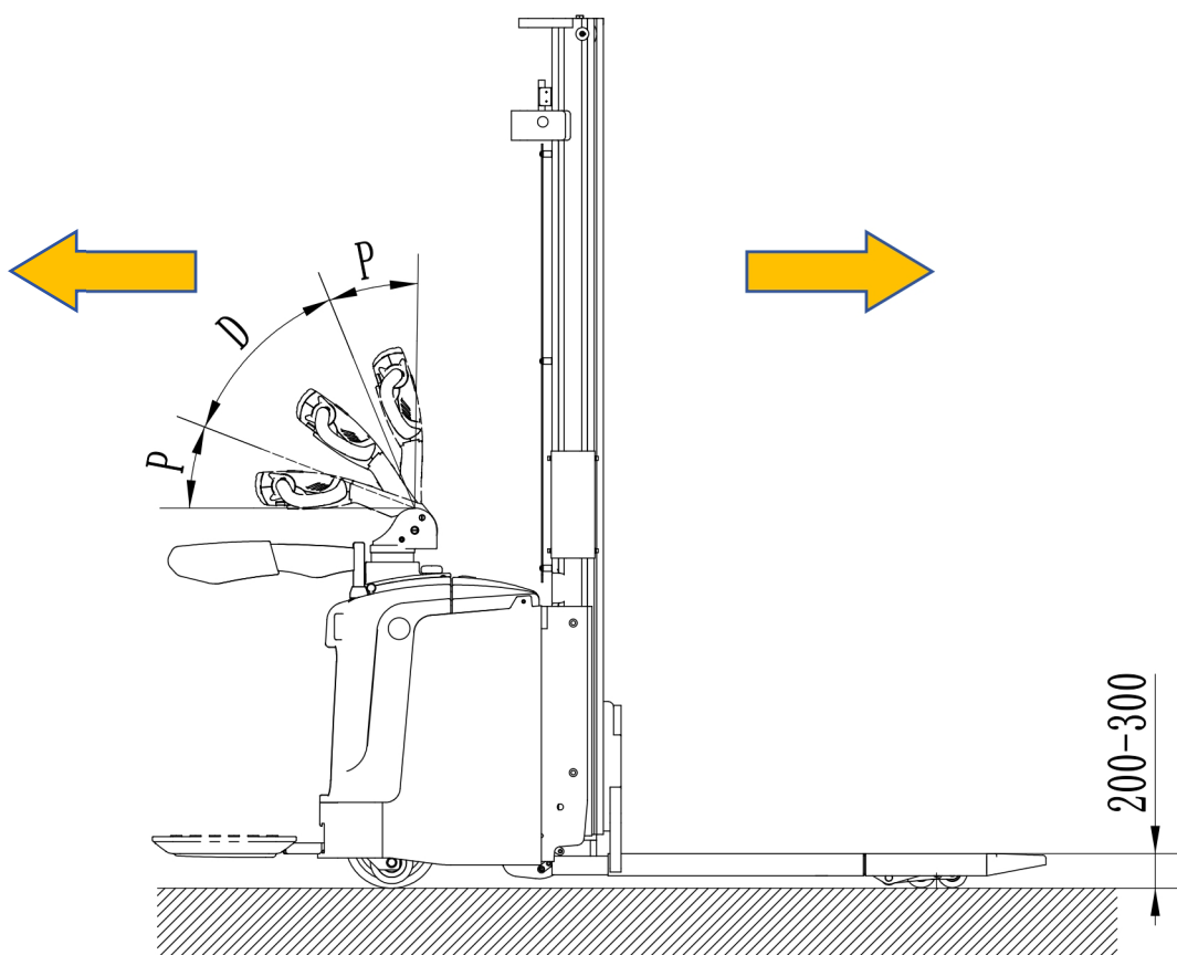
图 8-1 行驶示意图
