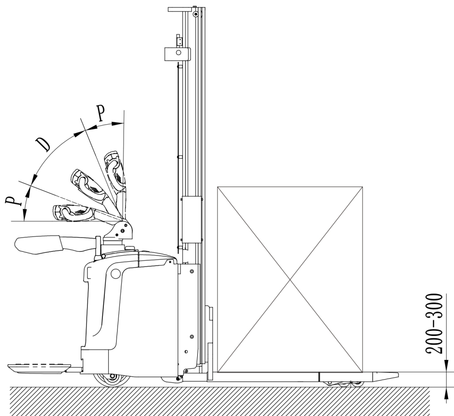
图 9-1 货物提升 200mm—300mm
