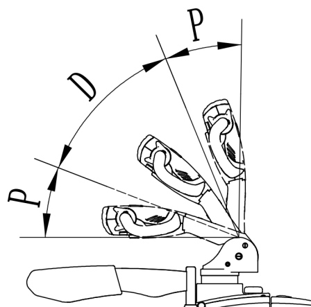
图 8-3 操纵杆角度
