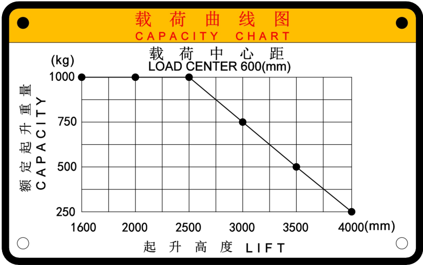
图 3-5-1 1.5t 载荷曲线示意图
