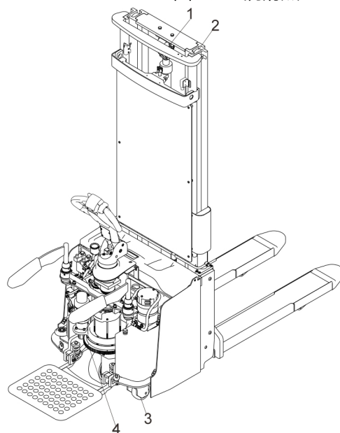
图 13-1 润滑点
