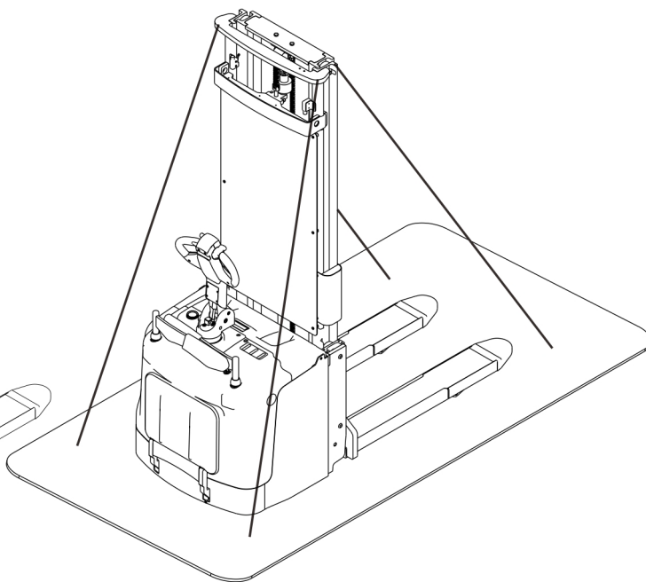
图 5-2 固定点
