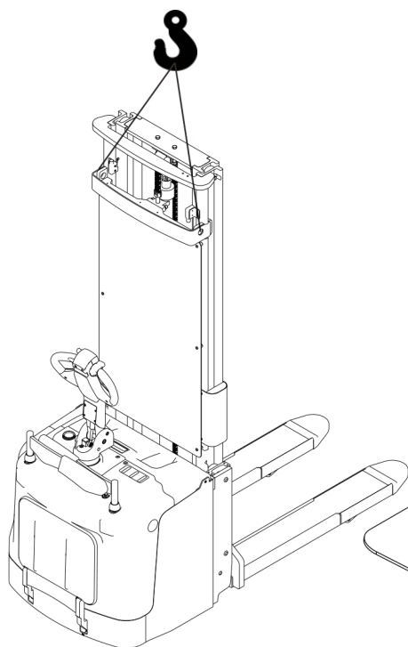
图 5-1 起吊
