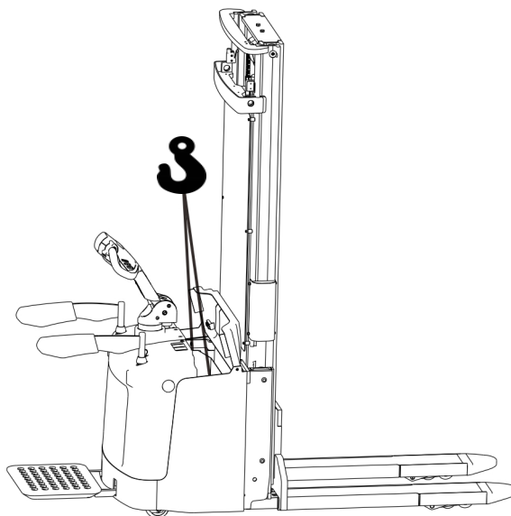
图 10-1 电池更换示意图
