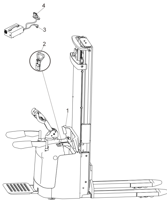
图 10-2 充电器充电示意图
