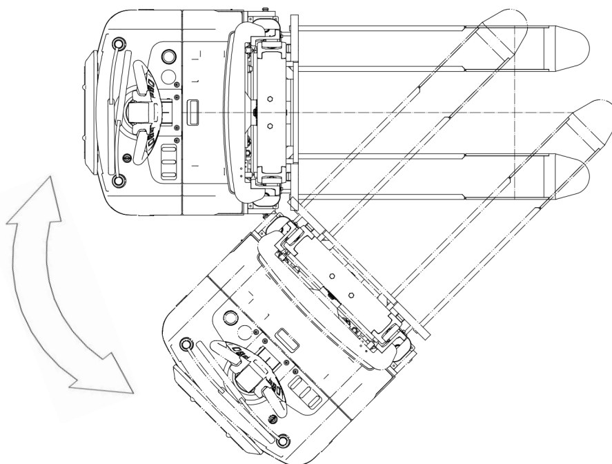
图 8-2 转向示意图
