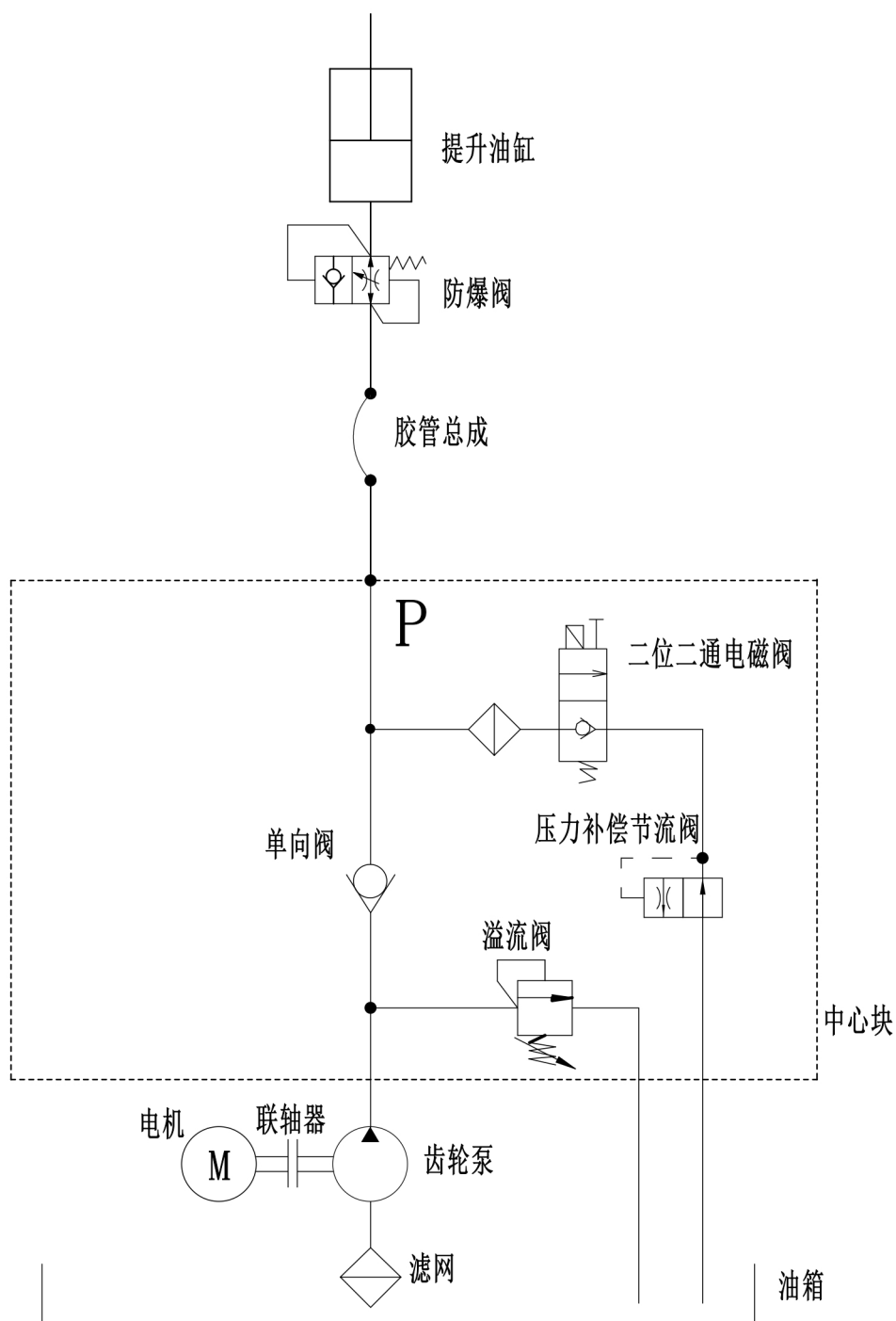
图 16-1 液压原理图
