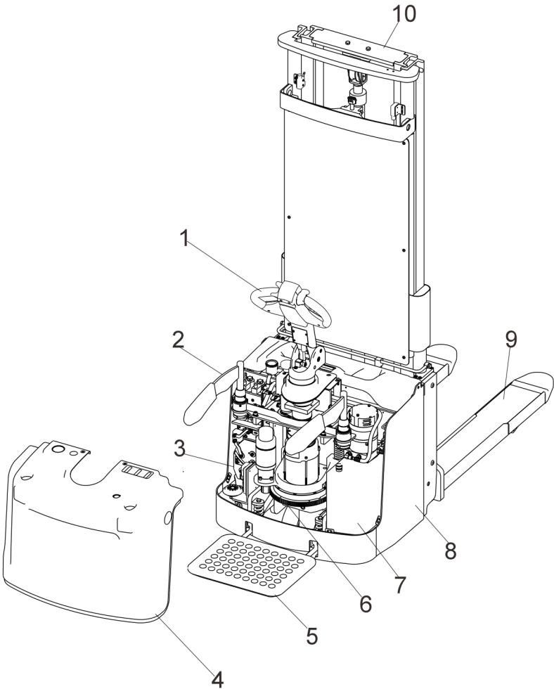
图 3-1 主体分类
