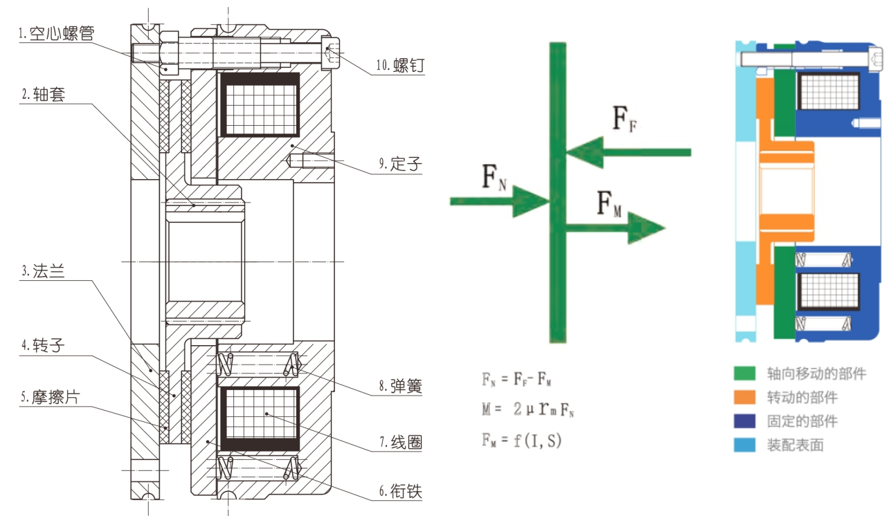
图 8-4 制动原理图
