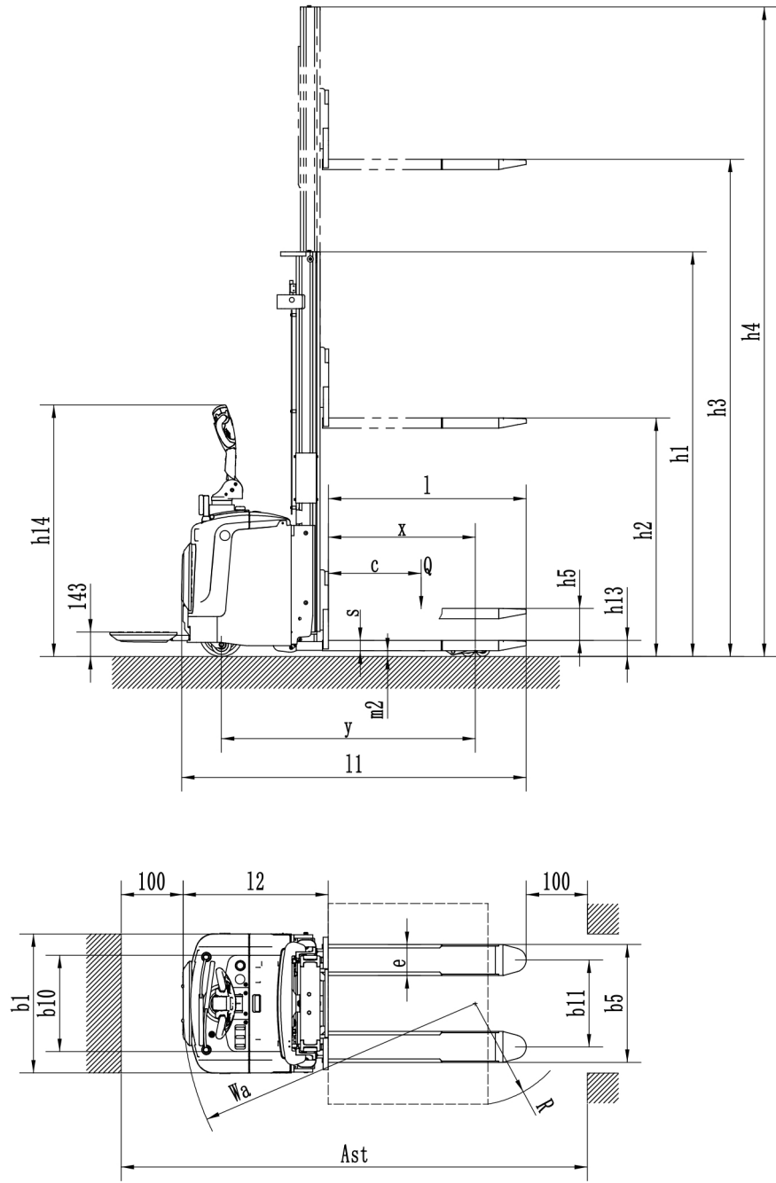
图 3-2 技术参数图
