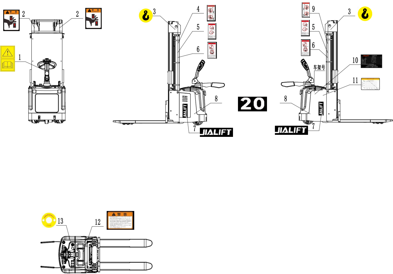
图 3-3 标贴描述
