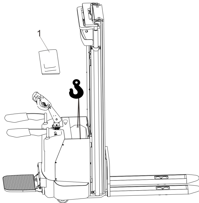
图 10-1 电池更换示意图
