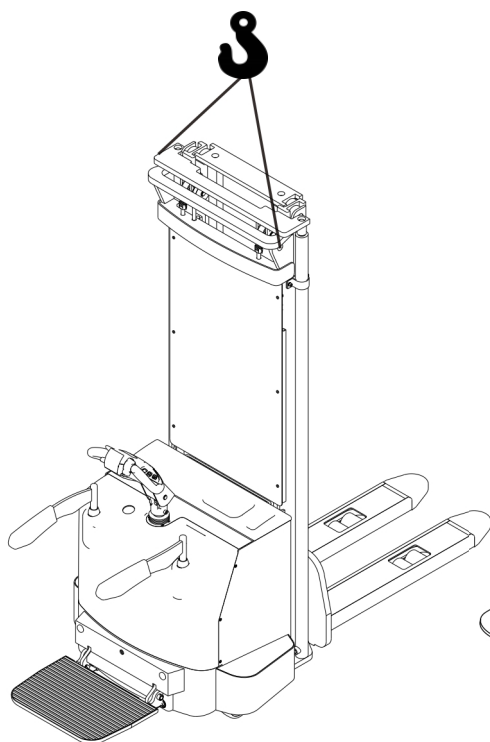
图 5-1 起吊
