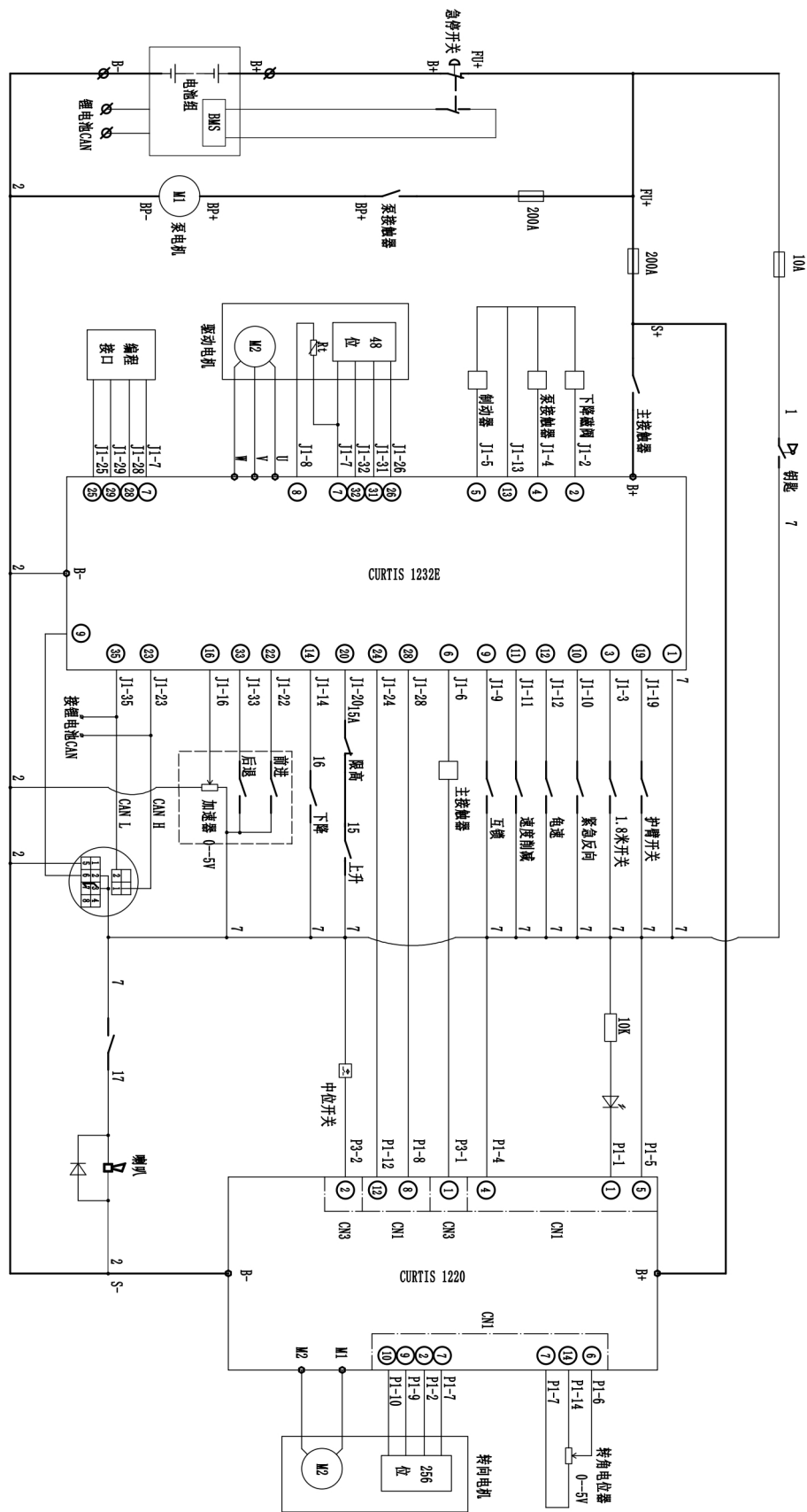
图 15-1 电气原理图
