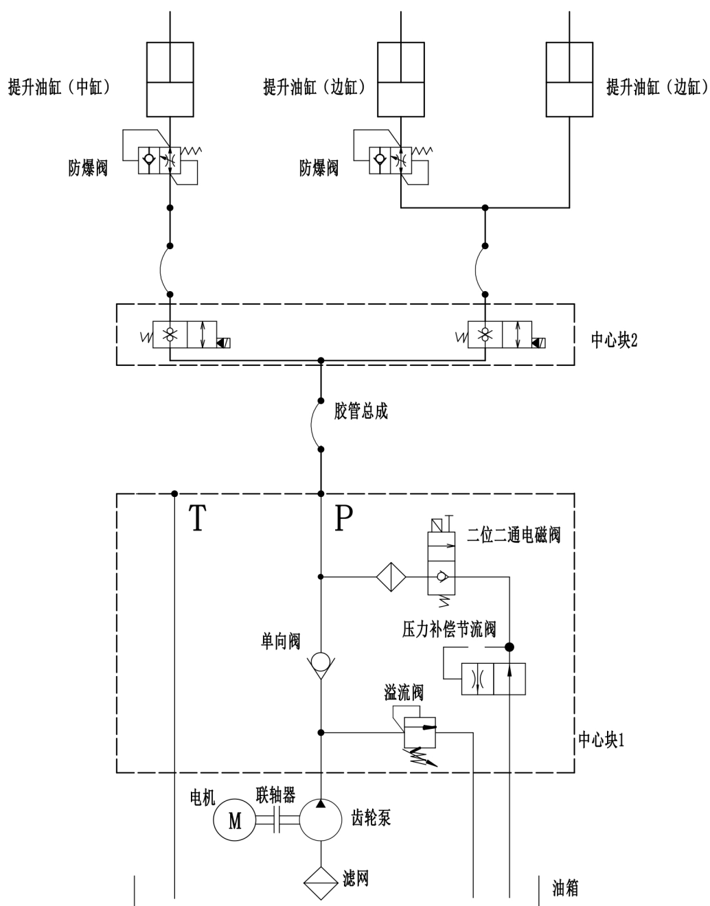
图 16-1 液压原理图
