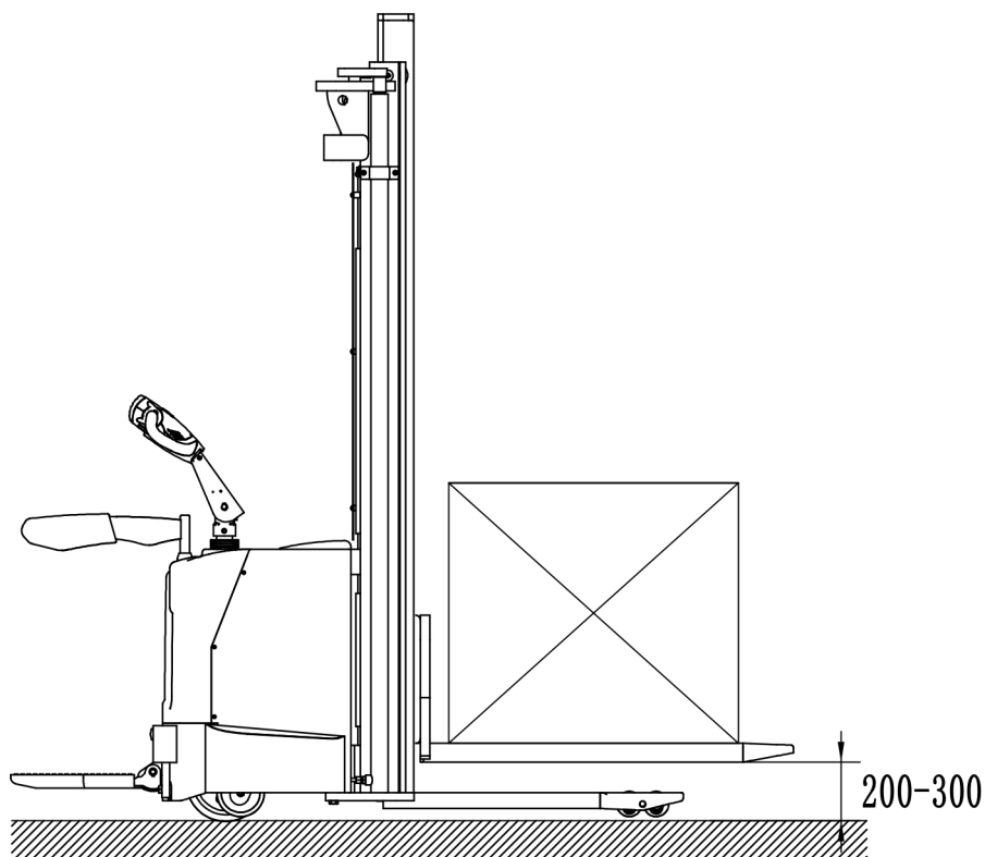
图 9-1 载荷行驶示意图
