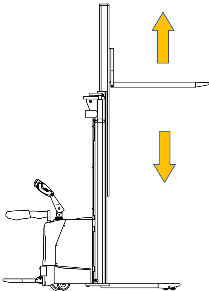
图 8-5 起升示意图
