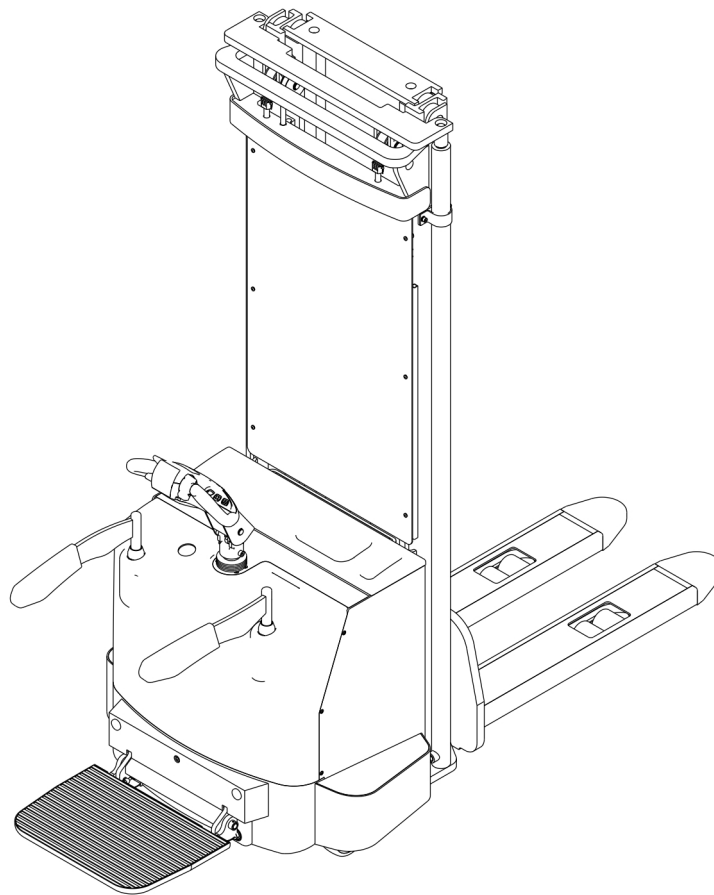
图 1-1 CL1555QD 电动托盘堆垛车
