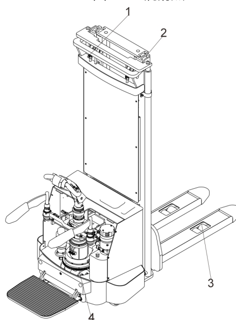
图 13-1 润滑点
