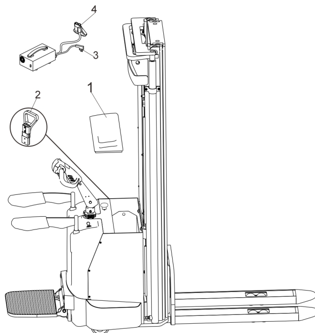
图 10-2 充电口位置示意图
