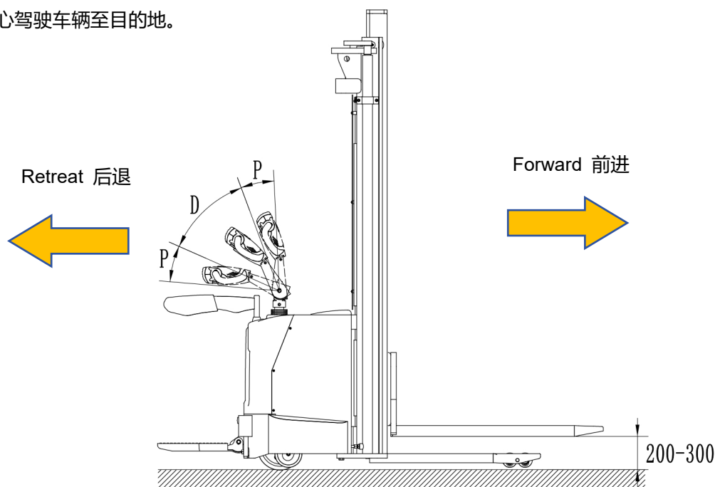
图 8-1 行驶示意图
