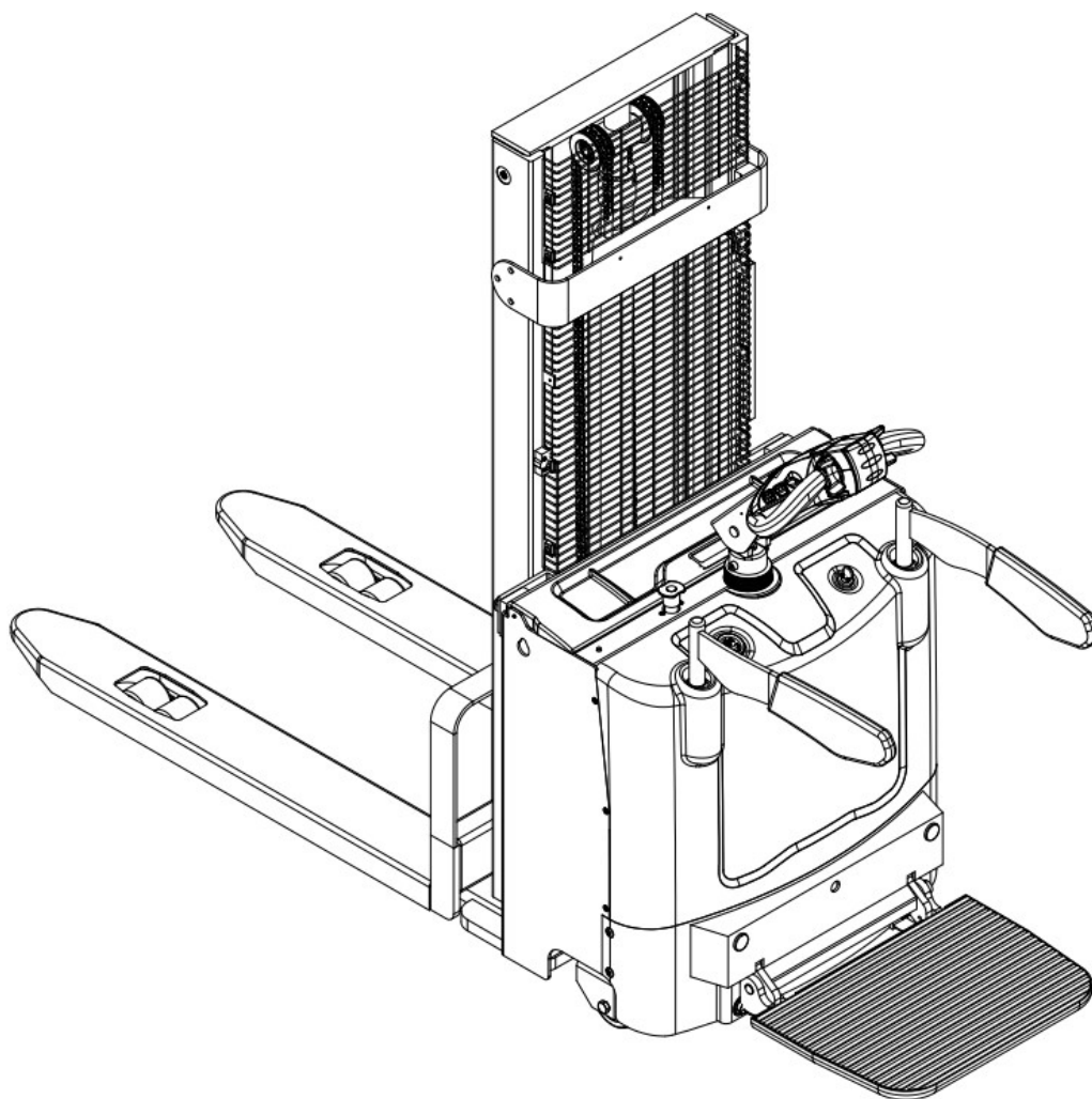
图 1 CL15E-B 电动托盘堆垛车
