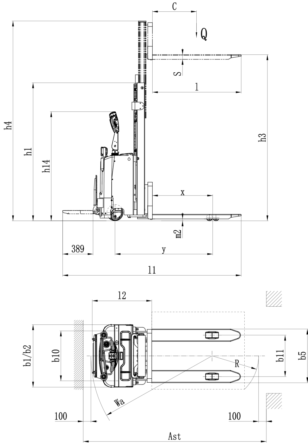
图 3 技术参数图
