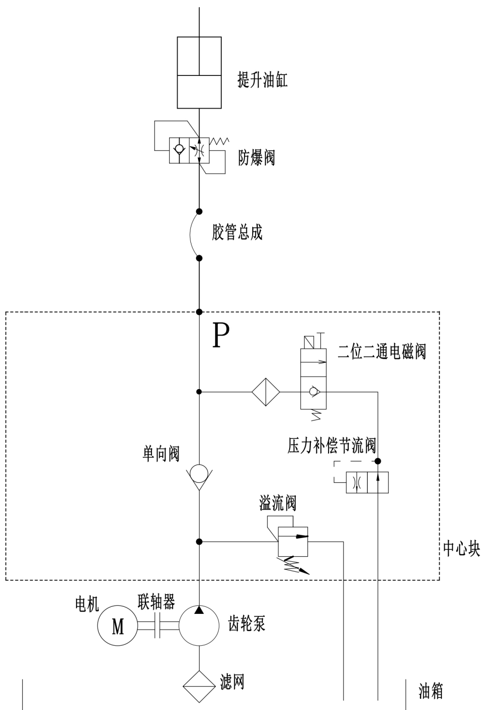
图 33 液压原理图
