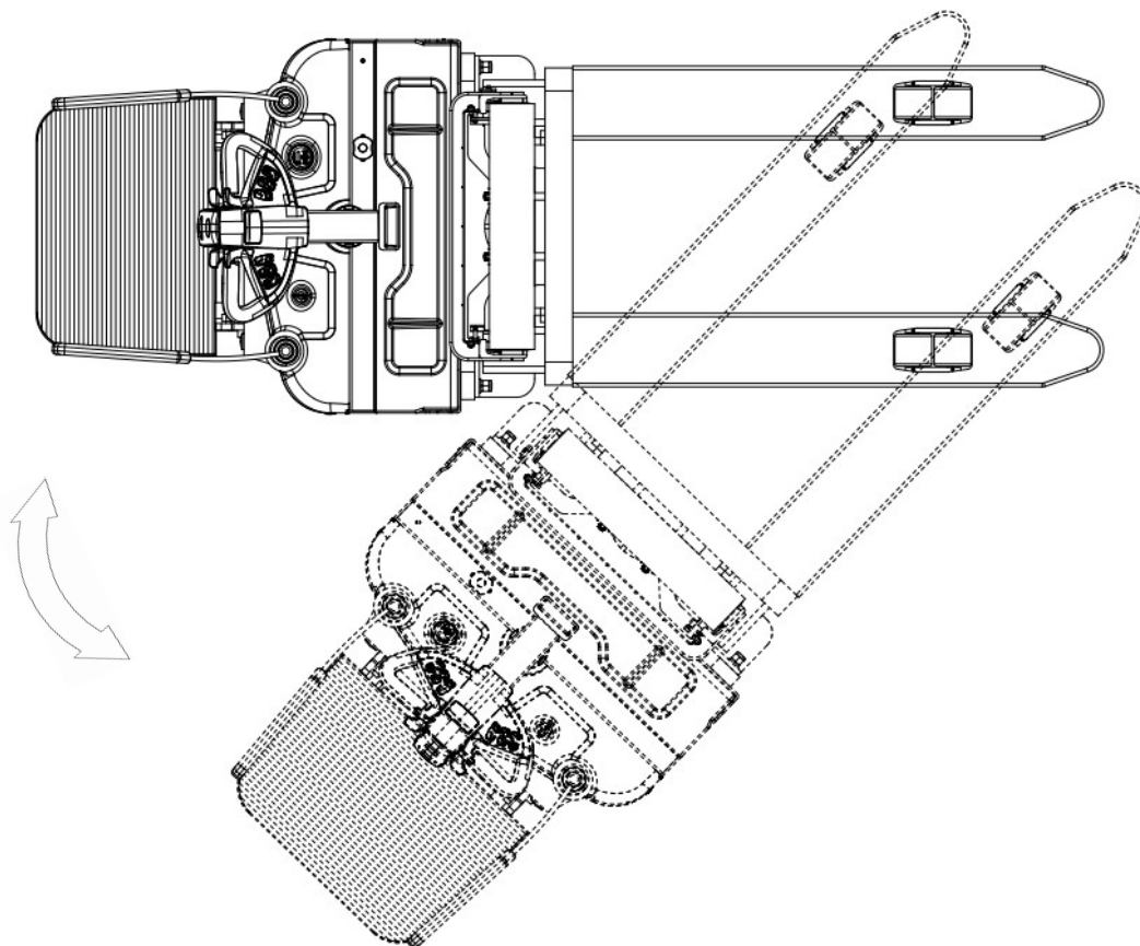
图 16 转弯轨迹
