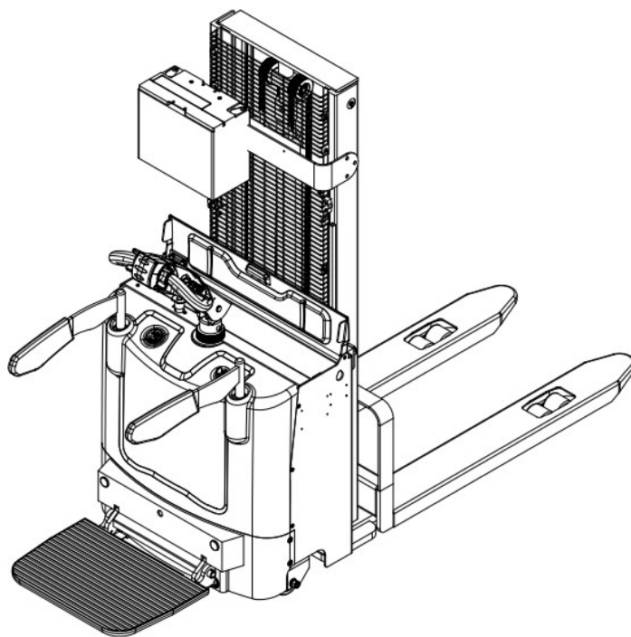
图 25 电池更换
