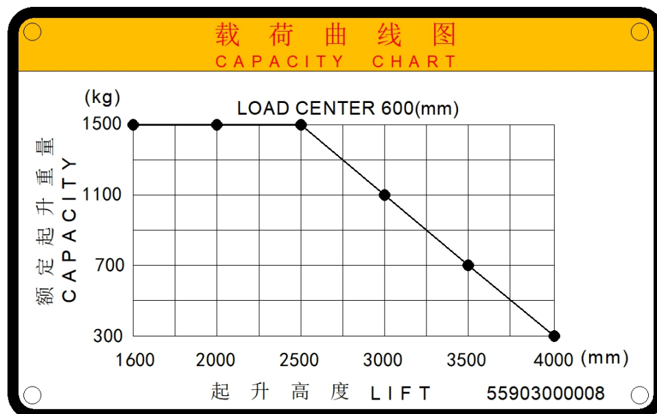
图 6 载荷曲线示意图
