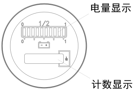
图 28 圆形电量表（锂电池）
