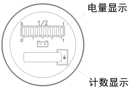
图 27 圆形电量表（蓄电池）
