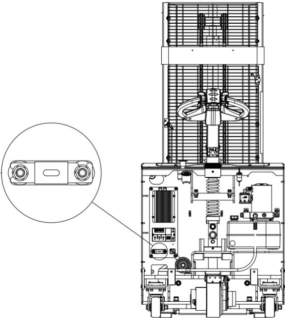
图 31 保险丝位置
