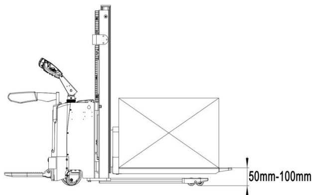
图 23 货物提升 50mm—100mm
