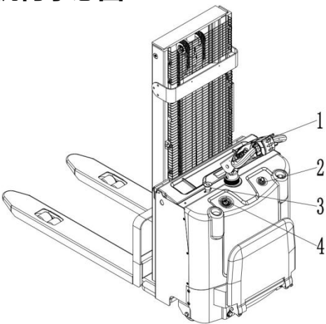
图 9 车辆操作机构
