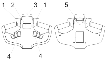
图 11 操作手柄——标准款
