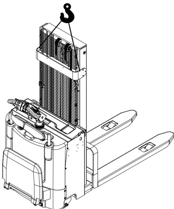
图 7 起吊
