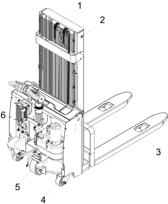
图 30 润滑点
