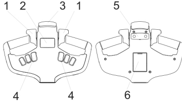
图 13 操作手柄——刷卡器（指纹款）
