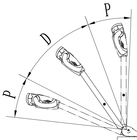
图 8-3 操纵杆角度
