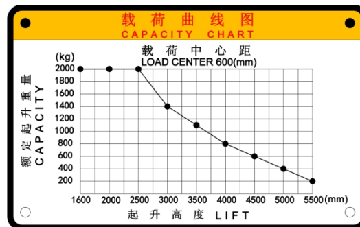
图 3-6-1 载荷曲线图 (三级门架)
