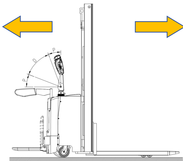
图 8-2 行驶示意图
