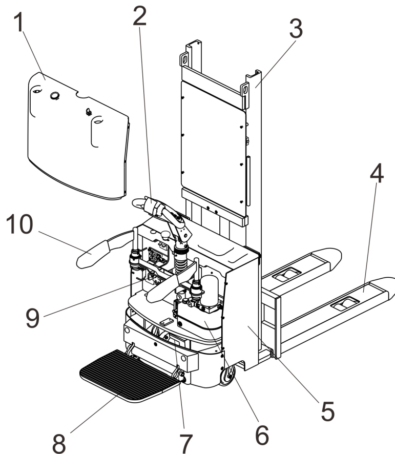
图 3-1 主体分类
