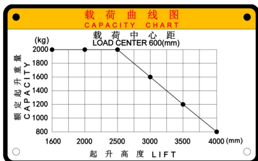
图 3-6-1 载荷曲线图
