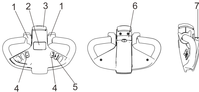
图 7-2 操作手柄
