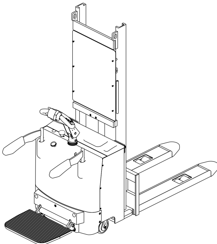
图 1-1 CL20 电动托盘堆垛车
