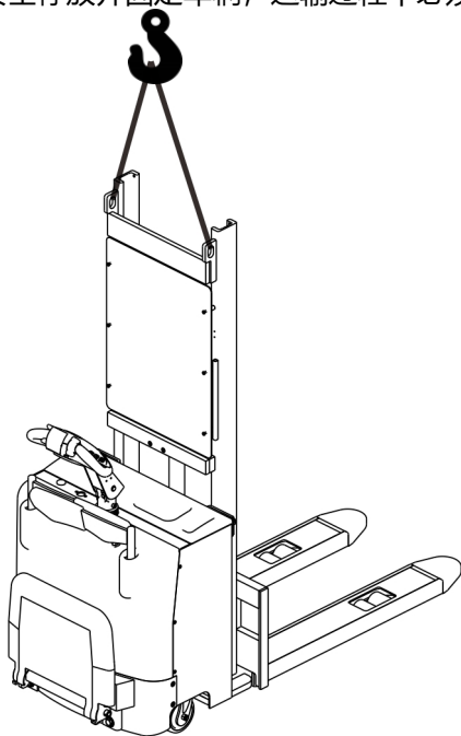
图 5-2-1 起吊
