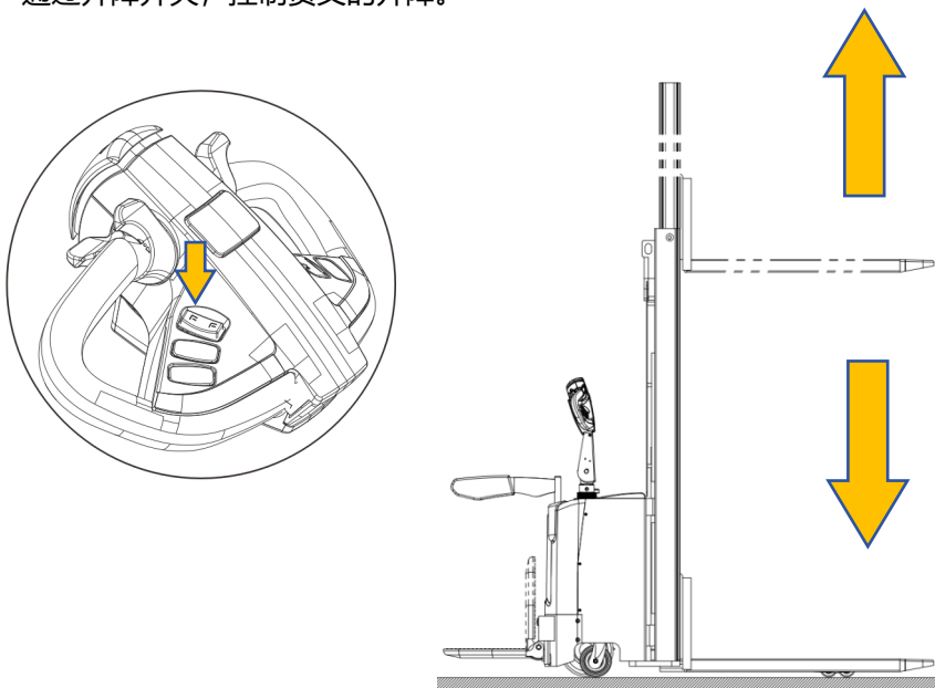
图 8-7 起升示意图
