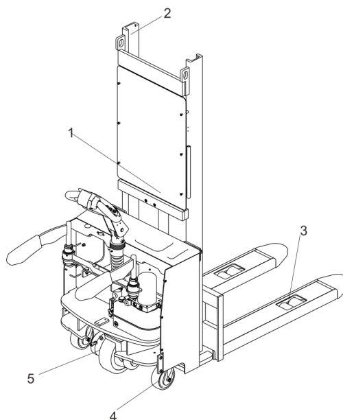
图 13-2 润滑点
