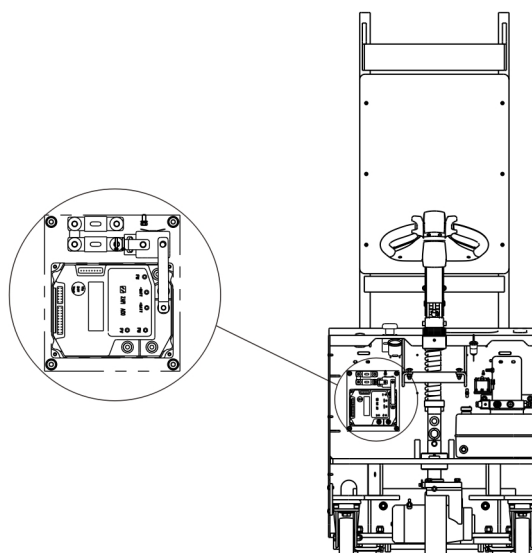
图 13-3 保险丝位置
