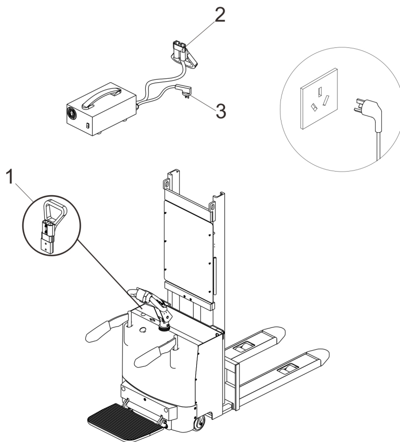
图 10-2-1 充电示意图
