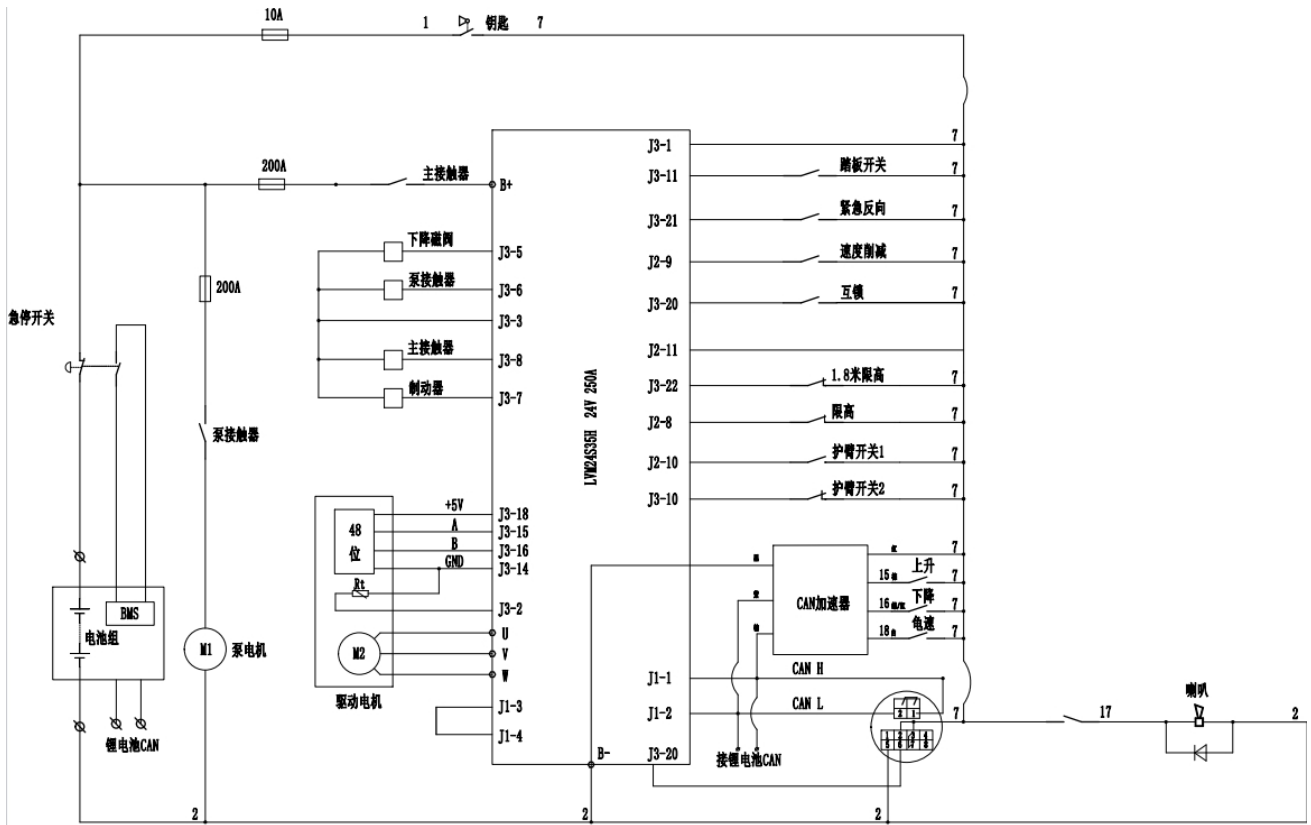
图 15-3 电气原理图（前拓控制器）
