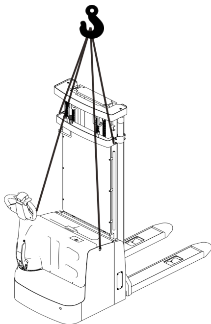
图 5-2-1 起吊
