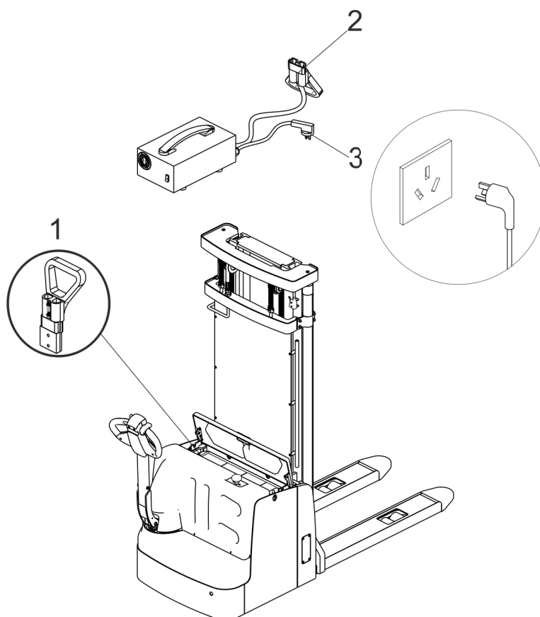
图 10-2 充电示意图
