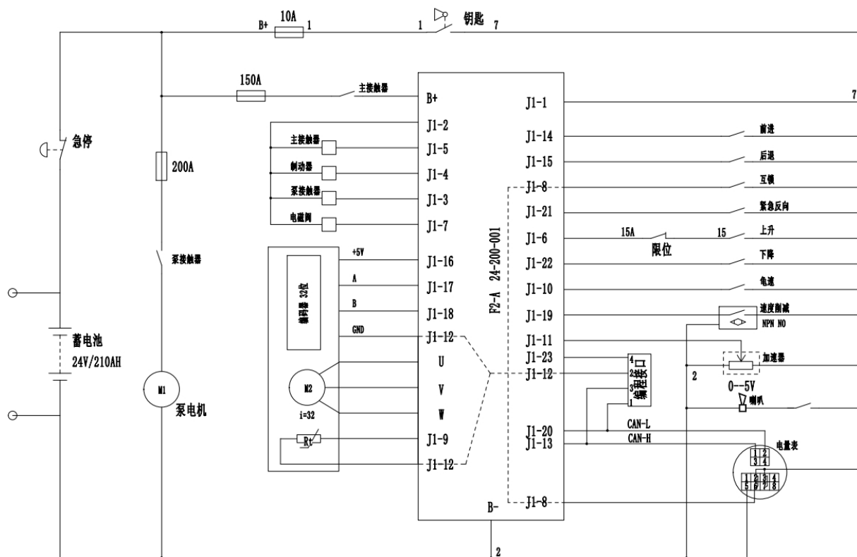
图 15-1 电气原理图 (F2-A)
