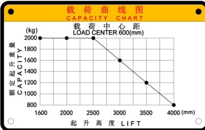
图 3-6-2 载荷曲线图 (2t)
