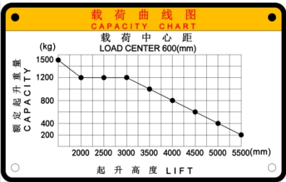
图 3-6-1 载荷曲线图 (1.5t)
