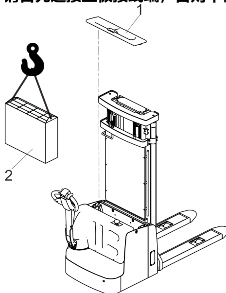
图 10-1 电池更换示意图
