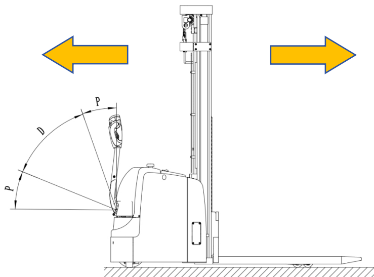
图 8-2 行驶示意图
