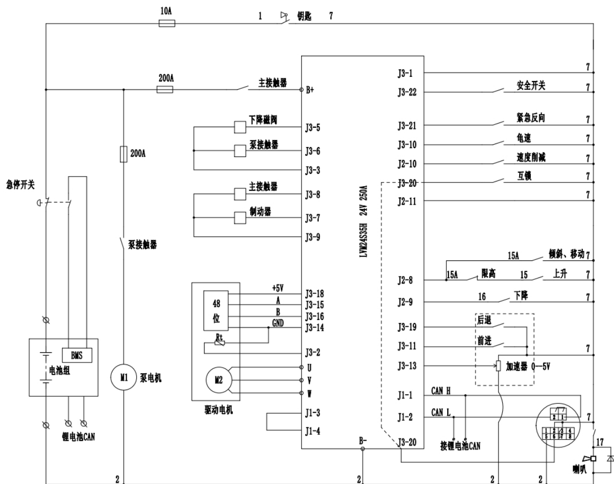
图 15-1 电气原理图（国产控制器）
