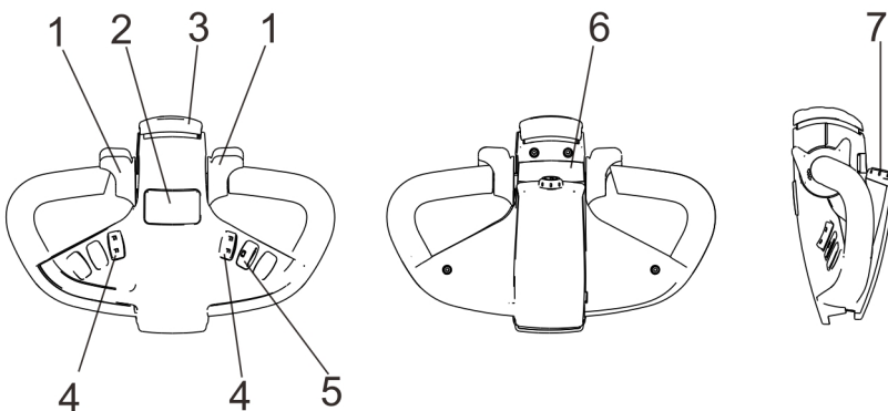
图 7-2 操作手柄
