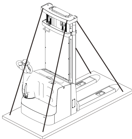
图 5-2-2 固定点
