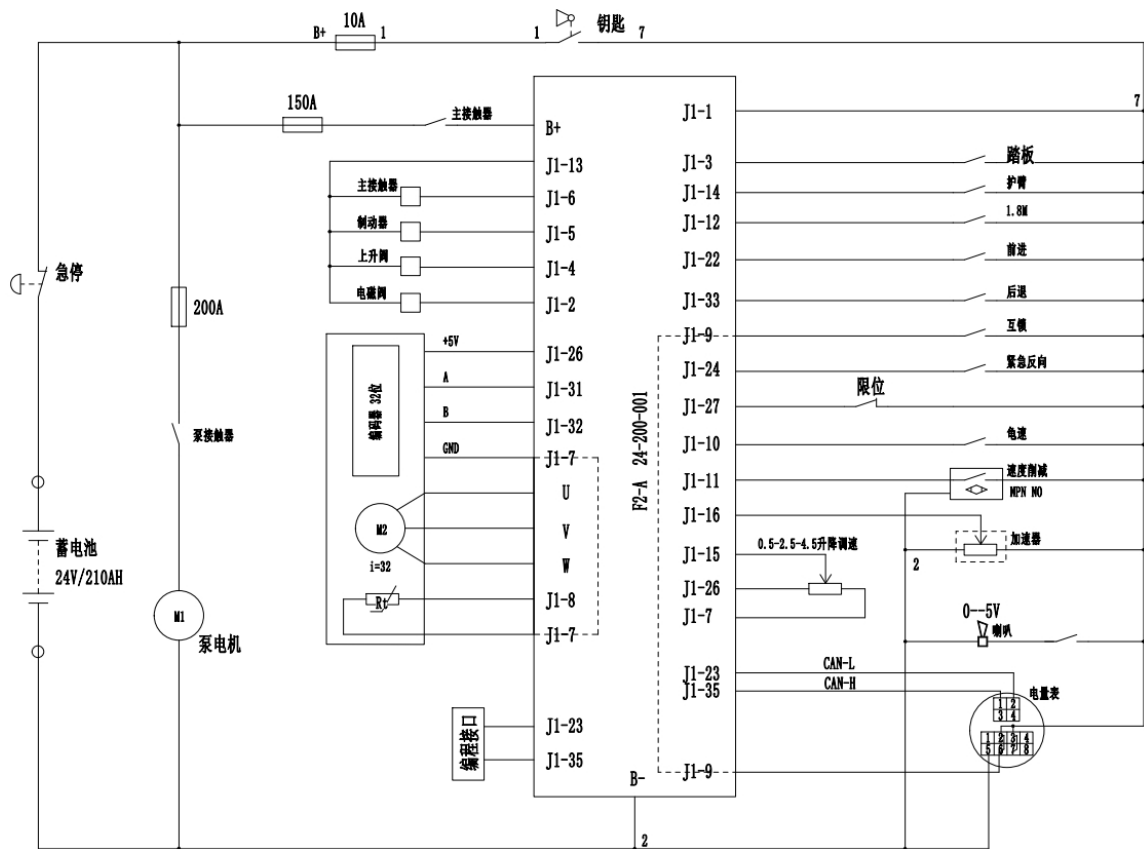
图 15-2 电气原理图 (F2-C)
