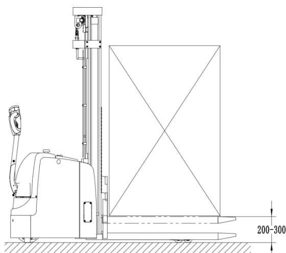
图 9-3 大体积物料
