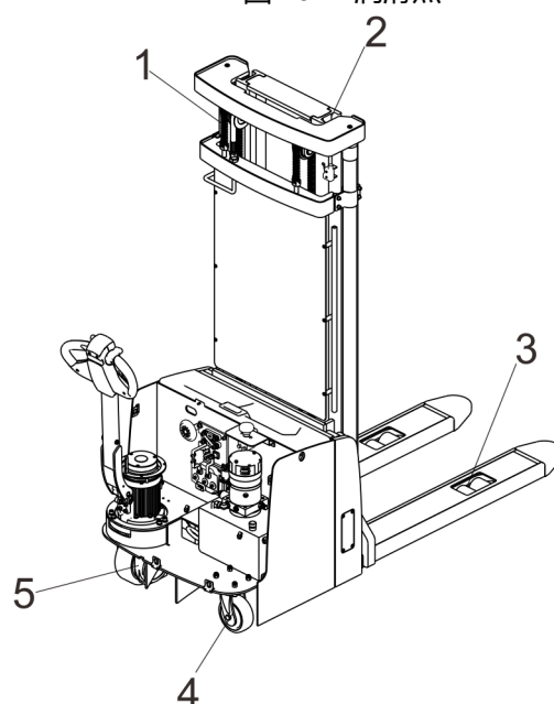
图 13-2 润滑点
