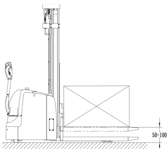
图 9-2 小体积物料
