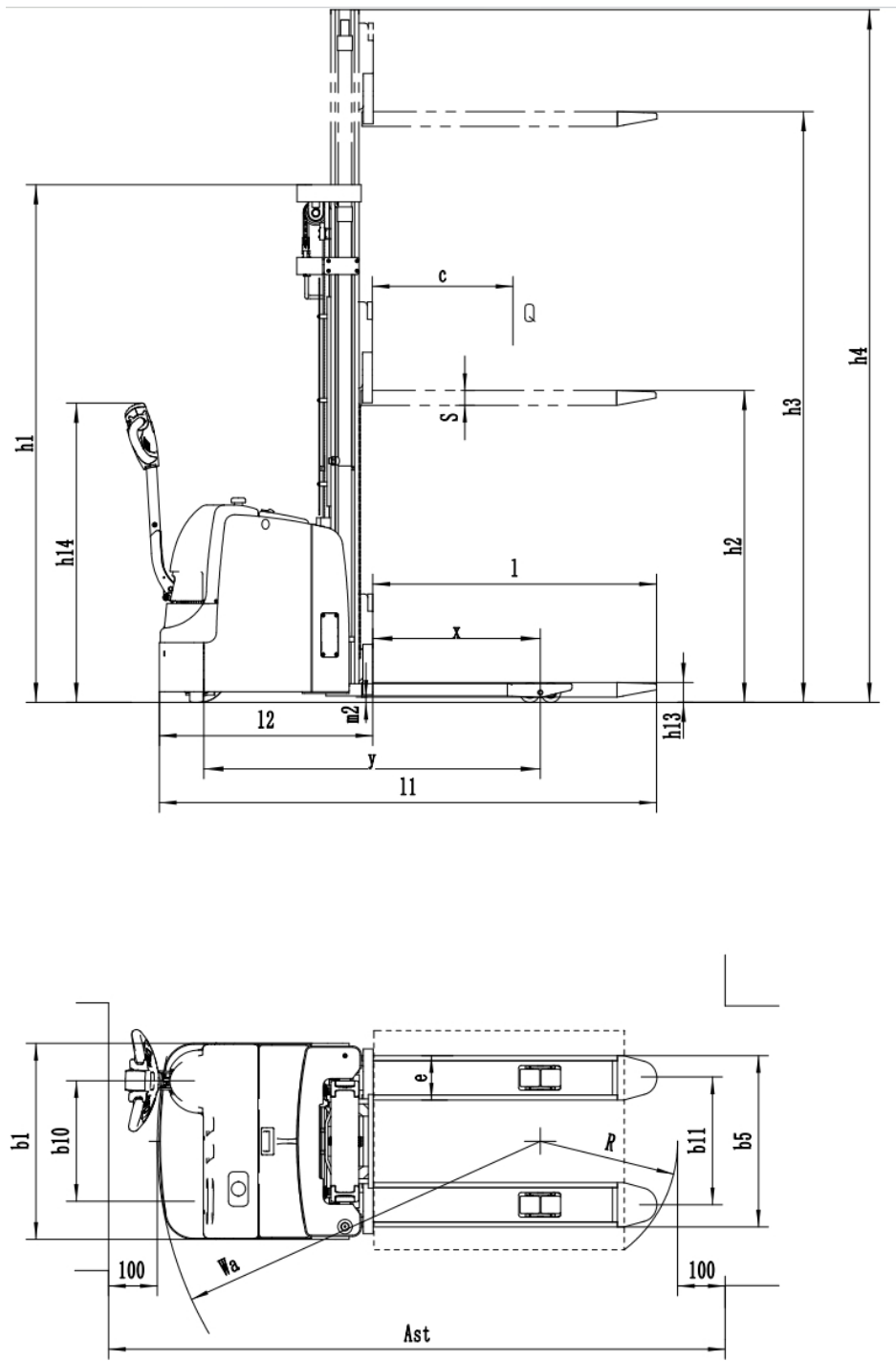
图 3-2 技术参数图
