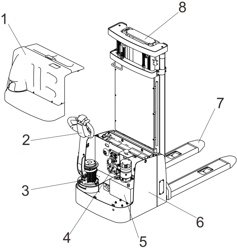
图 3-1 主体分类
