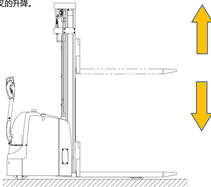
图 8-7 起升示意图
