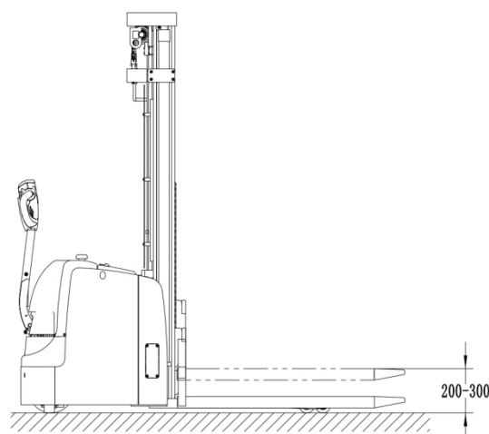
图 9-1 货叉离地 200mm-300mm
