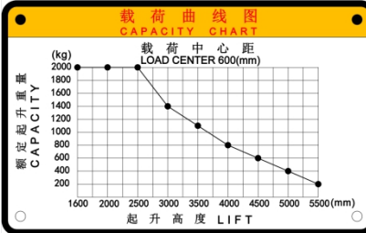
图 3-6-3 载荷曲线图 (2t 三级全自由)
