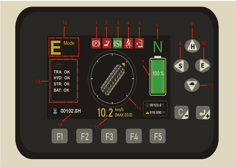
图 13-4 显示屏区域
