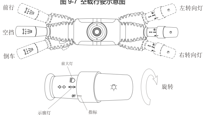
图 9-8 组合开关
