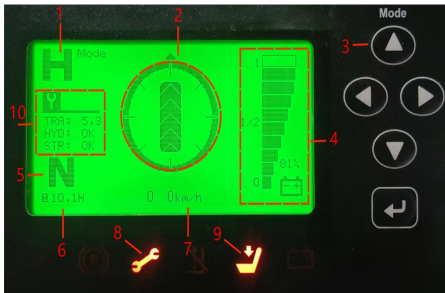
图 13-1 显示屏区域
