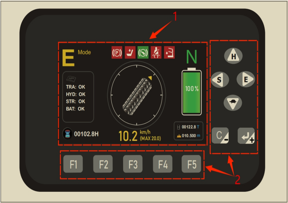
图 13-2 柯蒂斯仪表（F4-A 控制器）
