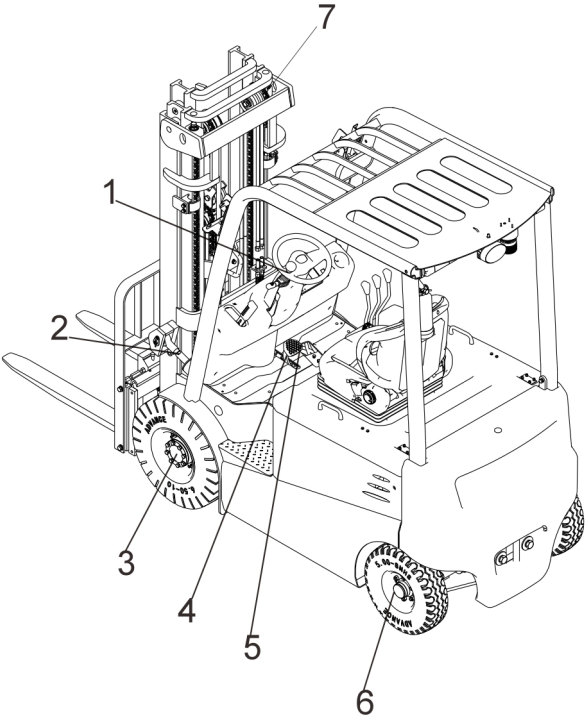
图 14-1 润滑点
