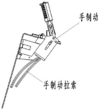
图 9-17 停车制动装置
