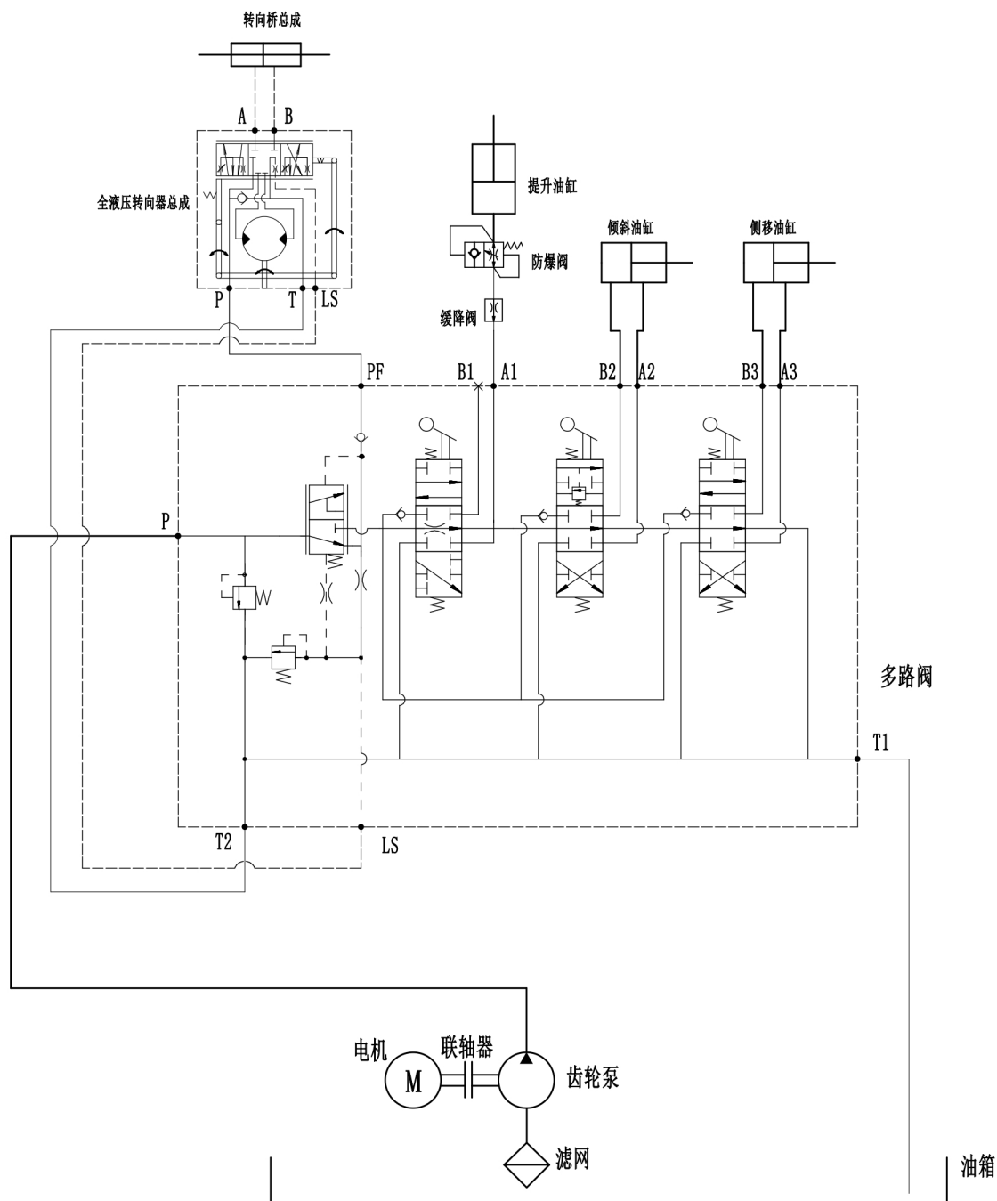
图 17-1 液压原理图
