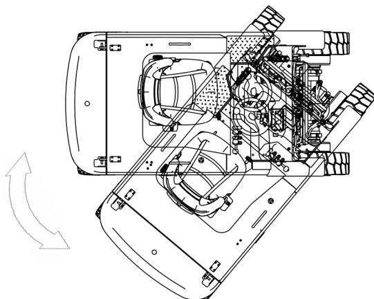
图 9-11 转弯轨迹示意图
