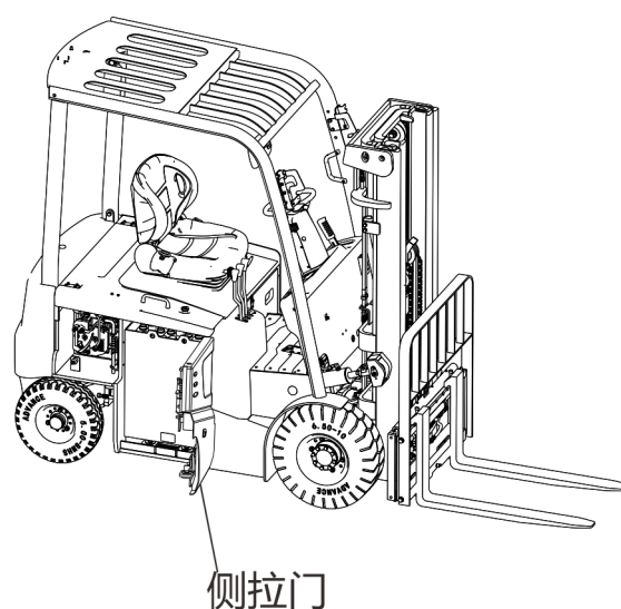
图 11-1 电池更换示意图
