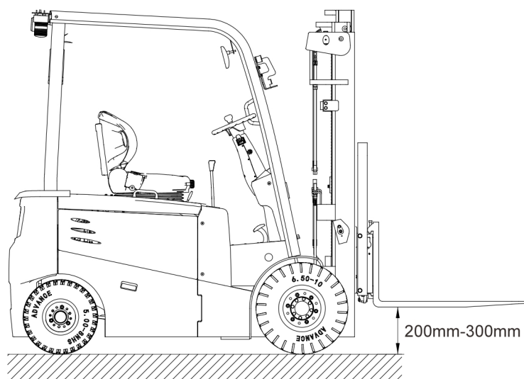
图 9-7 空载行驶示意图
