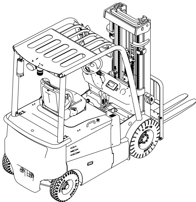
图 1-1 EA20-B 电动平衡重式叉车
