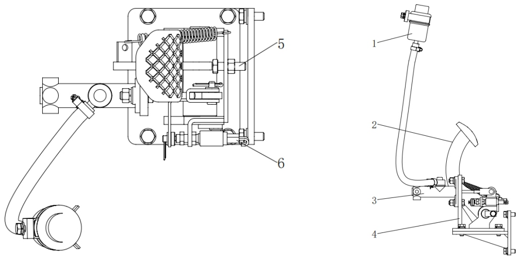
图 9-15 制动踏板示意图
