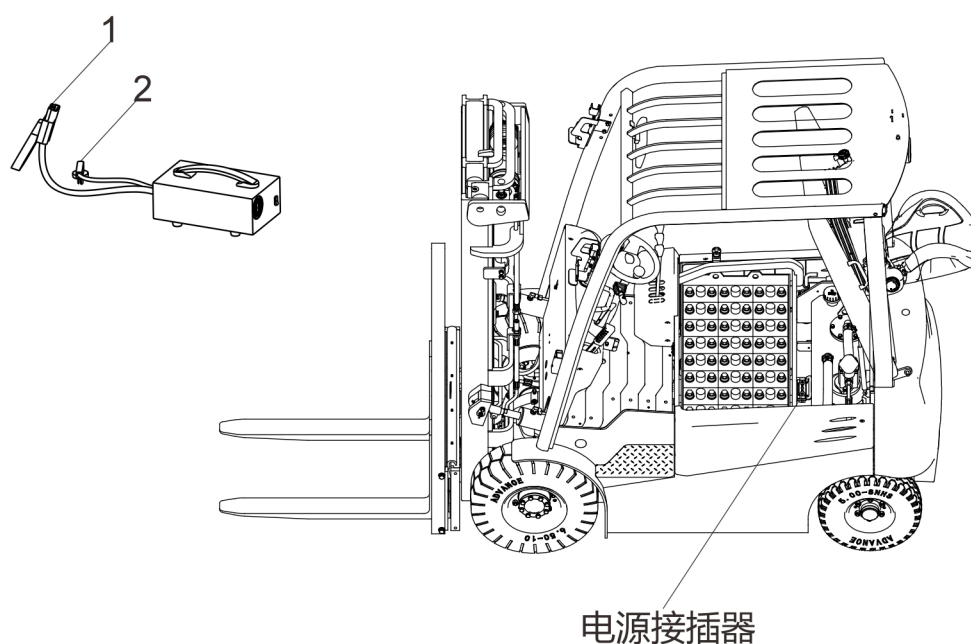
图 11-2 充电口位置示意图
