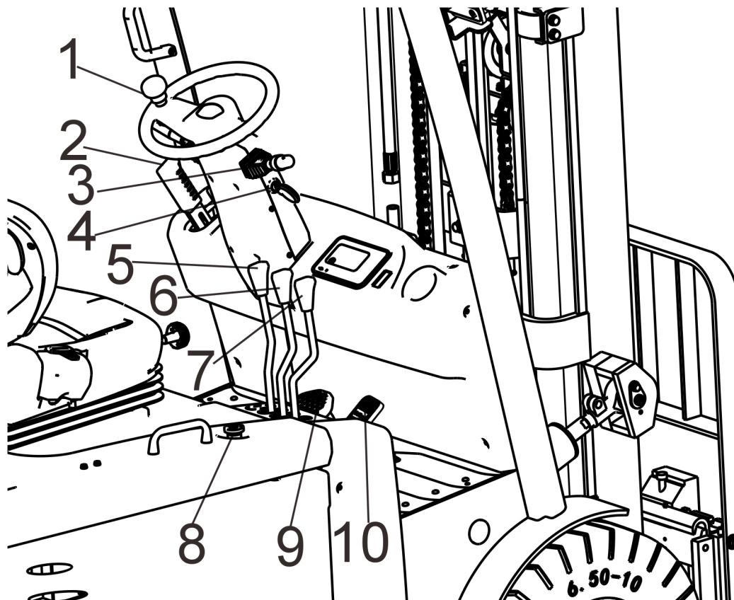
图 8-1 操作控制台
