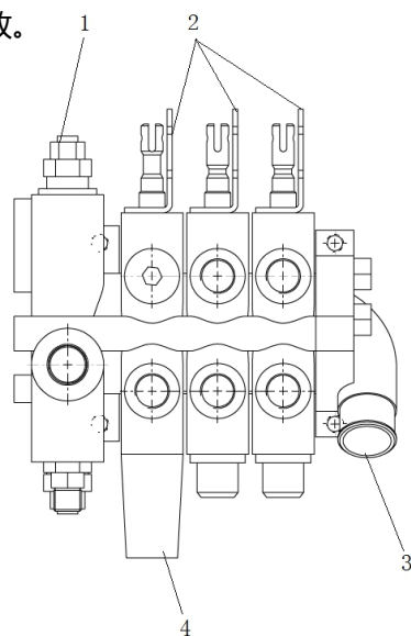
图 5-1 多路阀外形
