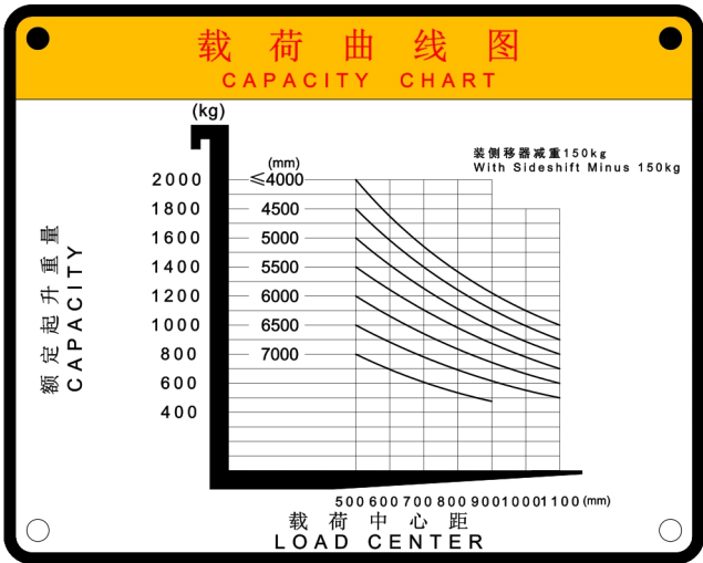
图 6 载荷曲线示意图
