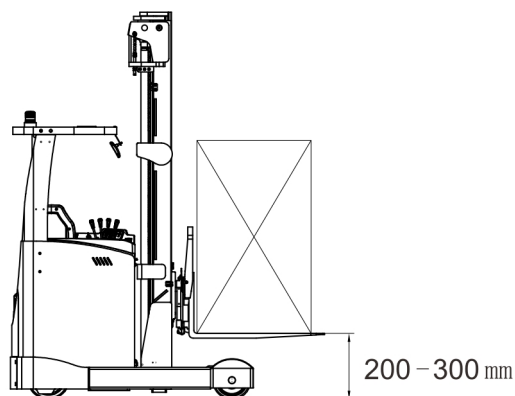
图 26 大体积物料 200-300mm
