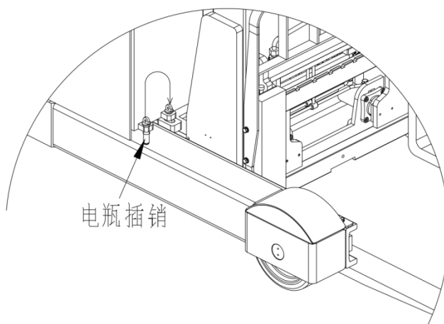
图 27 电池更换示意图
