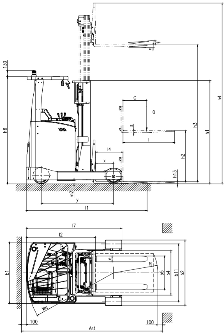
图 3 技术参数图
