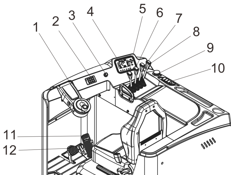
图 9 操作控制台
