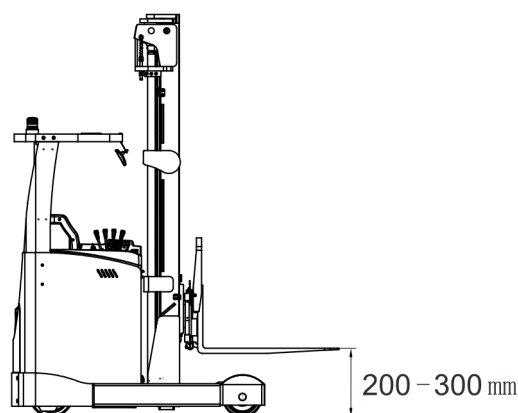
图 24 货叉离地 200mm-300mm
