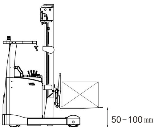
图 25 货物提升 50mm—100mm
