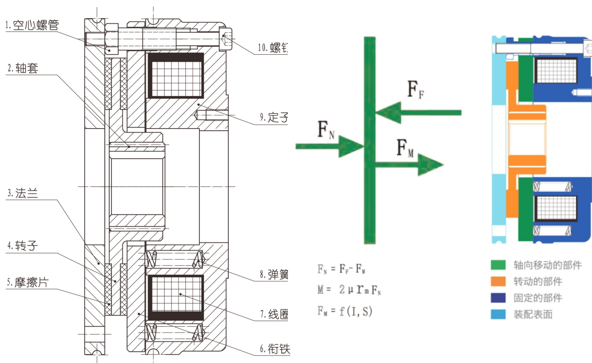
图 15 制动原理图
