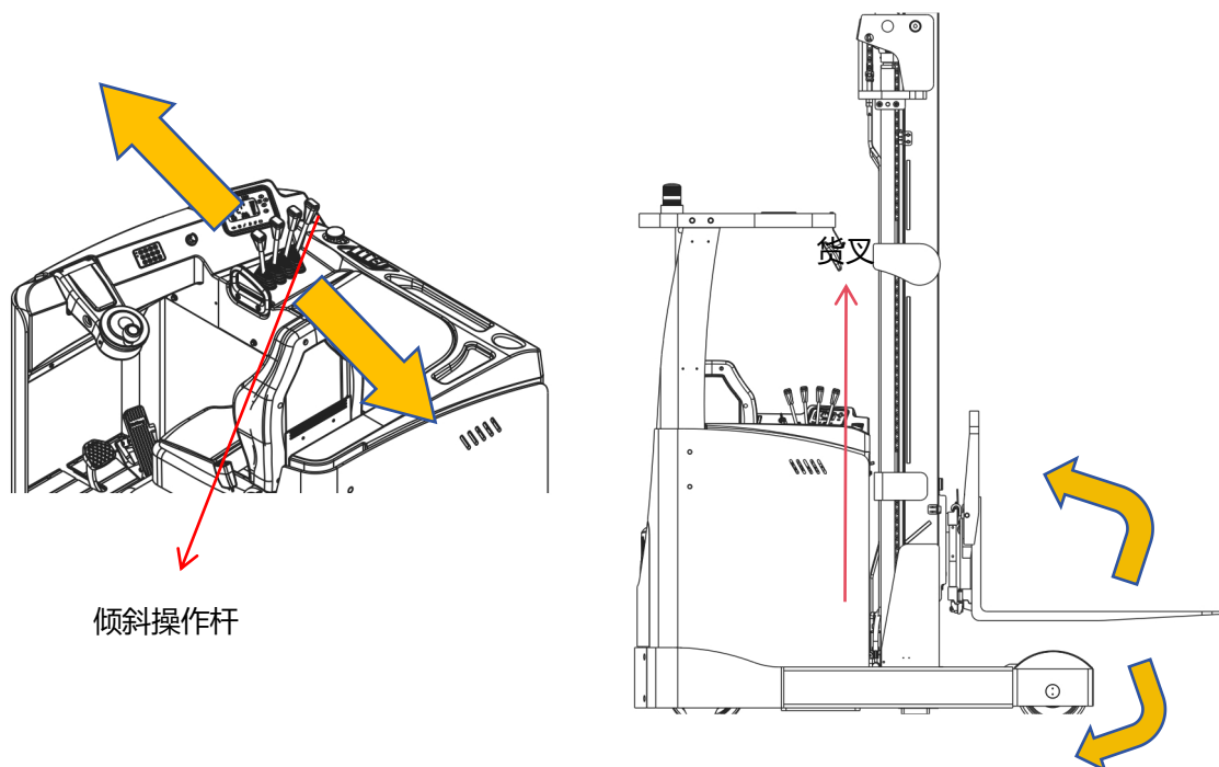
图 22 货叉前后倾斜示意图
