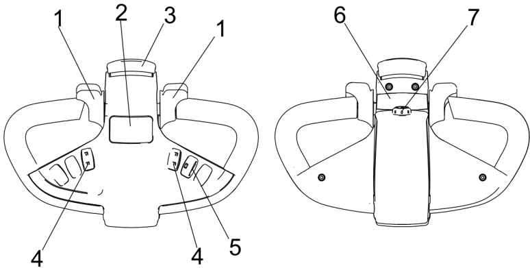
图 9 操作手柄
