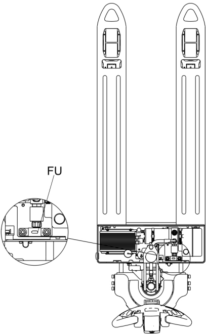
图 25 保险丝位置
