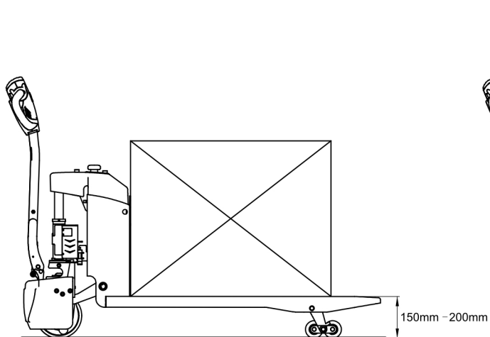
图 19 货物提升
