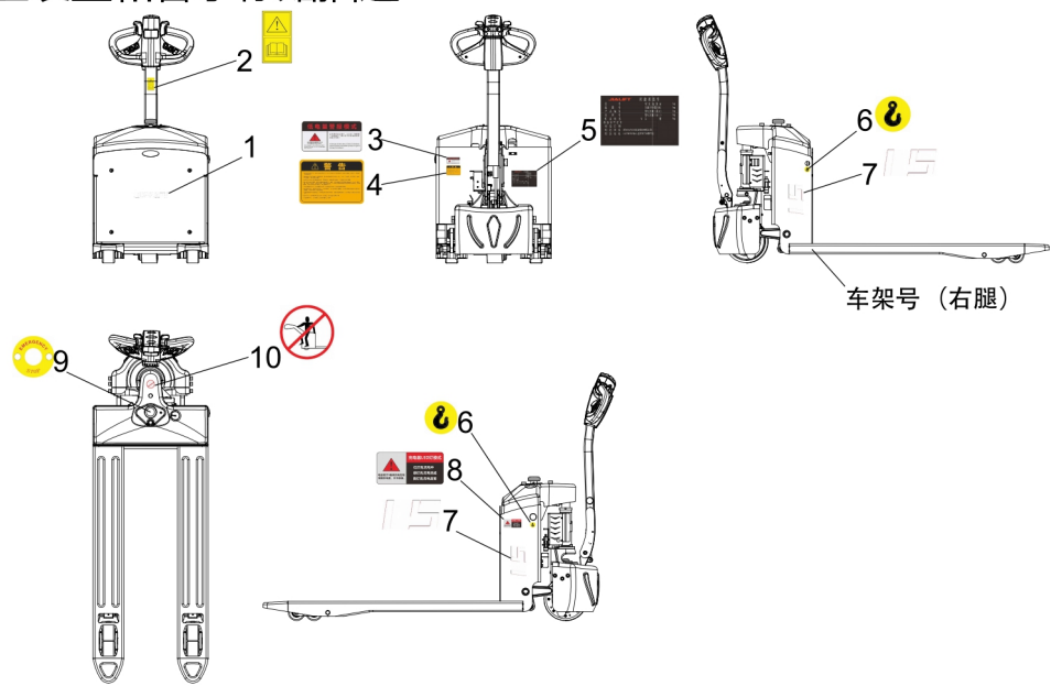
图 4 标贴描述
