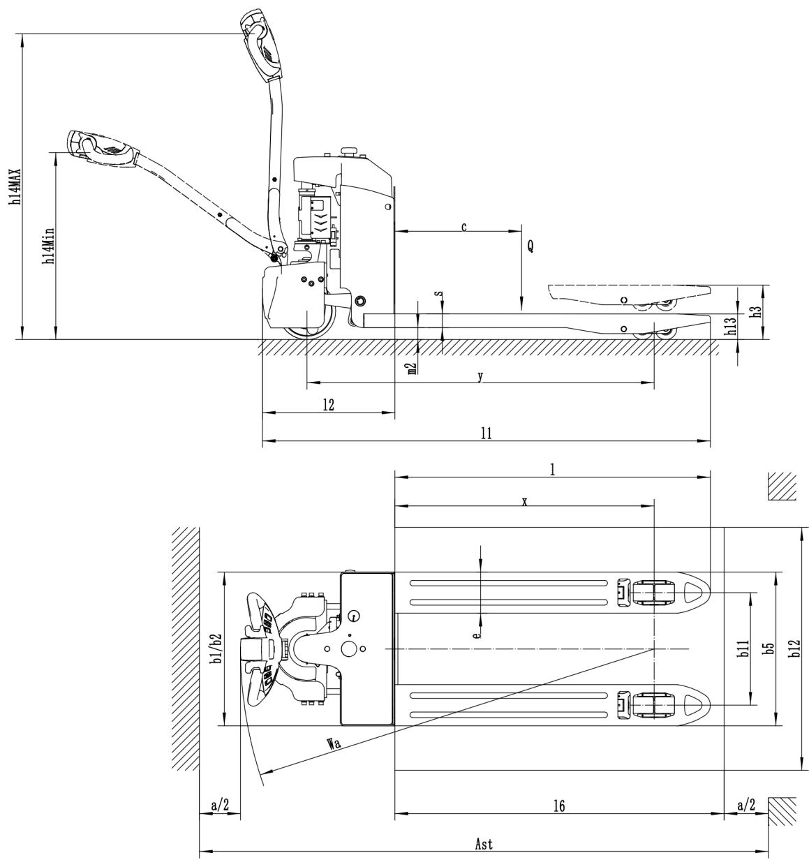
图 3 技术参数图
