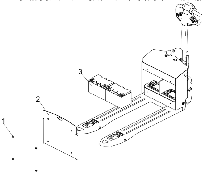
图 21 电池更换示意图
