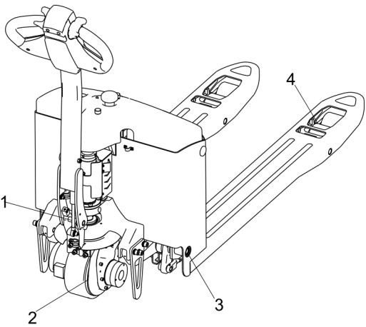
图 24 润滑点
