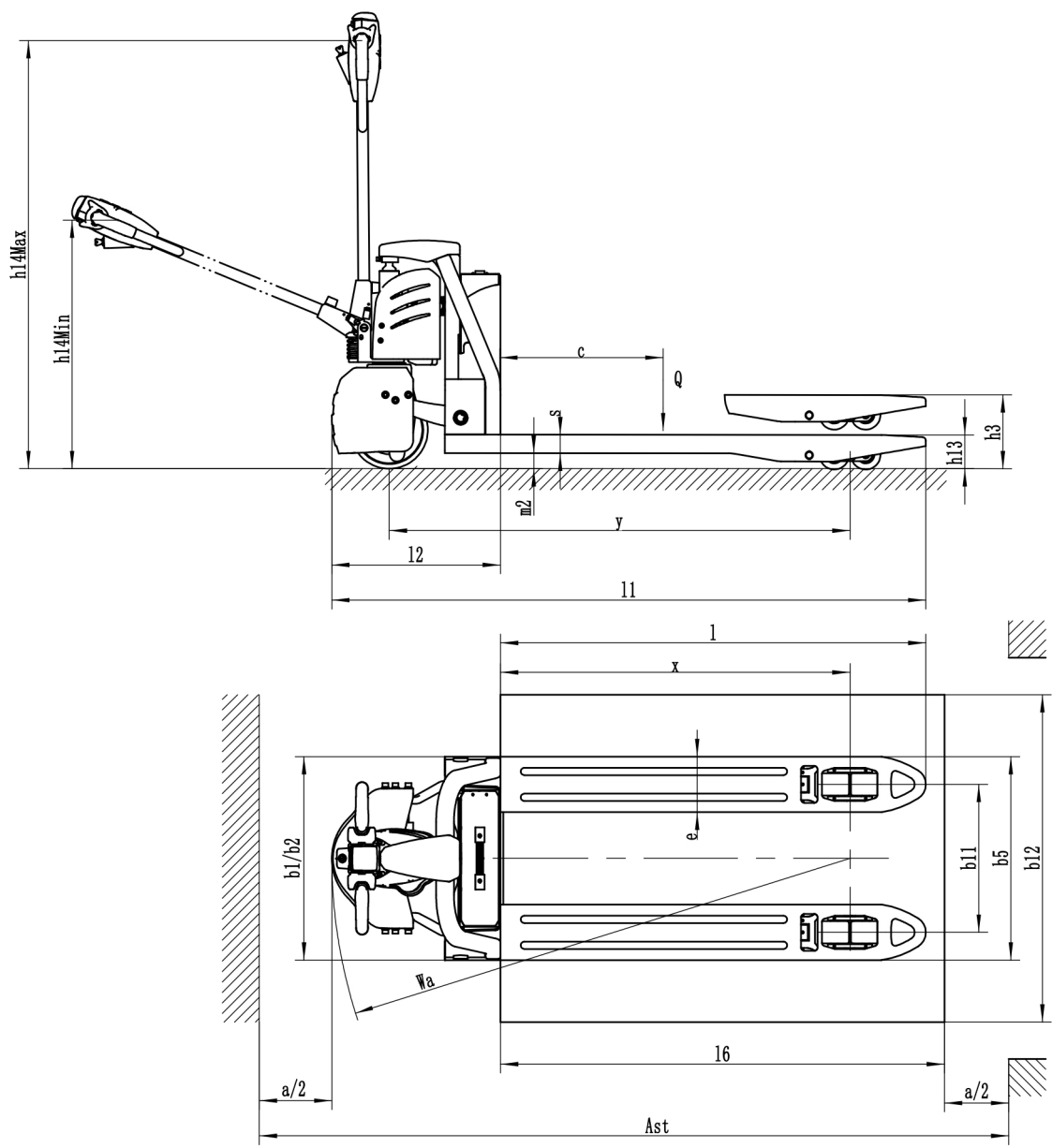
图 3 技术参数图
