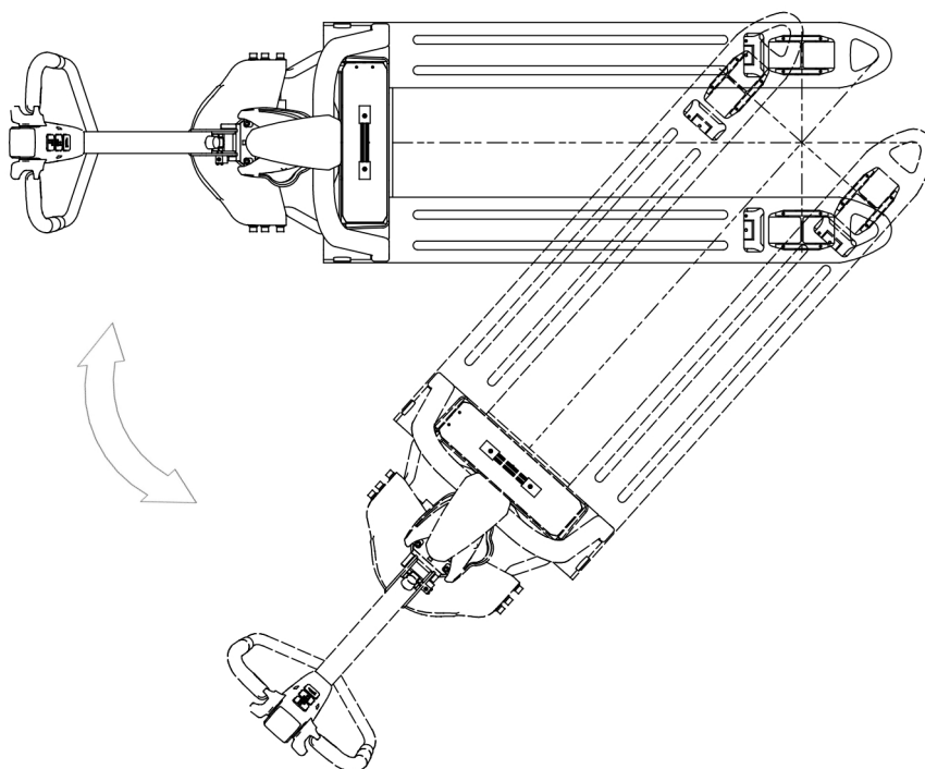
图 12 转弯轨迹示意图
