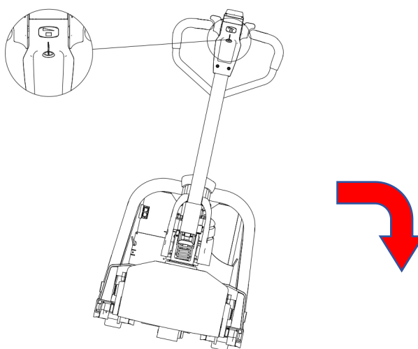
图 17 车辆倾覆
