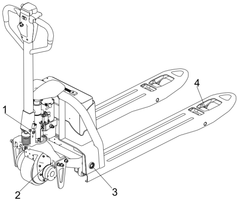
图 23 润滑点
