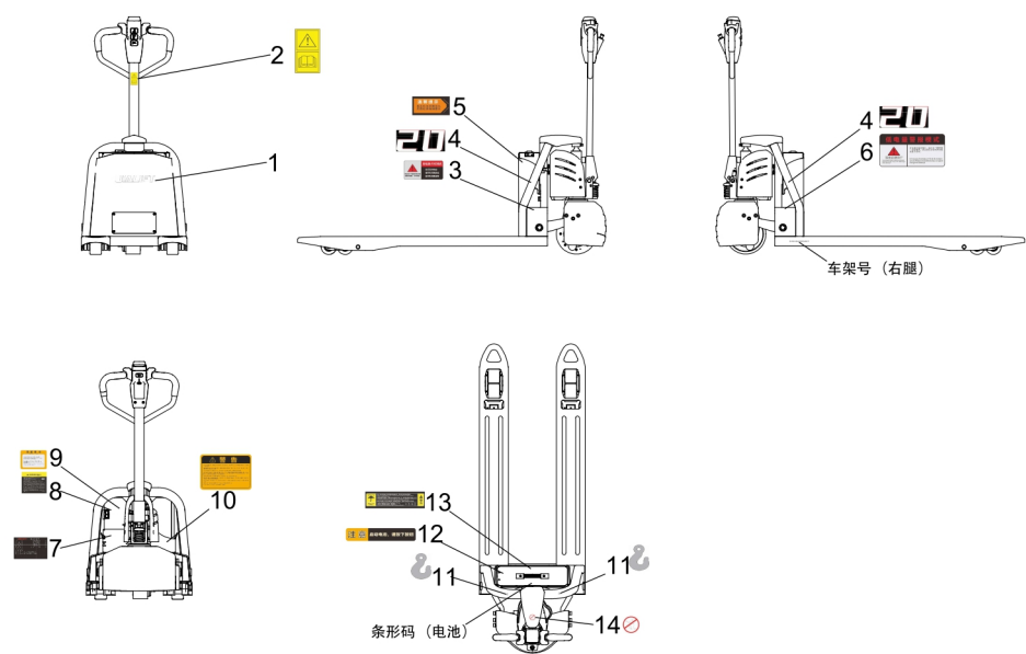
图 4 标贴描述
