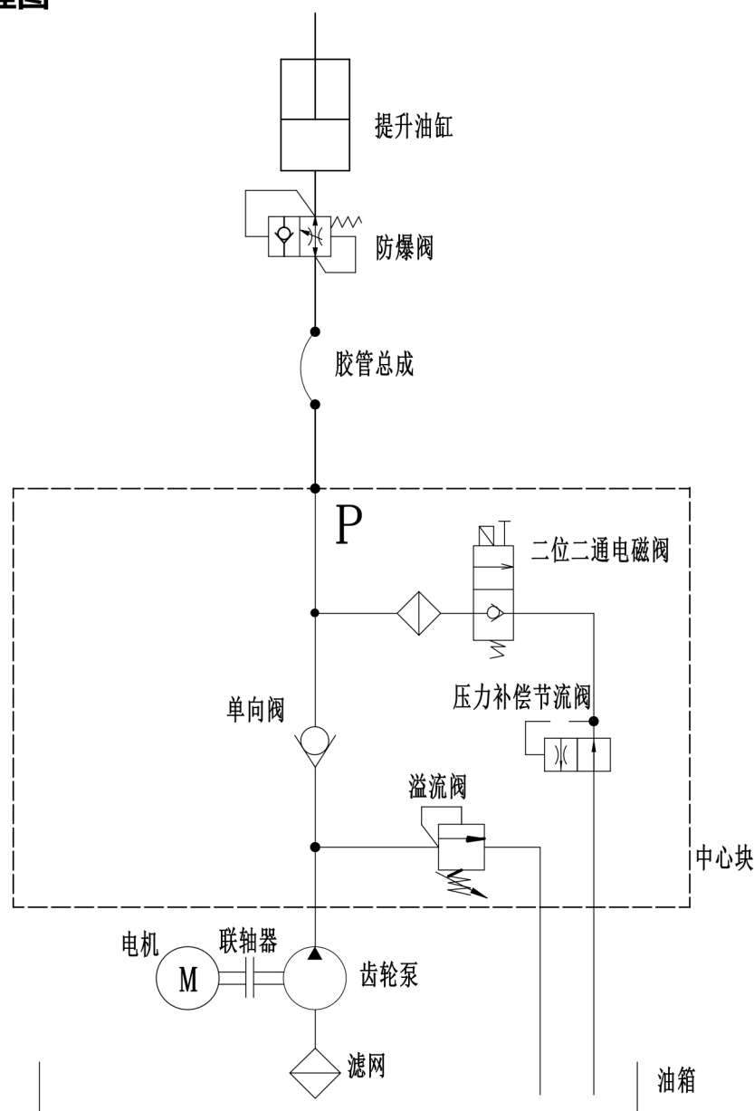
图 26 液压原理图
