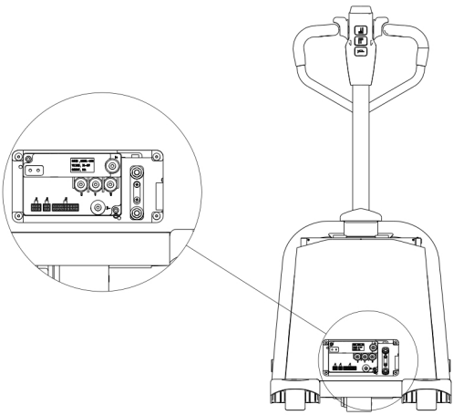
图 24 保险丝位置
