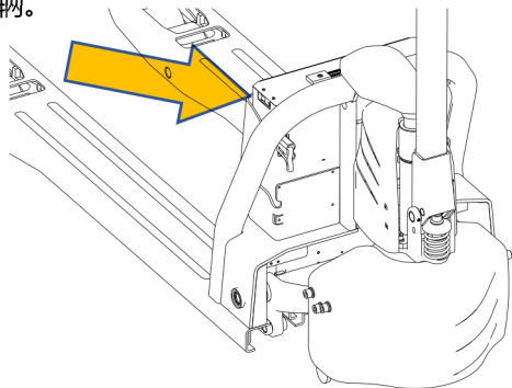
图 15 按下电池开关按钮
