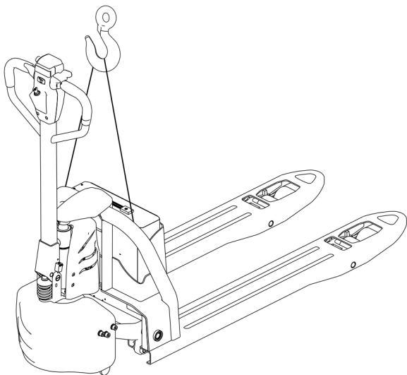
图 6 起吊
