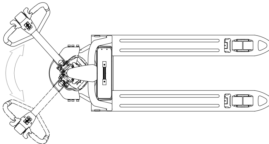
图 11 转向示意图
