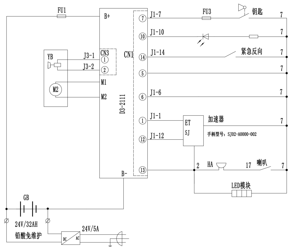
图 23 电气原理图
