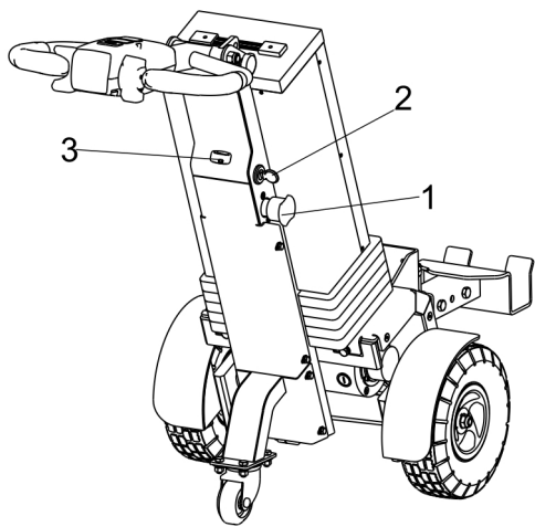
图 8 操作控制台
