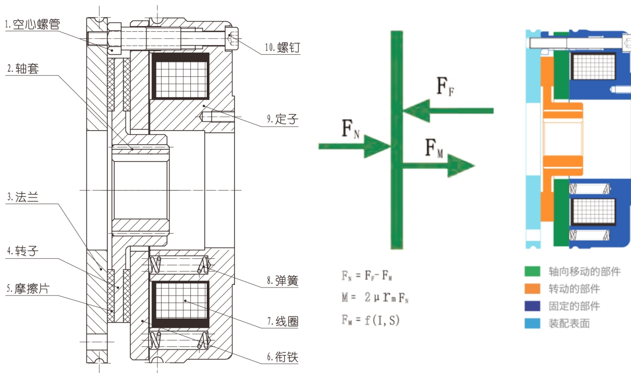
图 14 制动原理图
