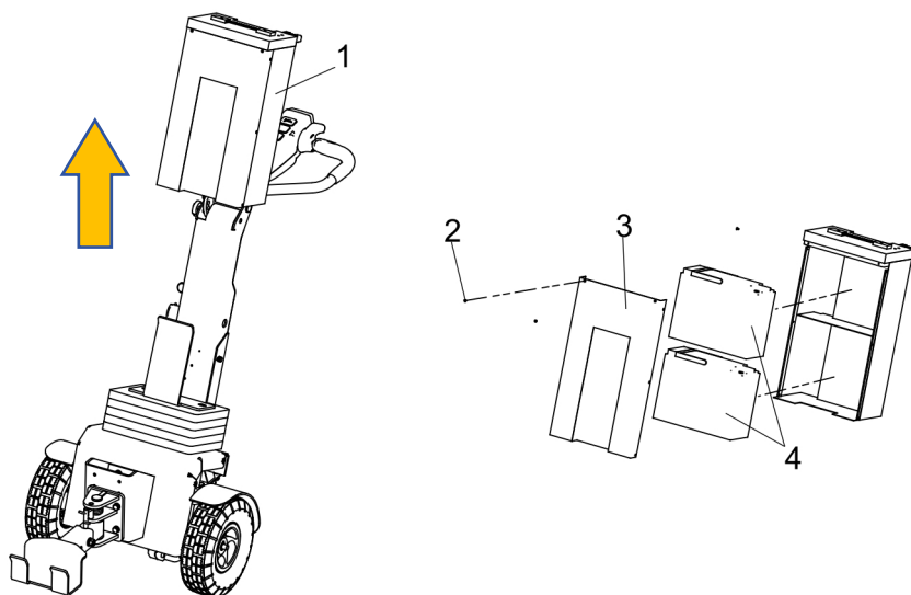
图 18 电池更换示意图
