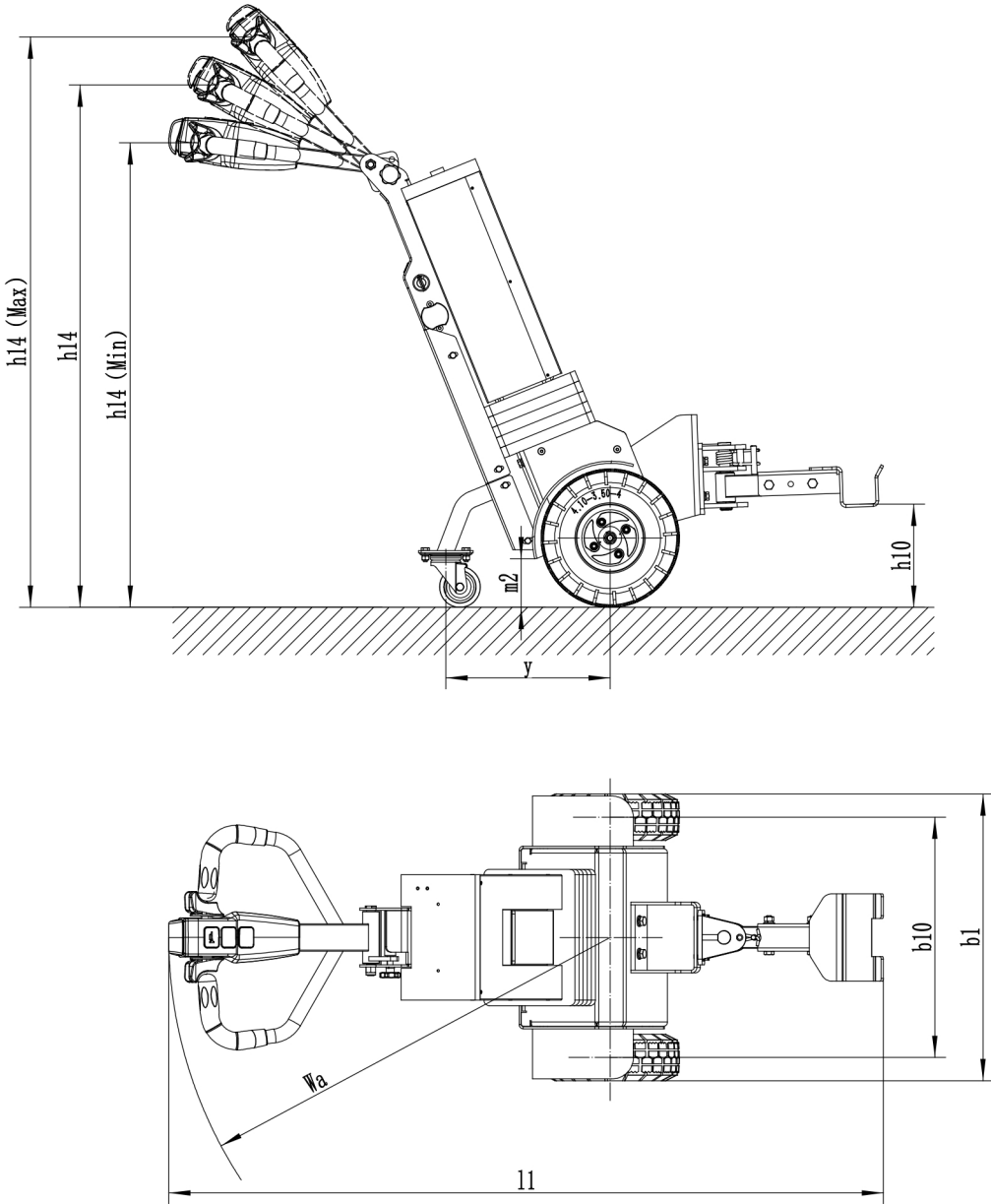
图 3 技术参数图
