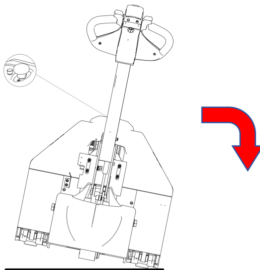
图 18 车辆倾覆
