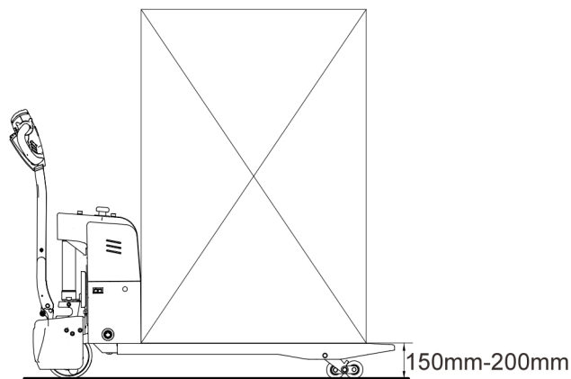
图 20 大体积物料
