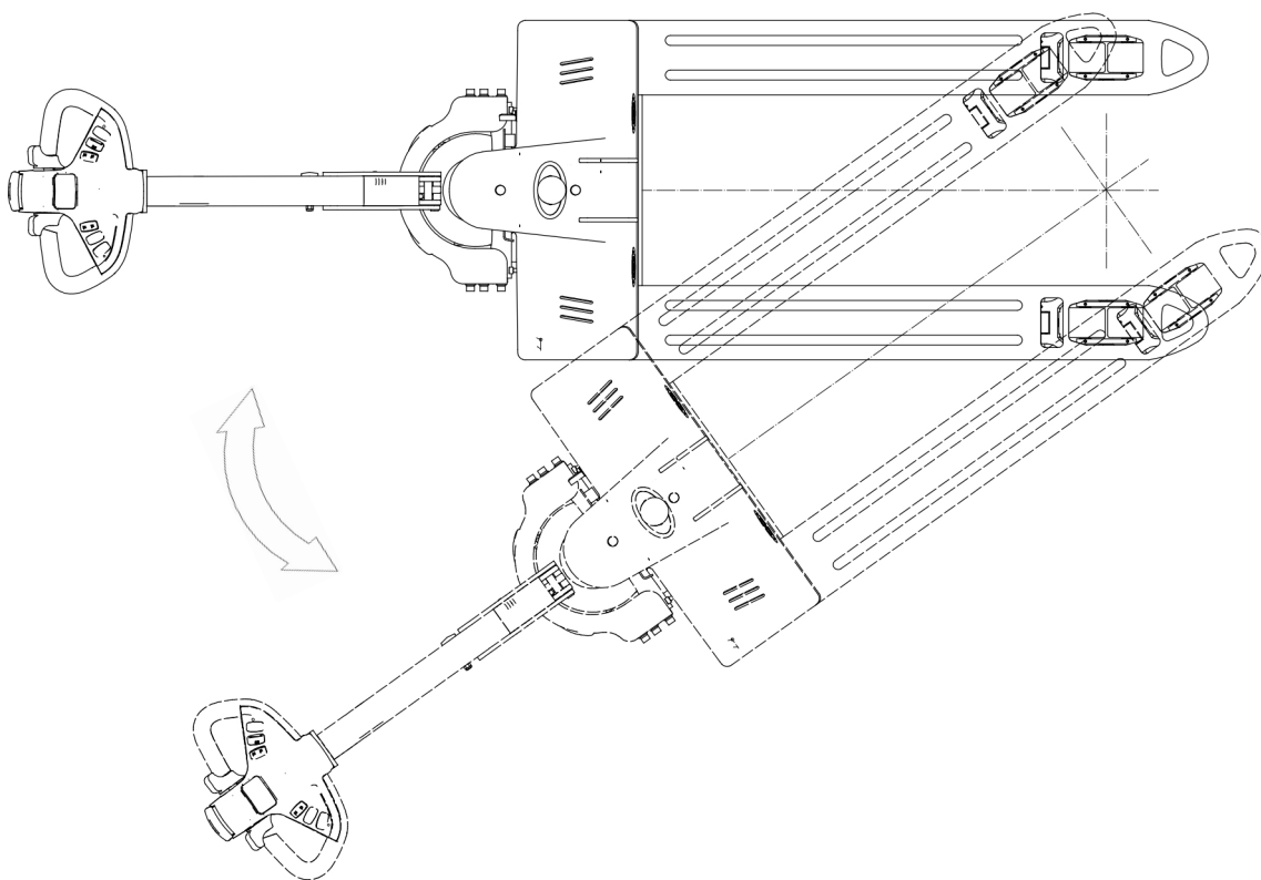
图 13 转弯轨迹示意图
