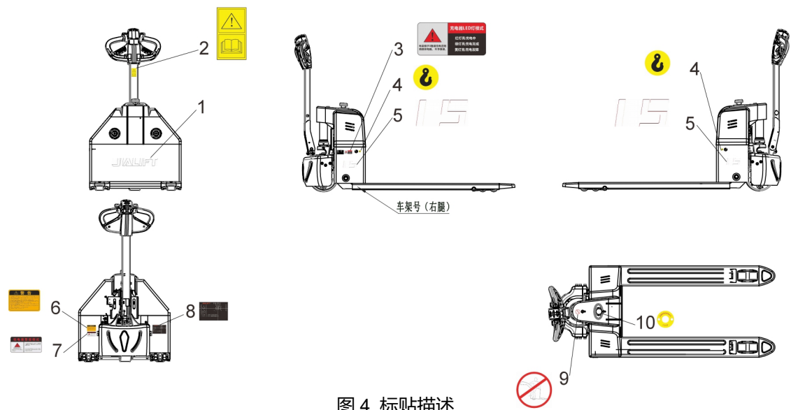
图 4 标贴描述
