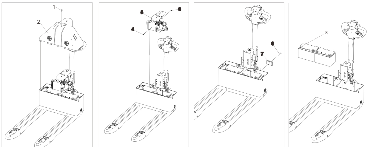
图 21 电池更换示意图
