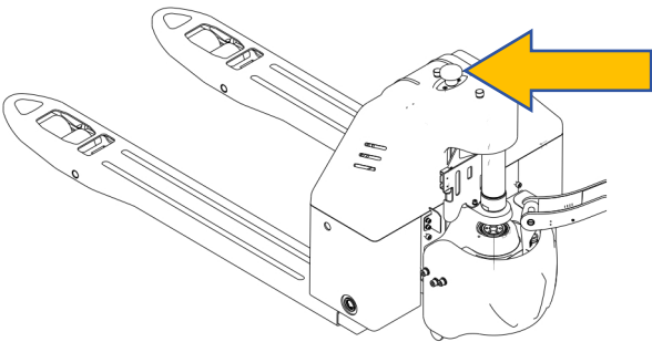
图 16 按下急停开关
