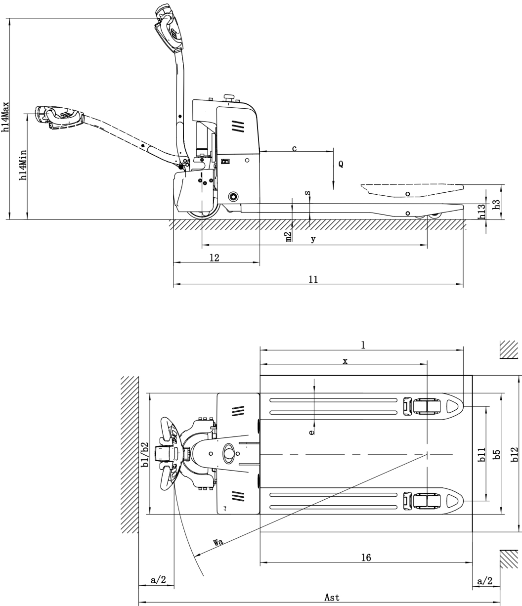
图 3 技术参数图
