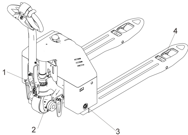
图 24 润滑点
