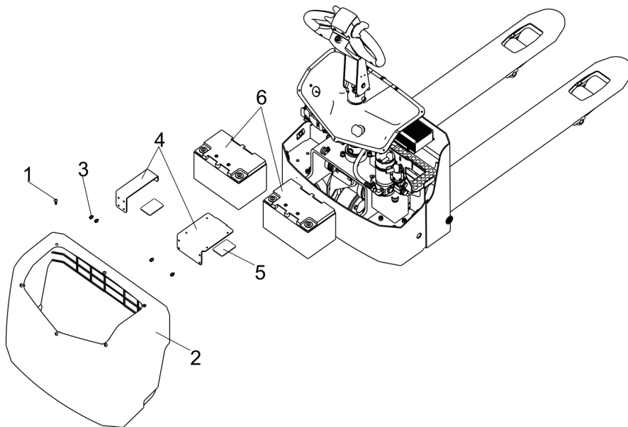
图 21 电池更换示意图
