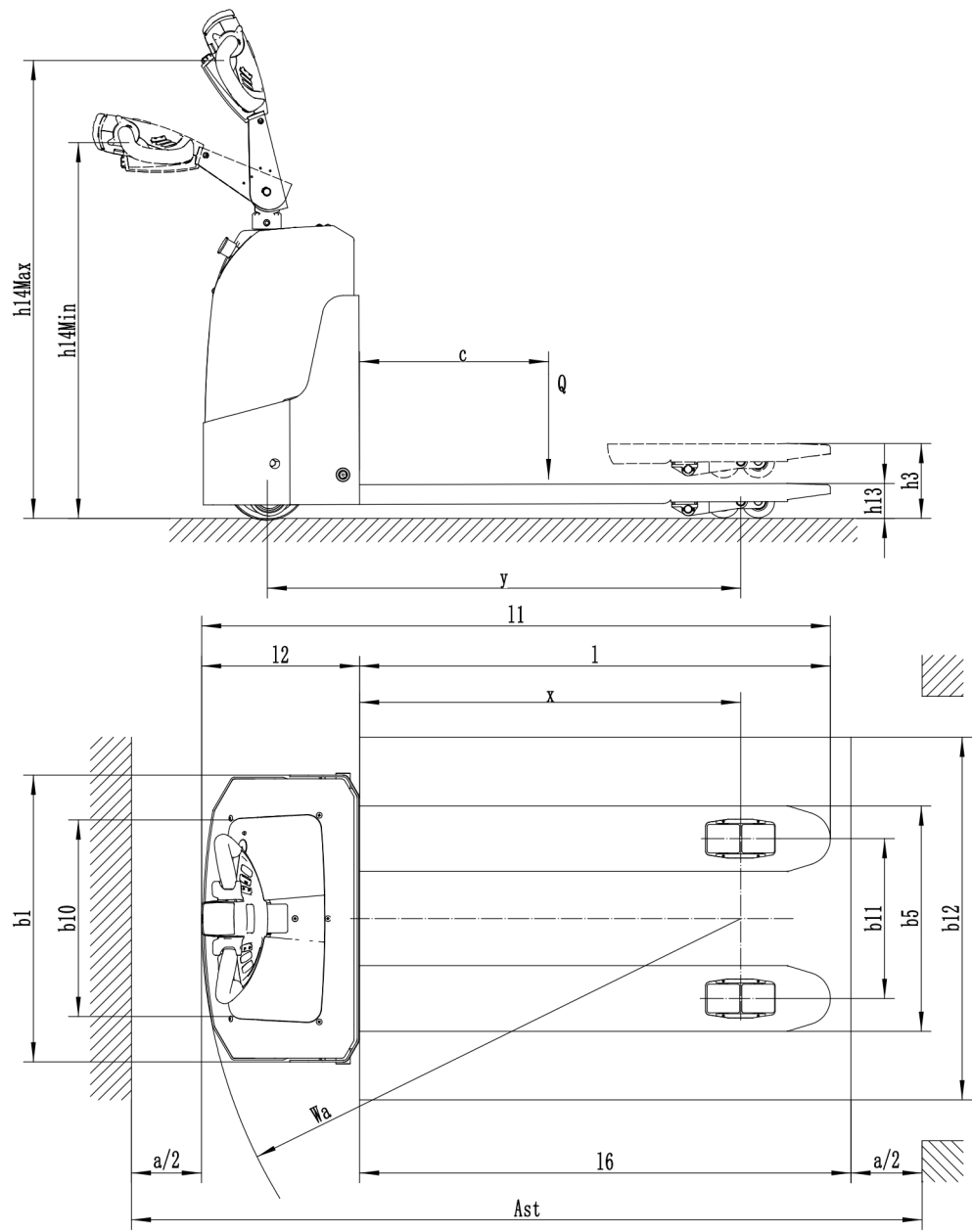
图 3 技术参数图
