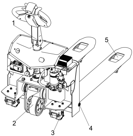
图 24 润滑点
