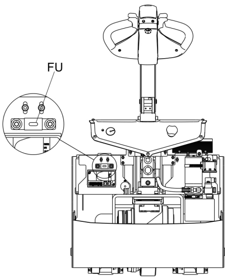
图 25 保险丝位置
