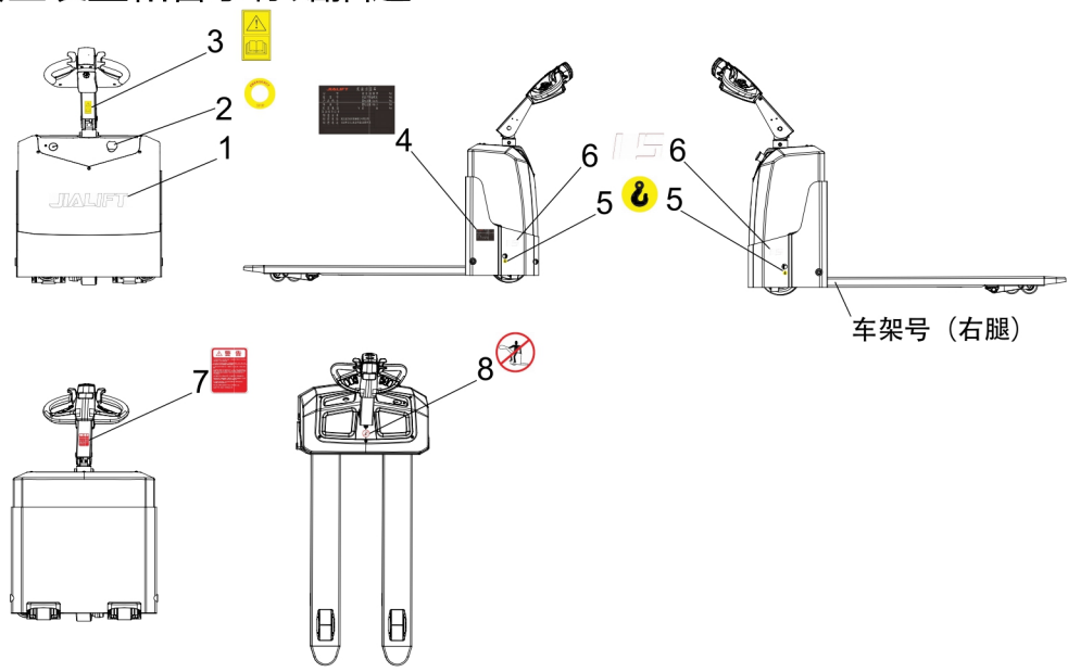
图 4 标贴描述
