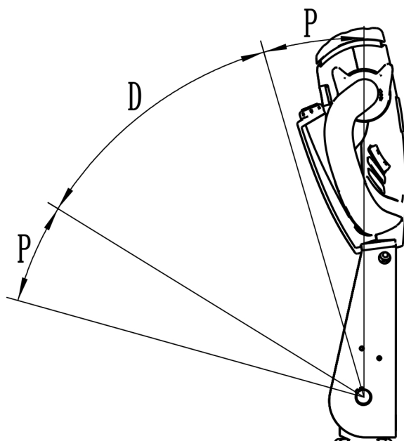
图 14 操纵杆角度
