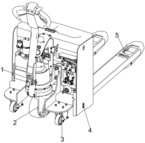
图 24 润滑点
