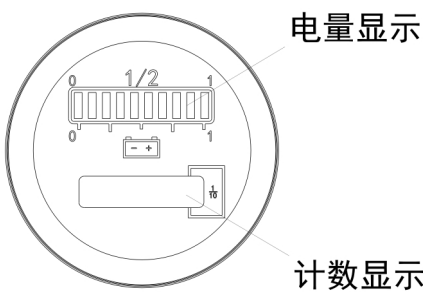
图 23 圆形电量表
