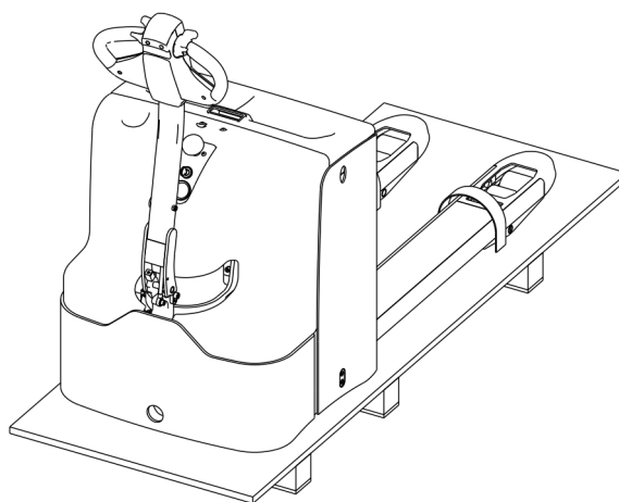
图 7 固定点
