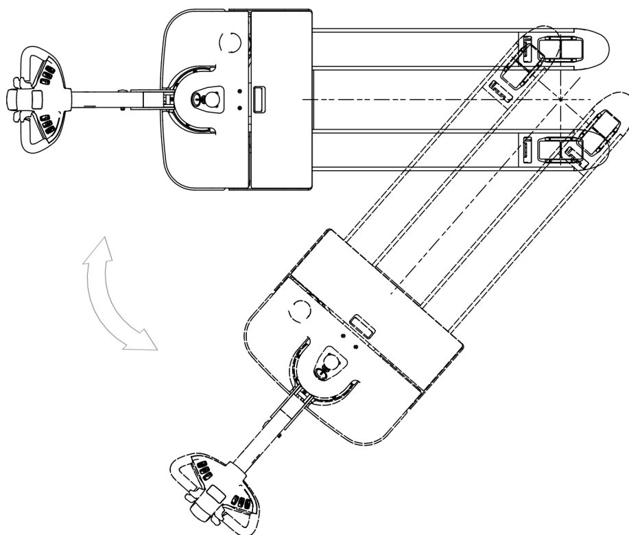
图 13 转弯轨迹示意图
