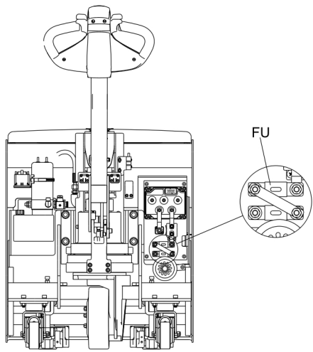
图 25 保险丝位置
