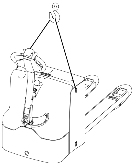
图 6 起吊
