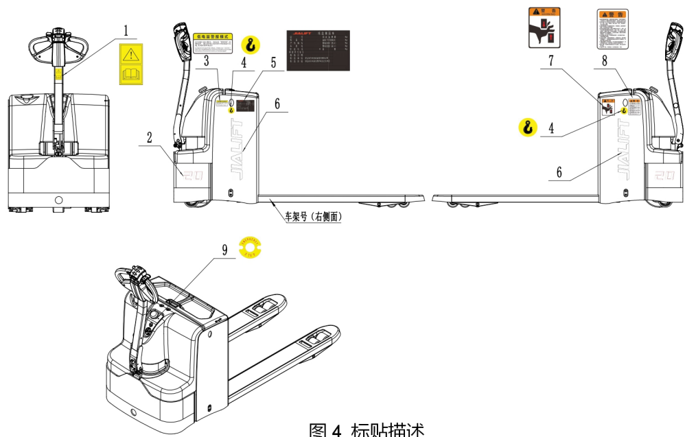
图 4 标贴描述
