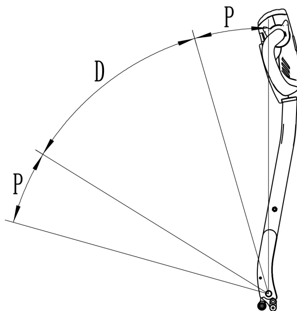
图 14 操纵杆角度
