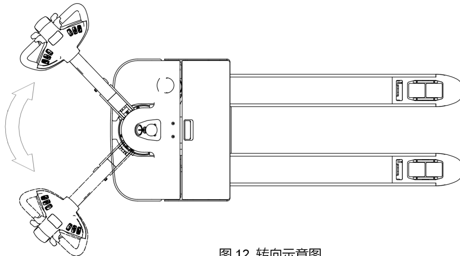
图 12 转向示意图
