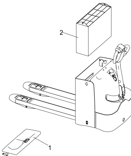
图 21 电池更换示意图
