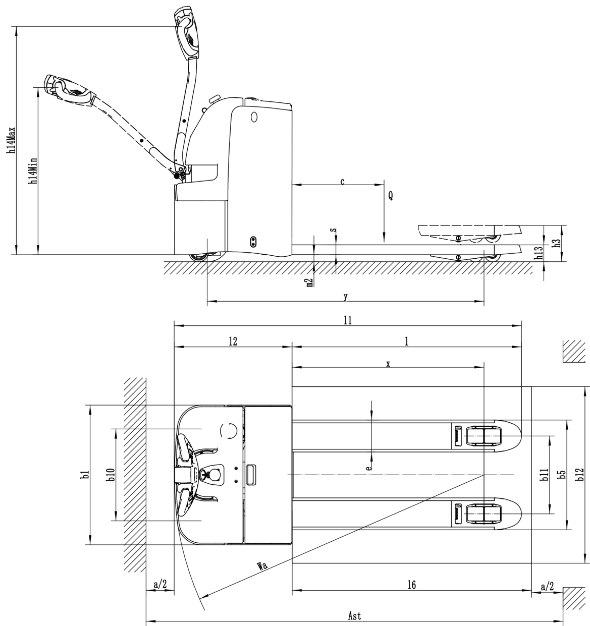
图 3 技术参数图
