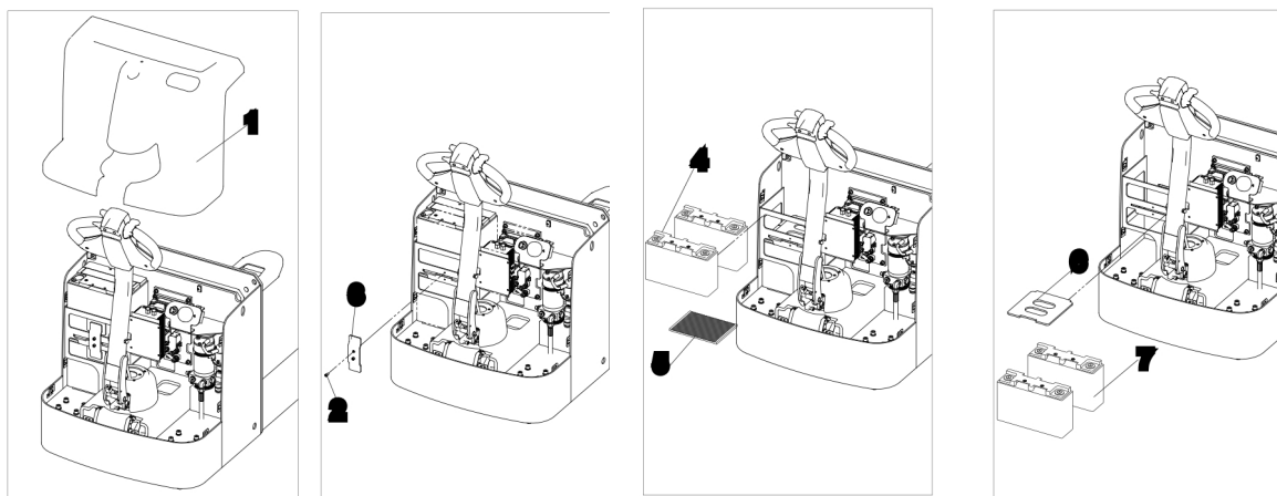
图 21 电池更换示意图
