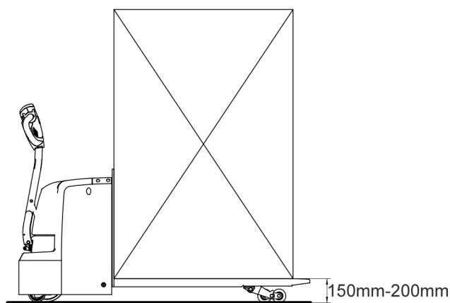
图 20 大体积物料
