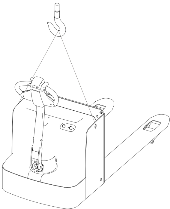
图 6 起吊
