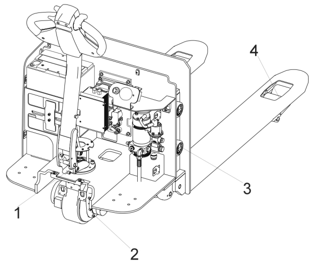
图 24 润滑点
