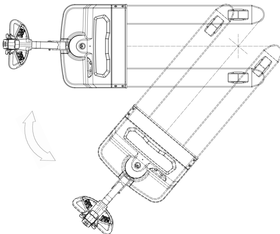
图 13 转弯轨迹示意图
