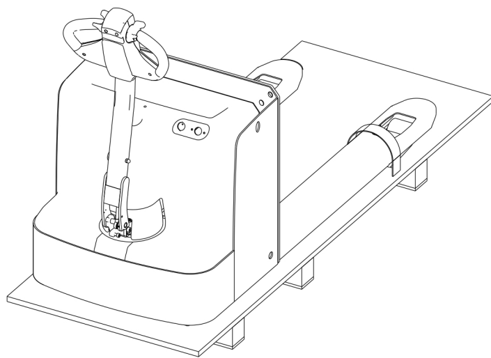
图 7 固定点
