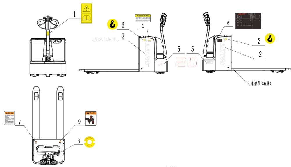
图 4 标贴描述
