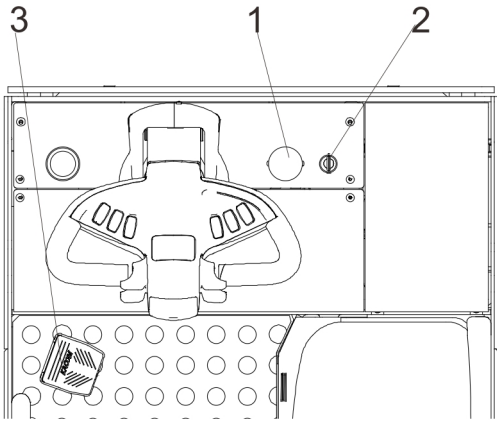
图 8 操作控制台
