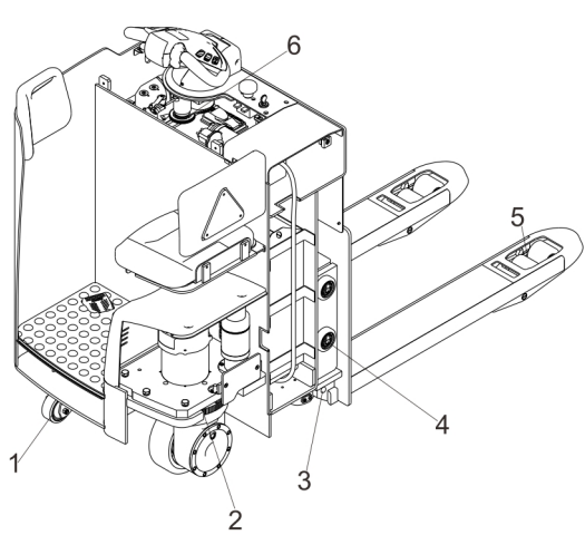
图 24 润滑点
