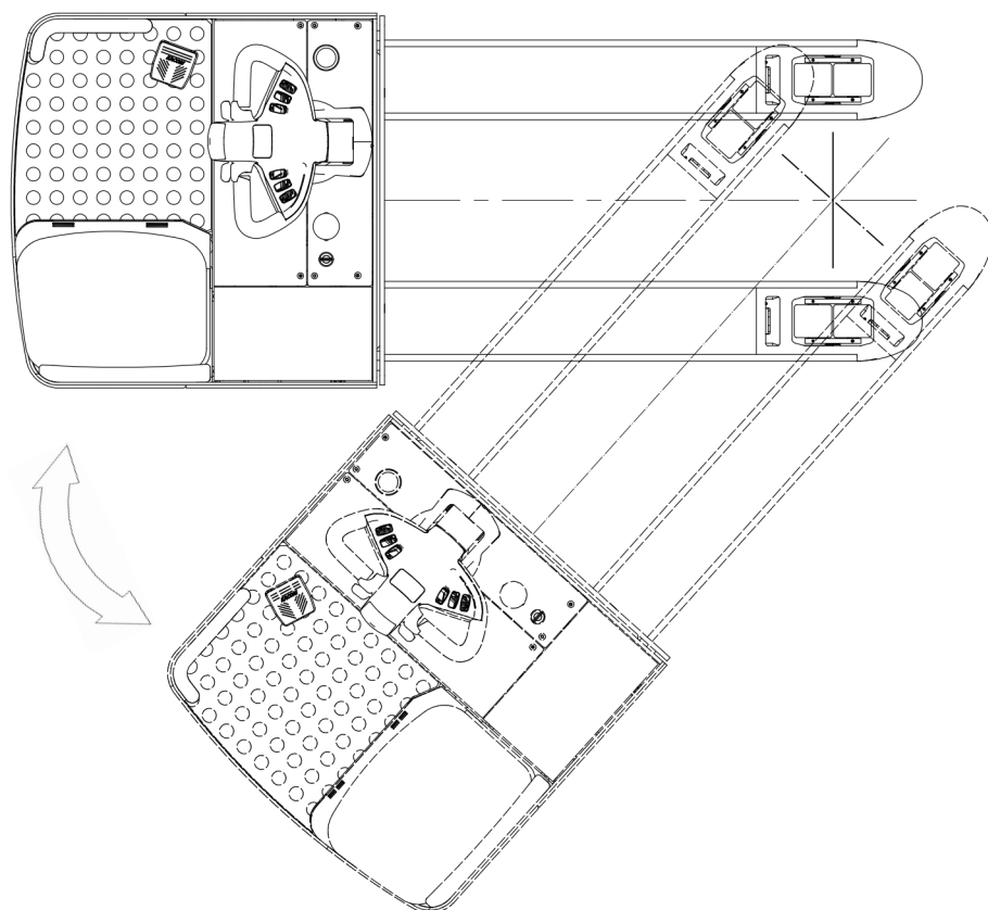
图 12 转向示意图
