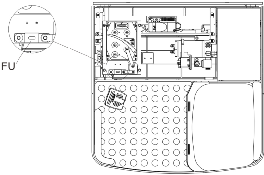
图 25 保险丝位置
