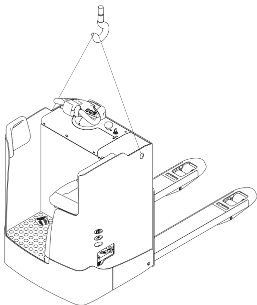
图 6 起吊
