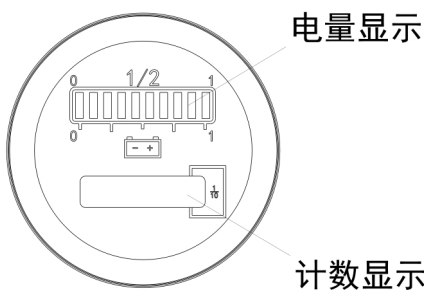
图 25 圆形电量表
