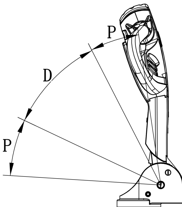
图 14 操纵杆角度
