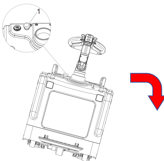
图 20 车辆倾覆
