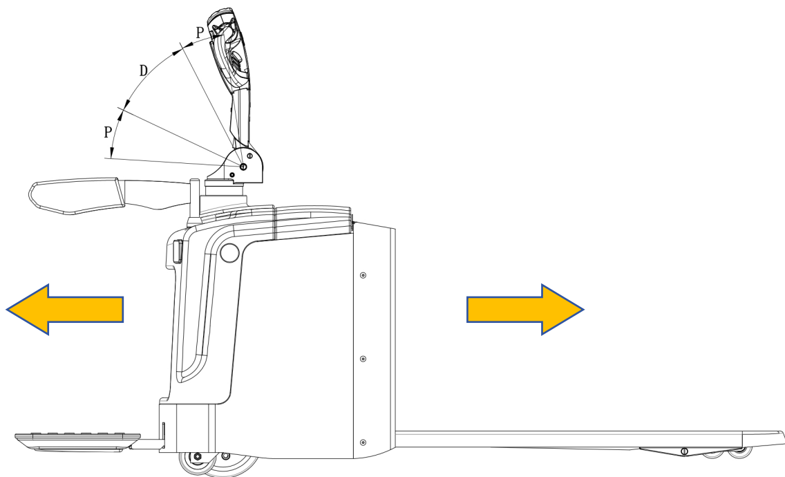
图 11 行驶示意图
