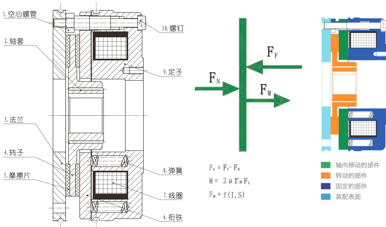
图 15 制动原理图
