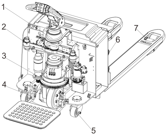
图 26 润滑点
