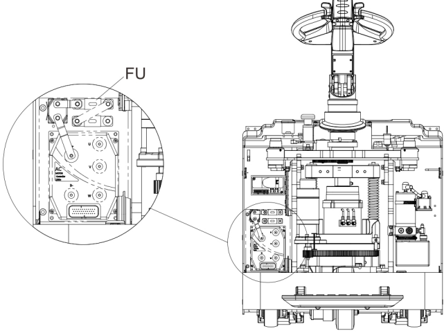
图 27 保险丝位置
