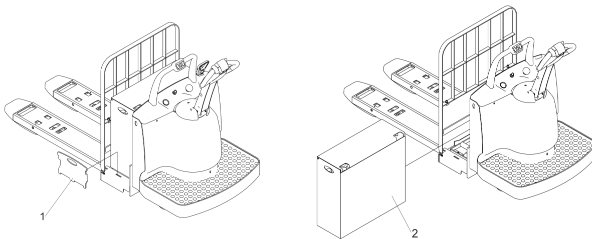
图 21 电池更换示意图
