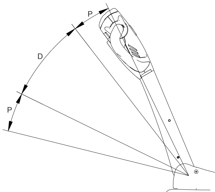
图 14 操纵杆角度
