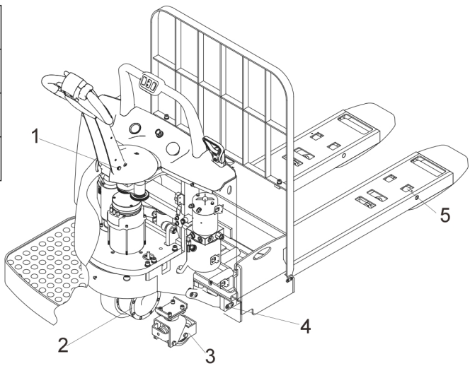
图 25 润滑点
