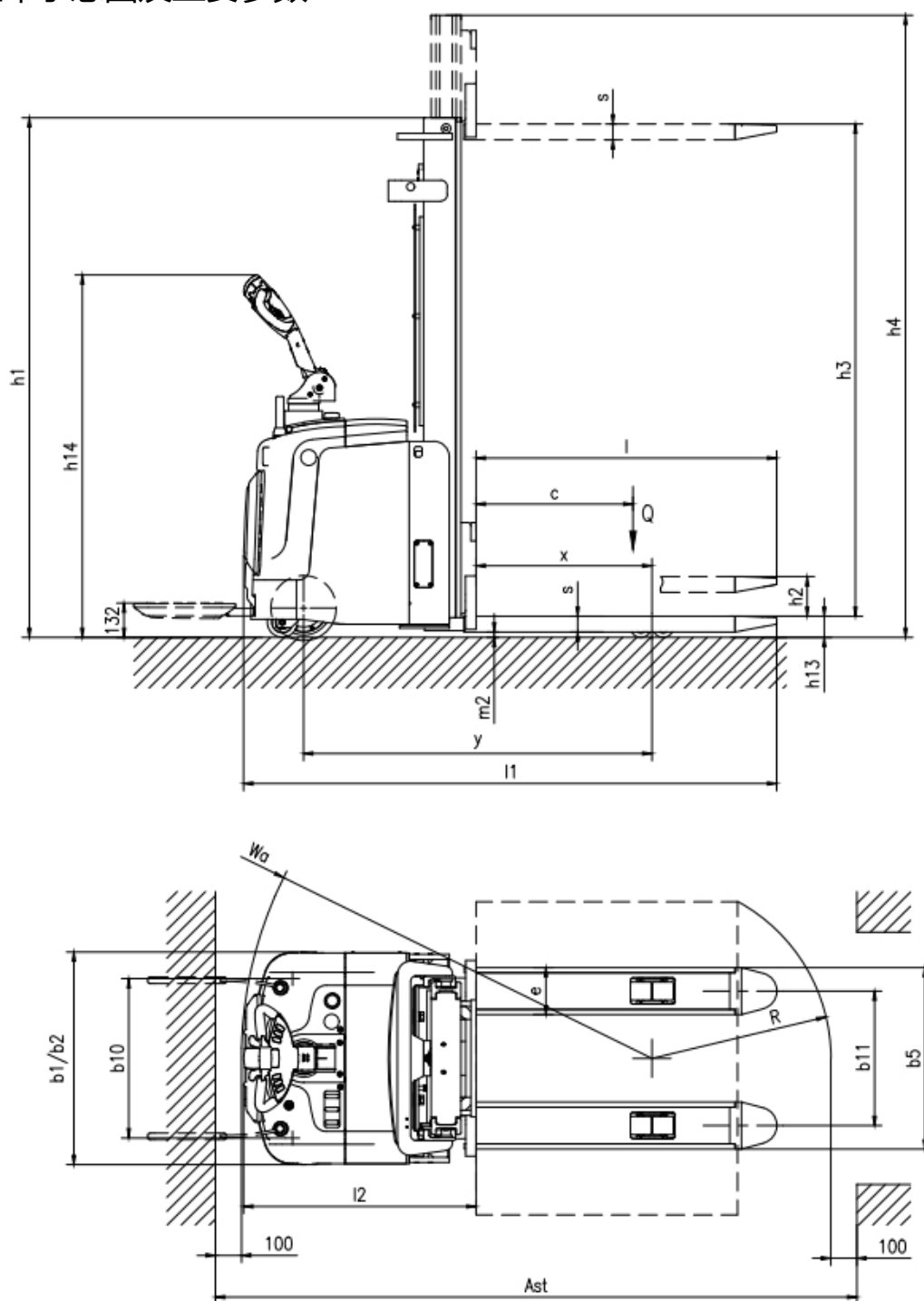
图 3 技术参数图
