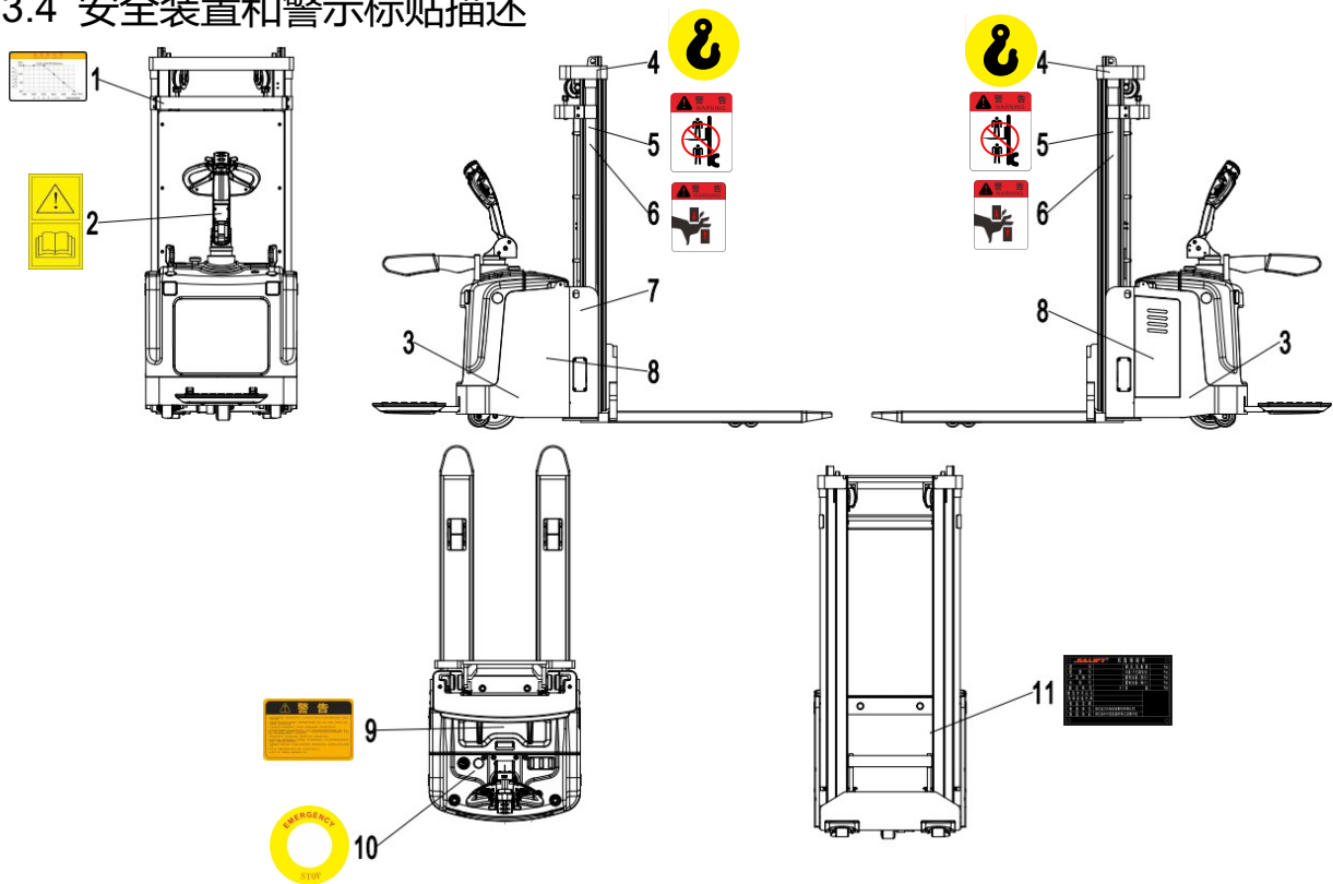
图 4 标贴描述
