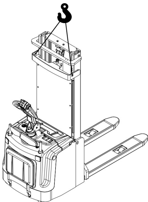
图 7 起吊
