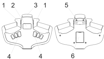
图 12 操作手柄——刷卡器（基础款）
