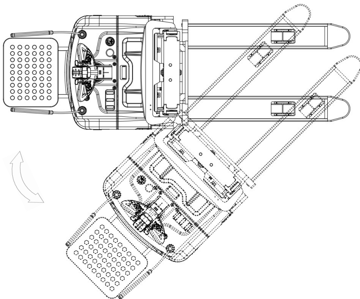
图 16 转弯轨迹
