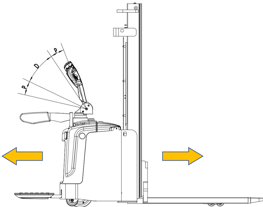
图 14 行驶
