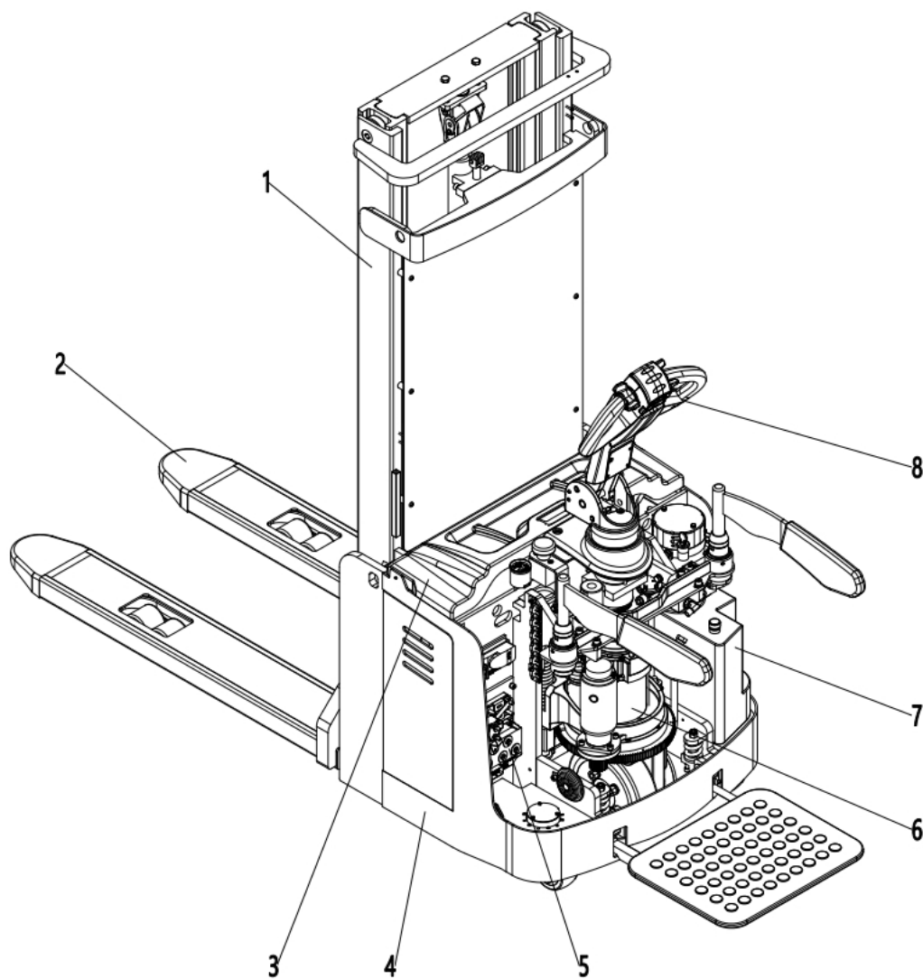
图 2 主体分类
