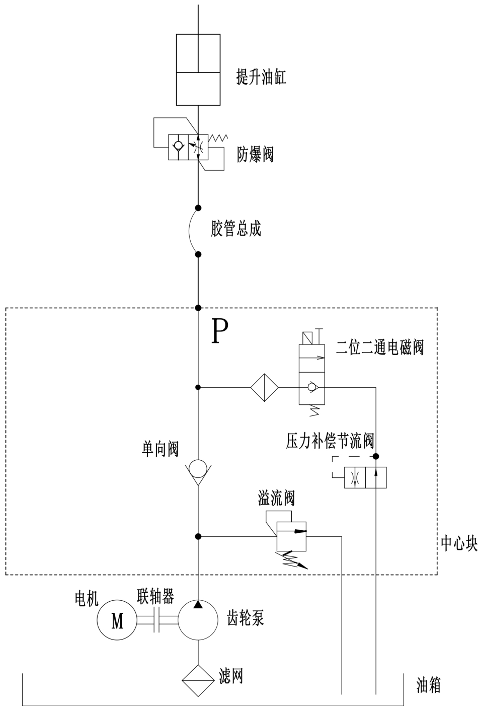
图 40 液压原理图 (单油缸)
