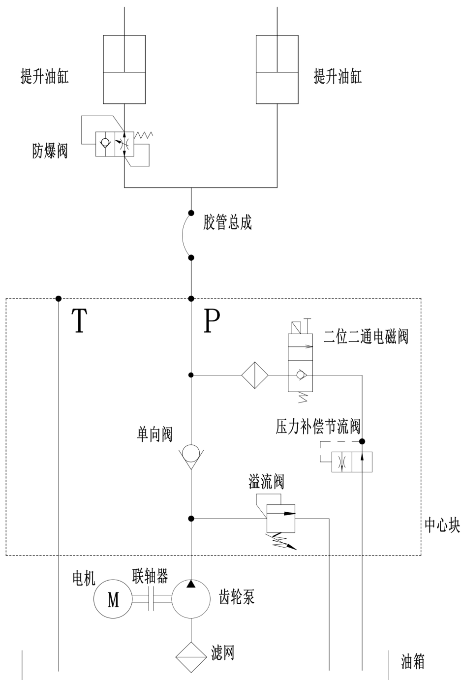
图 41 液压原理图（双油缸）
