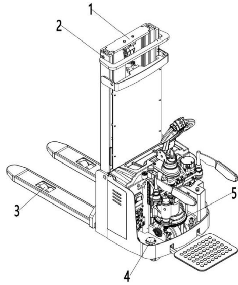
图 31 润滑点
