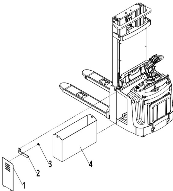
图 25 电池更换
