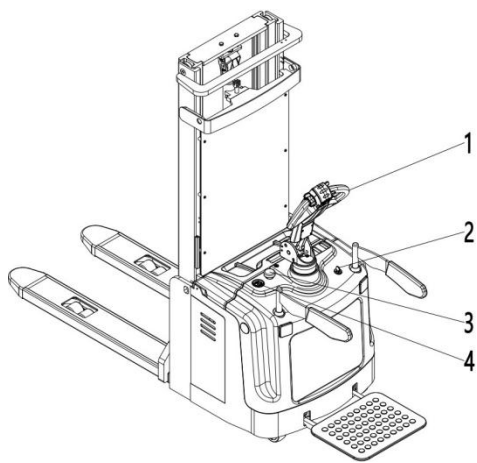
图 9 车辆操作机构
