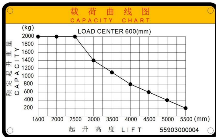
图 6 载荷曲线示意图
