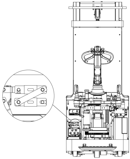
图 32 保险丝位置
