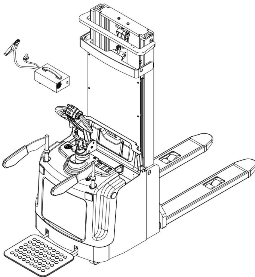
图 26 充电
